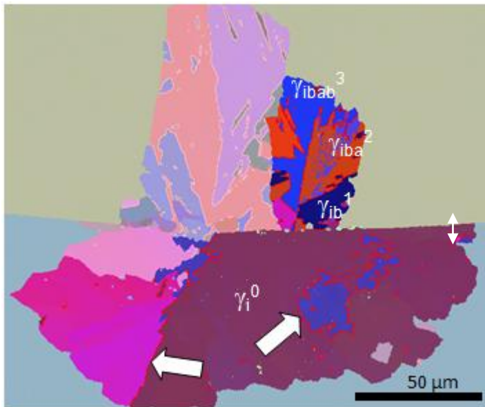
Figure 3. 8:- Carte EBSD représentée en code couleurs d'angles d'Euler, qui fait ressortir le chemin de maillage qui peut être utilisé pour remonter au germe à partir de la variante \gamma finale qui s'est formée. La flèche blanche à deux têtes montre comment la variante de maillage se retransforme à l'intérieur de son grain parent \alpha .
