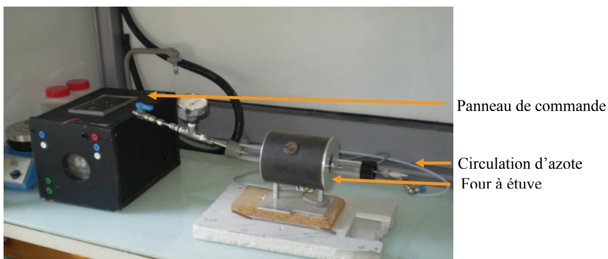
Fig. 53 Four à étuve
