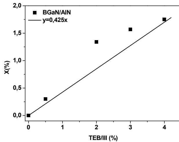
Fig. 63 Le coefficient d'incorporation du bore en phase solide pour la croissance du BGaN sur AlN.
