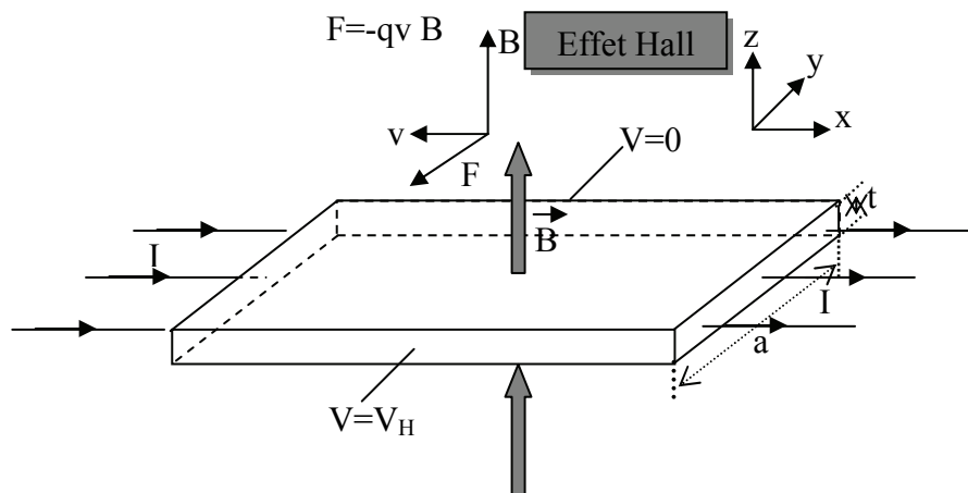
Fig. 16 Effet Hall
