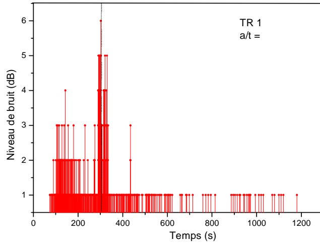
Figure 32 : Détection de point d'amorçage par émission acoustique (TR, a/t de 40%).
