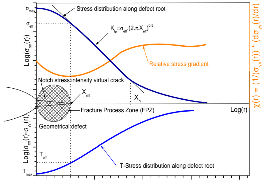
Figure 23 : Détermination du Facteur d'Intensité de Contraintes d'entaille et de la contrainte effective T_{eff} à la pointe de l'entaille, par l'application de la deuxième méthode.
