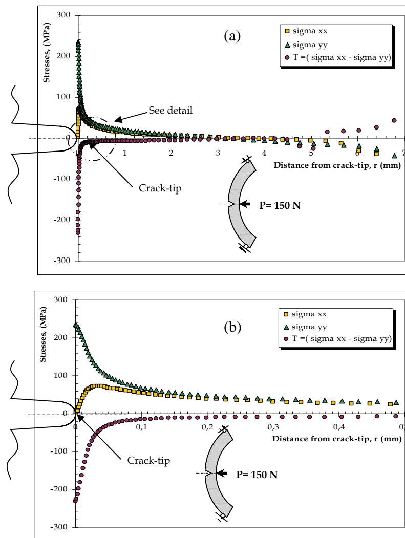
Figure 9 : (a) Exemples d'évolution des contraintes le long du ligament, pour un rapport d'épaisseur de 20% ( a/t = 0.2 , P = 150 \text{ N} ). (b) Détail de (a) [59].
