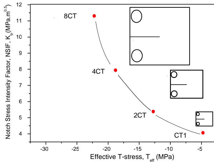
Figure 91 : Evolution de la courbe K_p - T_{eff} en fonction de l'évolution d'échelle de éprouvettes CT.
