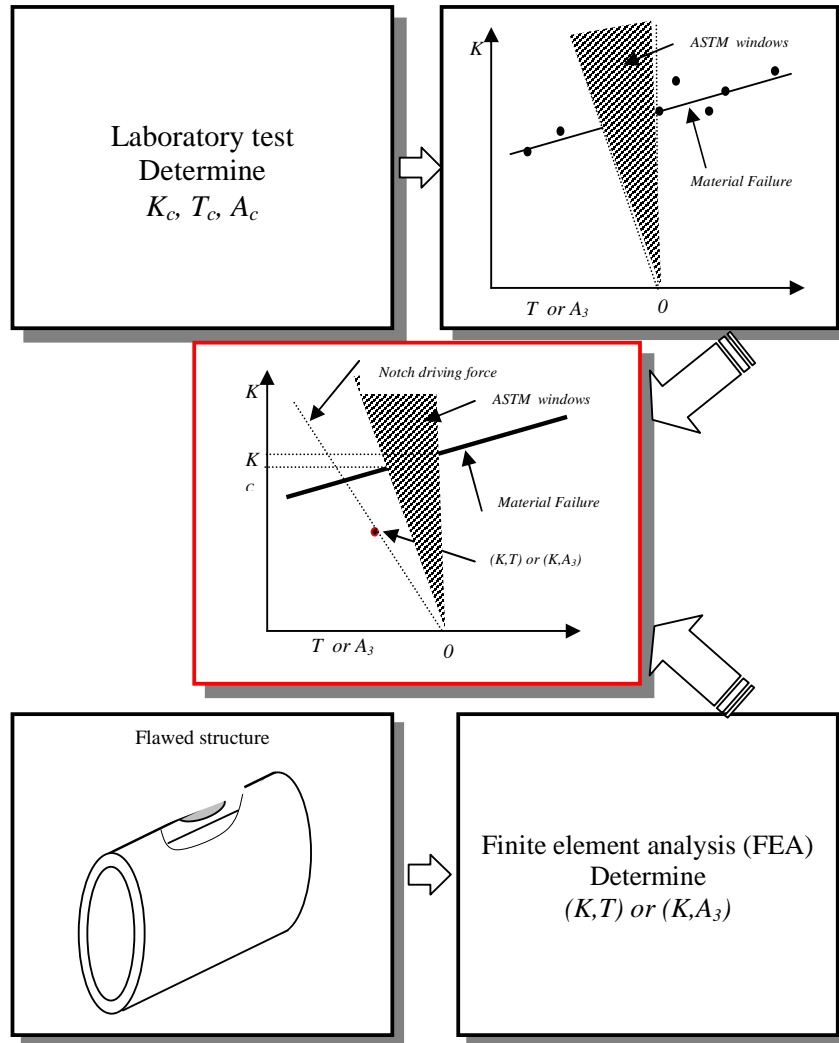
Figure 59 : Proposition d'une procédure d'évaluation.
