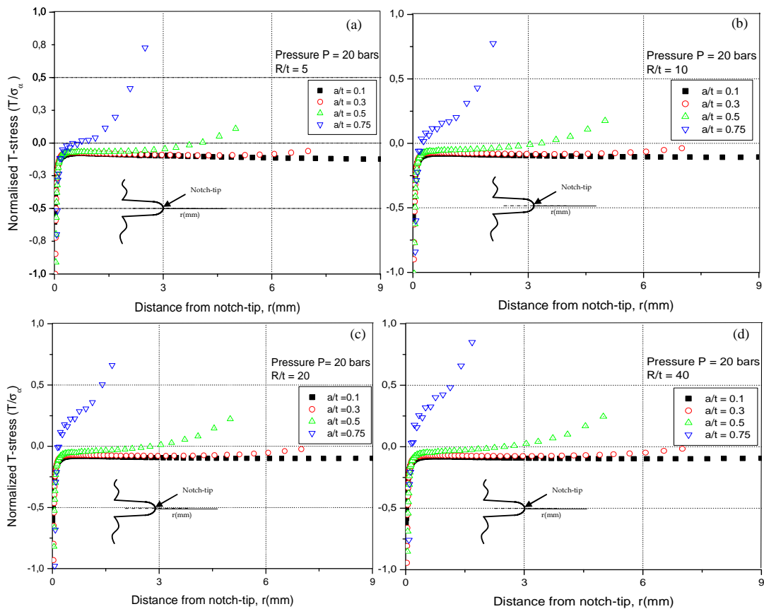
Figure 14 : Evolution de la contrainte T ( T/\sigma_\alpha ), pour une entaille longitudinale de surface et une pression de 20 bars, pour les cas : (a) R/t = 5 . (b) R/t = 10 . (c) R/t = 20 et (d) R/t = 40
