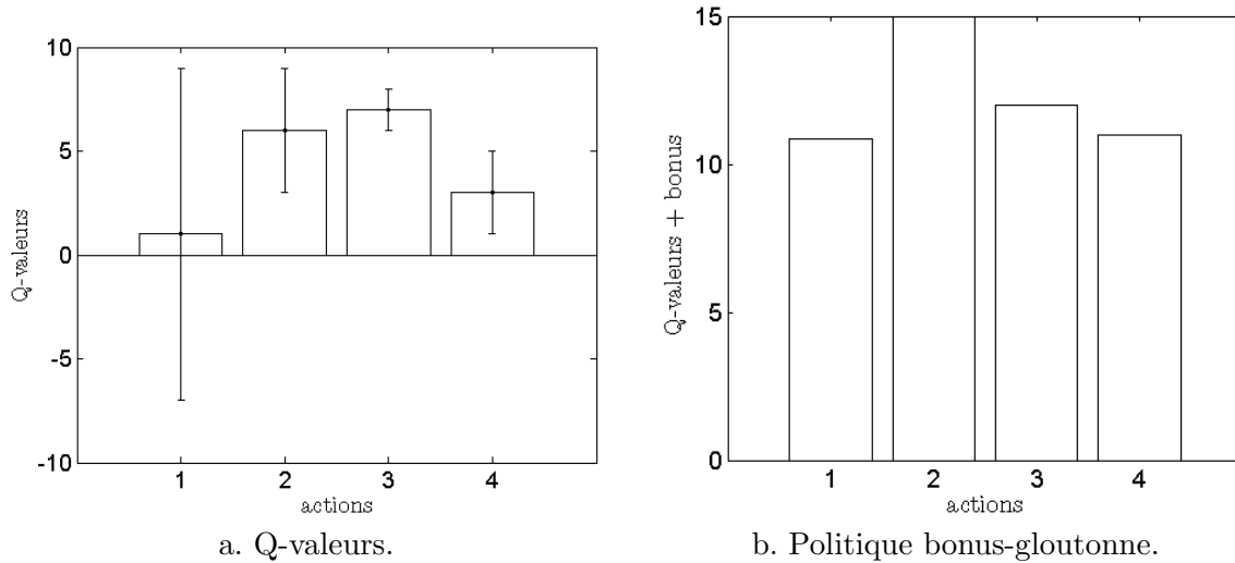
FIG. 6.7 – Politique bonus-gloutonne illustrée.
