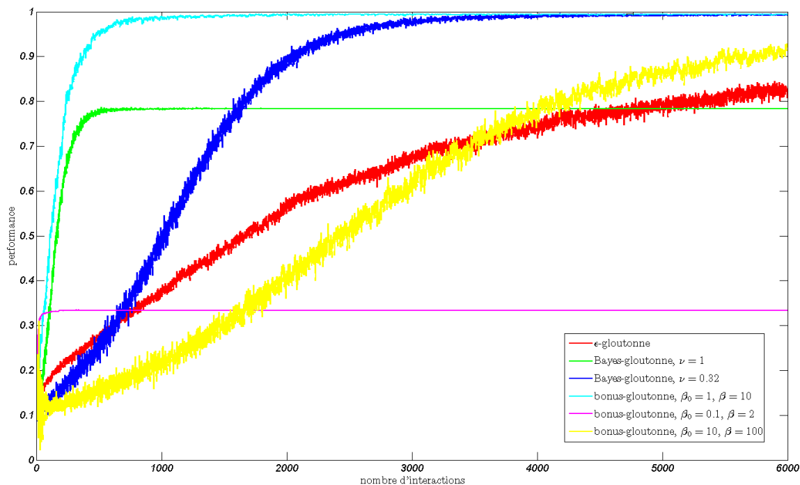
FIG. 6.13 – Bandits, influence des paramètres libres.
