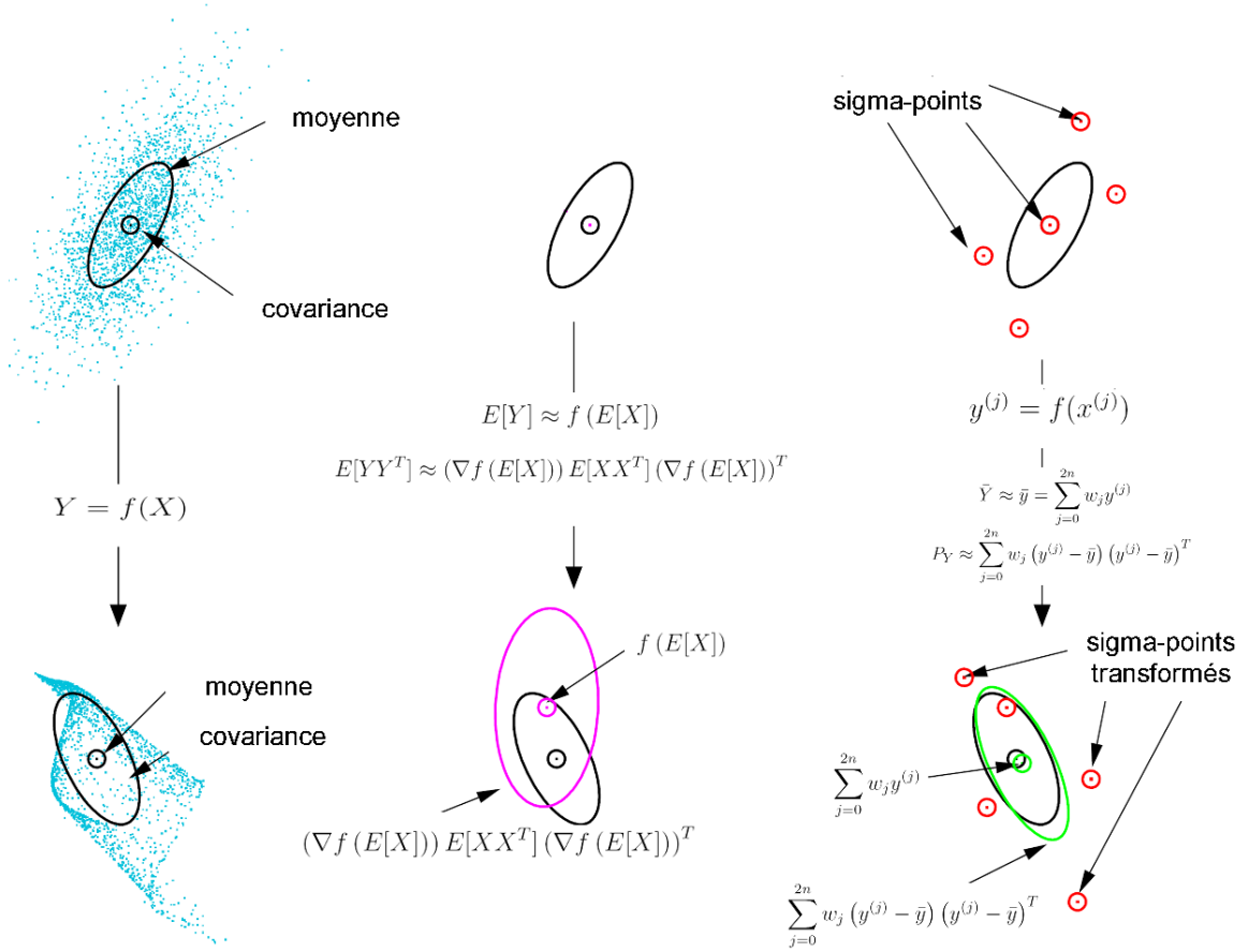
FIG. 3.1 – Illustration de la transformation non-parfumée.
