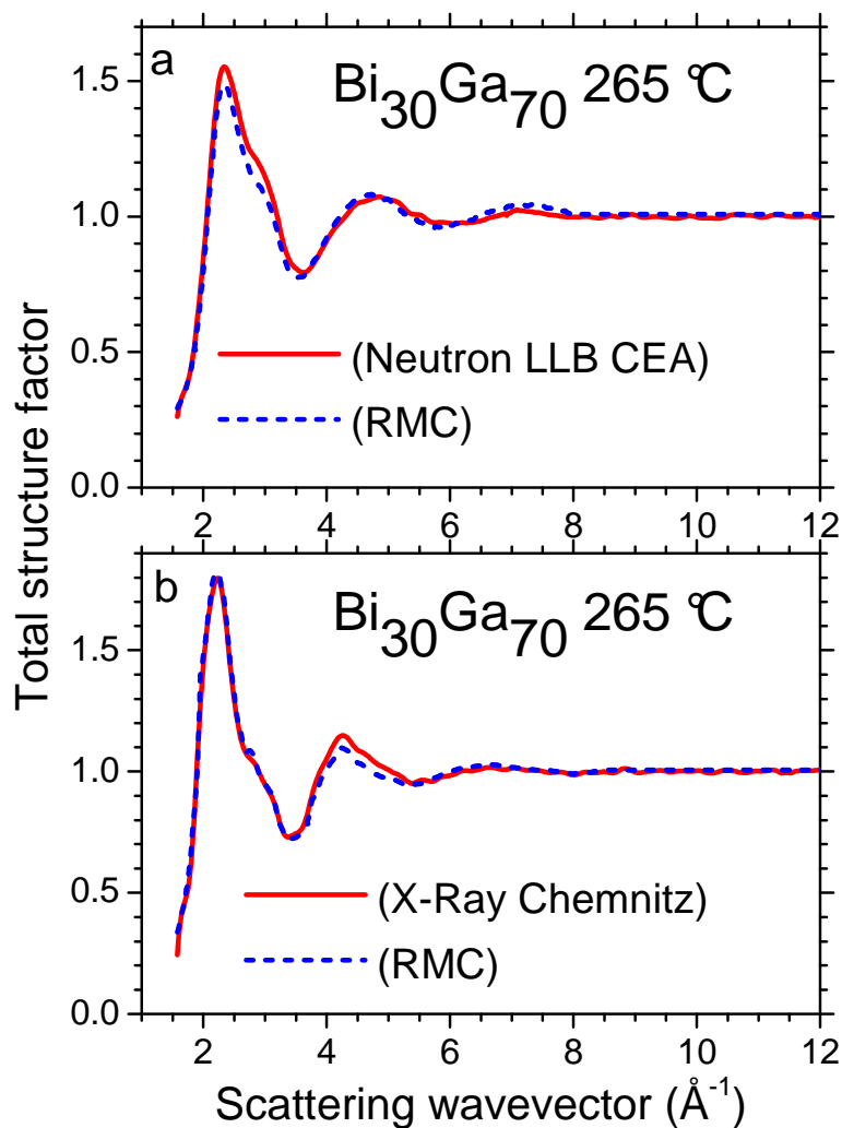
Figure 4.16 : Facteurs de structure totaux de Faber-Ziman S'(q) expérimentaux et modélisés par le code RMC de l'alliage liquide \text{Bi}_{30}\text{Ga}_{70} pour les neutrons (graphie du haut) pour les rayons X (graphie du bas).
