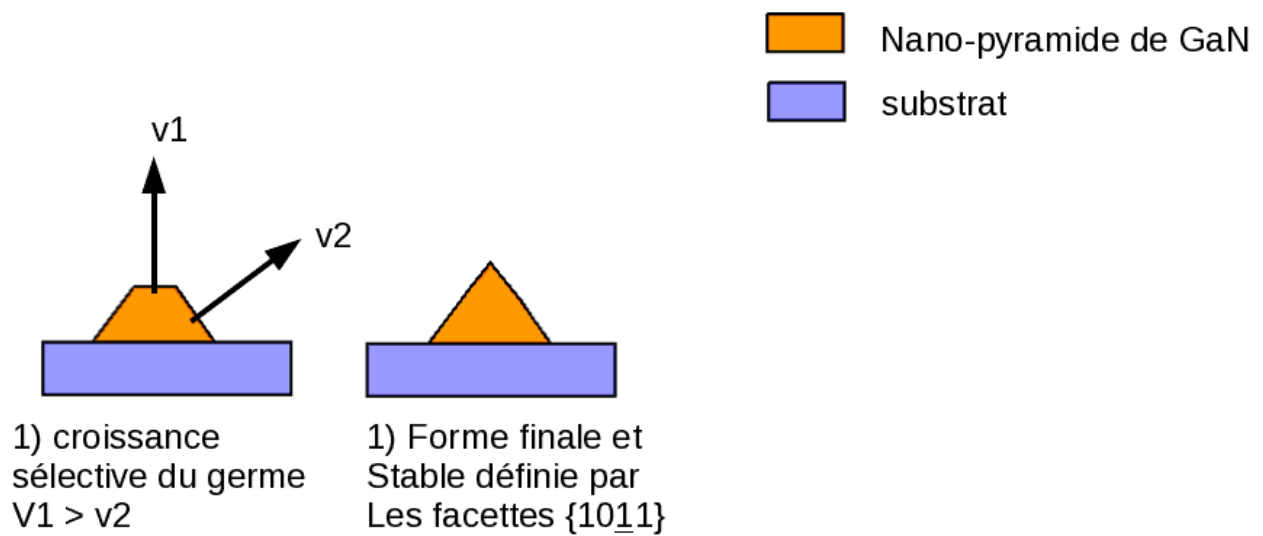
Fig.2.26 – Vitesses de croissance des différents plans cristallographiques des nano-pyramides de GaN épitaxiées sélectivement.
