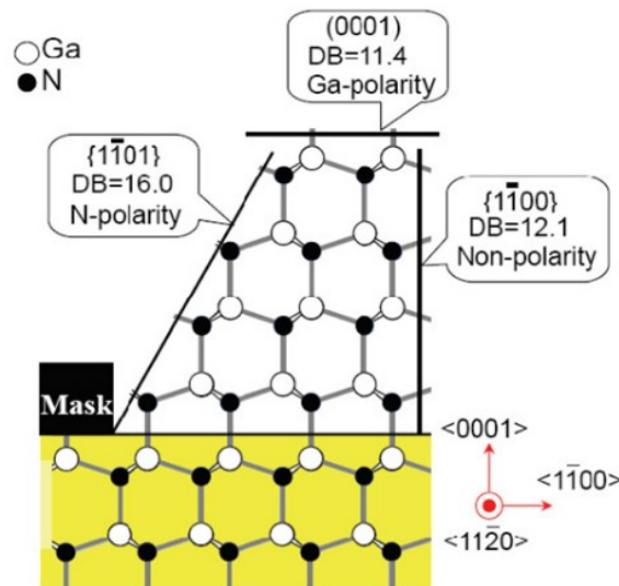
Fig. 1.12 - Densité de liaisons pendantes par unité de surface (en nm -2 ) pour différents plans cristallographiques de GaN [Hide07]
