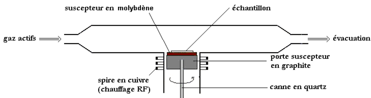
Fig. 2.2 - Schéma du réacteur en T utilisé au laboratoire
