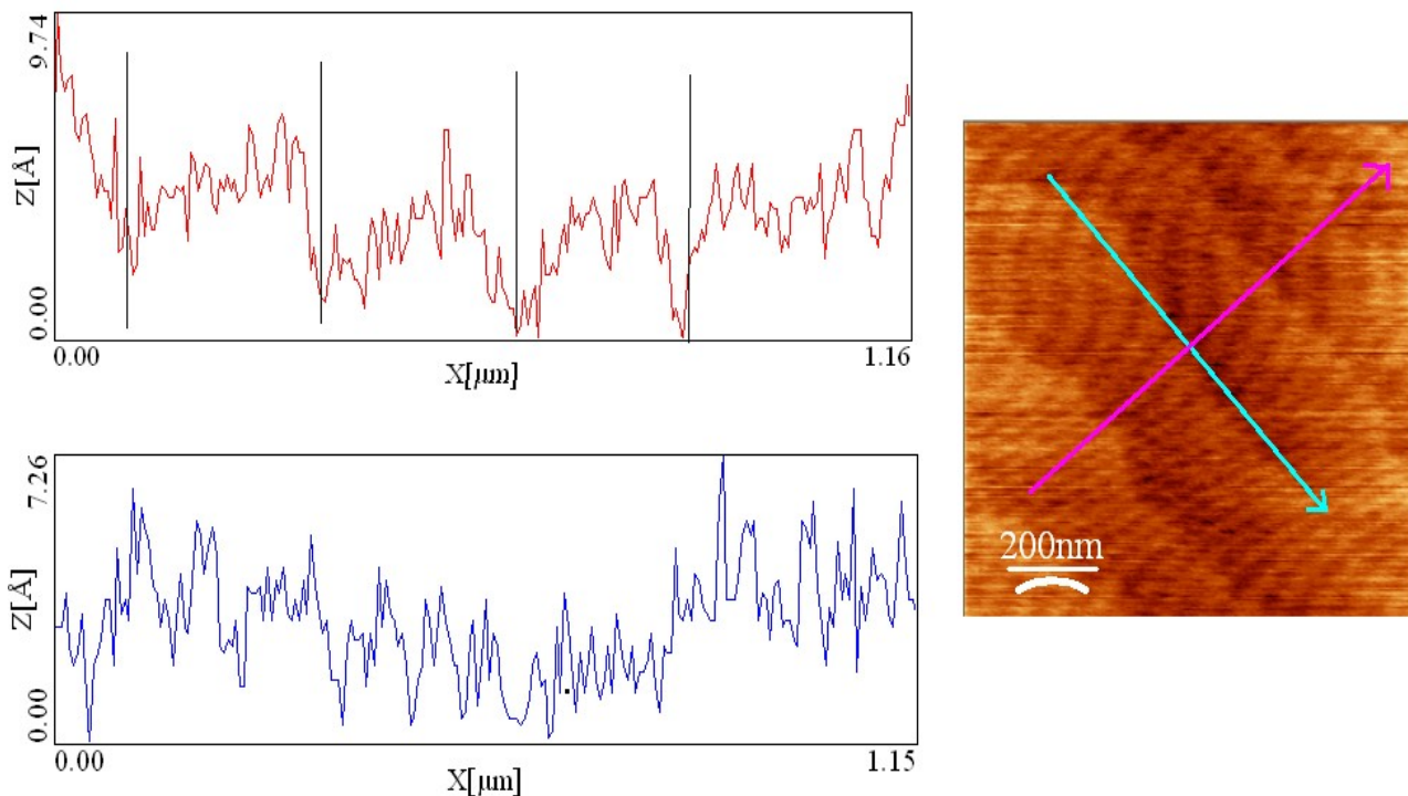
Fig.3.5 - Profils AFM mesurés sur un substrat de SiC. Le profil rouge provient de la mesure effectuée le long de la flèche mauve (// axe [11\bar{2}0] ) sur l'image AFM de droite, et le profil bleu provient de la la mesure effectuée le long de la flèche bleue (// à l'axe [11\bar{0}0] ). Les marches atomiques de hauteur moyenne égale à 2,5 \text{ \AA} sont repérables.
