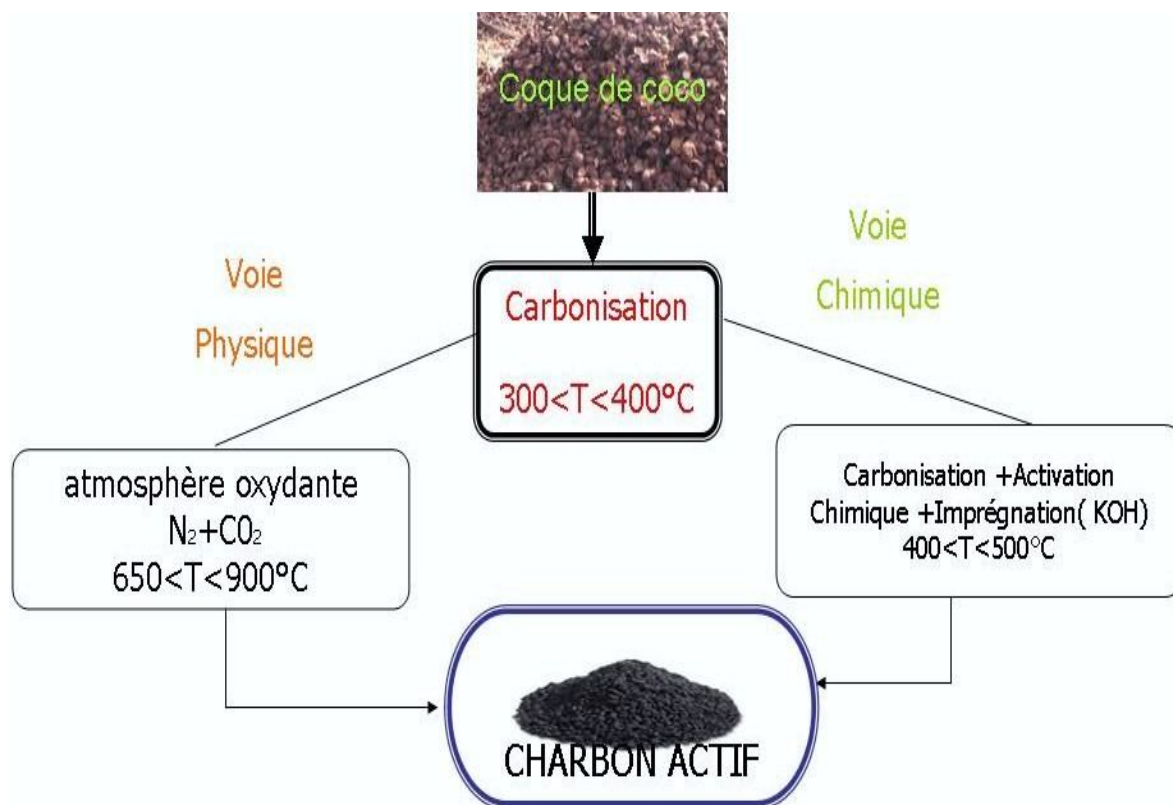
Figure II. 7 : Schéma synoptique des différentes voies d'activation (de la coque de coco au charbon actif) : la voie chimique utilise des agents oxydants chimiques ( \text{NaOH} , \text{H}_3\text{PO}_4 , \text{ZnCl}_2 ) après la pyrolyse. La voie physique consiste en une seule étape (pyrolyse), avant l'activation.
