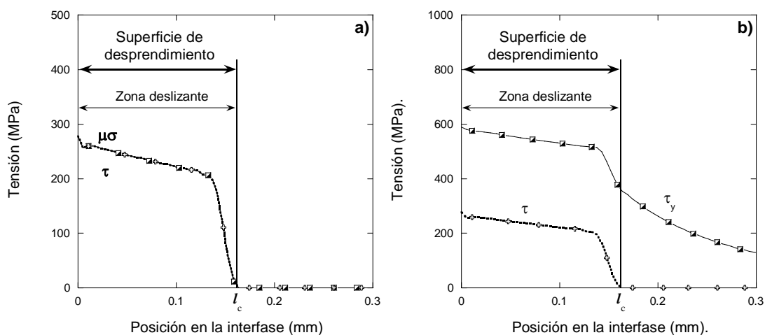
Figura 3.4: Comparación de la tensión de fricción \tau con: a) el producto \mu \cdot \sigma , b) la tensión límite del material de cizalladura \tau_y = \sigma_{eq} / \sqrt{3} . Velocidad de corte V = 8 \text{ m/s} , coeficiente de fricción implementado \mu = 0.2 .
