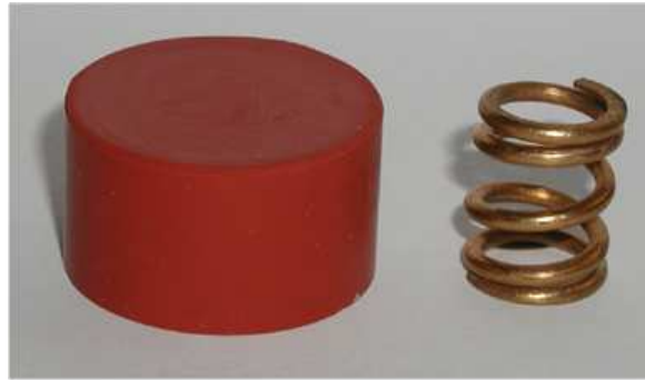
FIG. 5.1: Constituants du plot composite : cylindre en silicone et ressort en CuAlBe, d'après [Tahiri et al., 2004]
