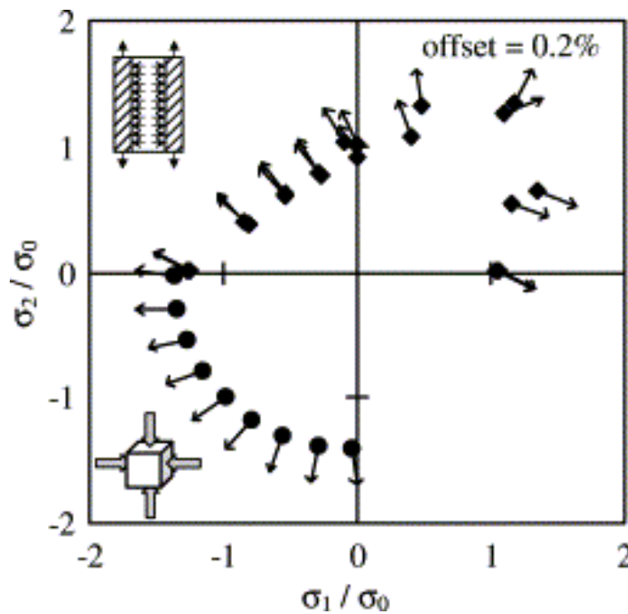
FIG. 1.18: Surface de charge de transformation expérimentale (alliage CuAlBe), d'après [L'excellent et al., 2002].
