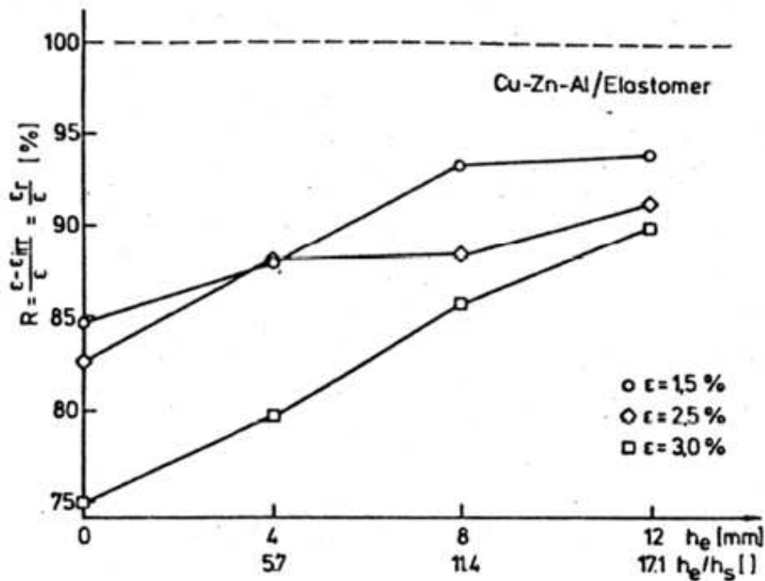
FIG. 1.20: Degré de déformation réversible lors d'une reprise de forme en fonction de la fraction d'épaisseur élastomère/AMF. L'ajout d'une couche épaisse d'élastomère facilite l'effet mémoire de forme, d'après [Thumann et al., 1986].
