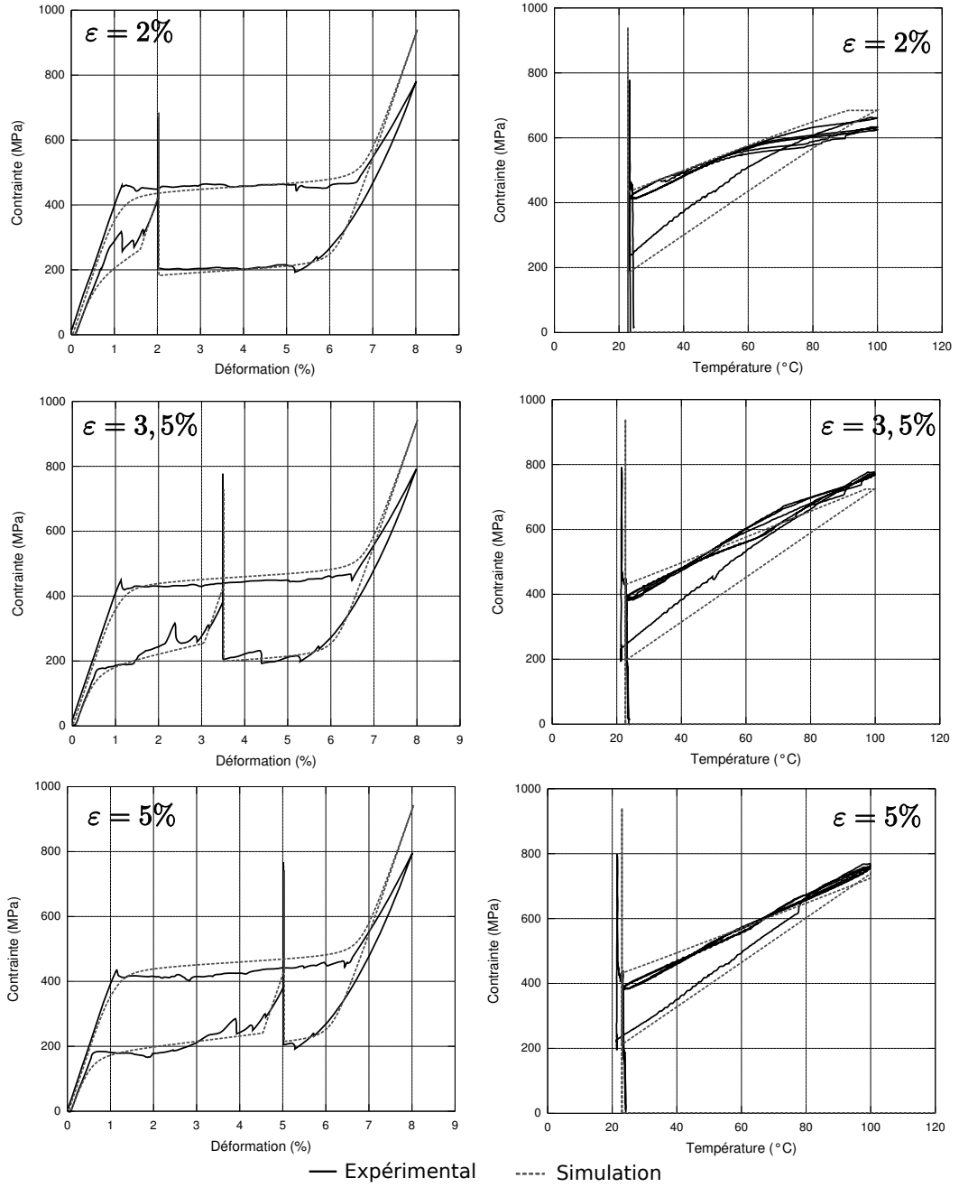
FIG. 4.29: Cycles de retours contraints - plateau inférieur
