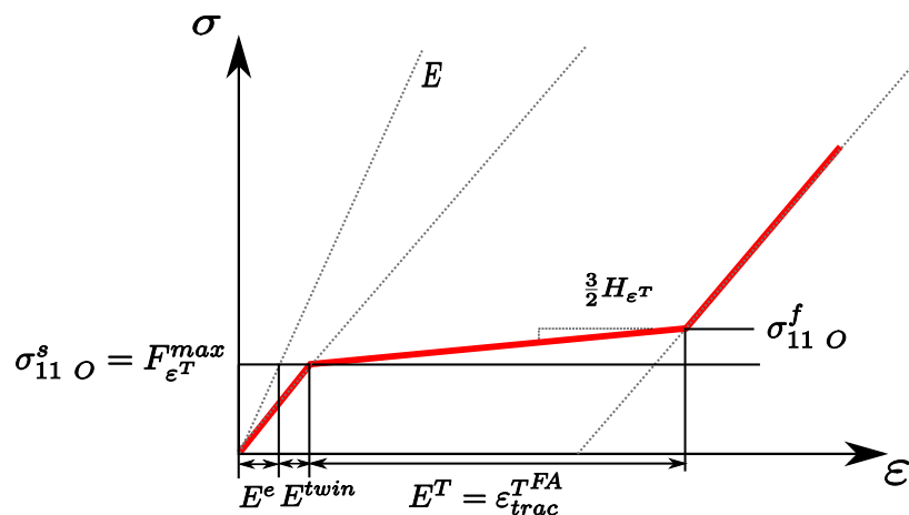
FIG. 4.2: Identification des paramètres F_{\epsilon}^{Tmax} , H_{\epsilon}^T et \epsilon_{trac}^{TFA} à partir d'une courbe de comportement de martensite initialement autoaccommodée, en traction uniaxiale. Pour la clarté du schéma, l'influence de la déformation élastique sur l'identification de la déformation maximale de la martensite autoaccommodée est négligée
