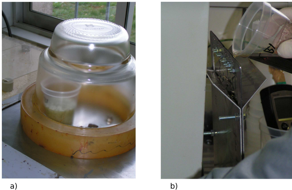
FIG. 5.10: a) procédé de dégazage du mélange. b) Opération de coulage
