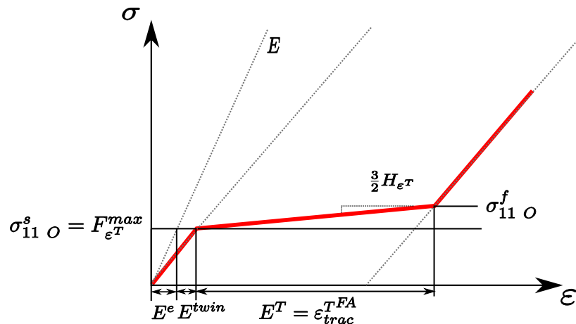
FIG. 4.2: Identification des paramètres F_{\epsilon T}^{max} , H_{\epsilon T} et \epsilon_{trac}^{TFA} à partir d'une courbe de comportement de martensite initialement autoaccommodée, en traction uniaxiale. Pour la clarté du schéma, l'influence de la déformation élastique sur l'identification de la déformation maximale de la martensite autoaccommodée est négligée
