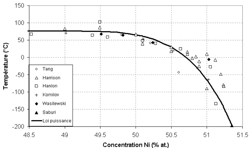
FIG. 6.4: Variation de la température M_s en fonction de la concentration de nickel. Comparaison entre la loi puissance et les résultats expérimentaux (pour les références des points expérimentaux, voir [Tang et al., 1999])
