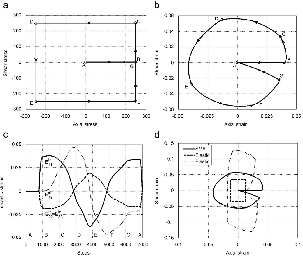
FIG. 2.1: a) Exemple de chargement proportionnel "carré" dans l'espace des contraintes axiales et de cisaillement b) évolution des déformations axiale et de cisaillement. c) Evolution dans le temps de la partition des déformations. d) Comparaison avec des lois élastiques et élastoplastiques (d'après [Panico et Brinson, 2007]).
