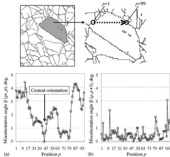
FIG. 4.6 – Représentation de la désorientation intragranulaire le long d'une ligne (en pointillés), dans la direction transverse, sur un grain pour une déformation de l'éprouvette de 14,4%. La désorientation est représentée par rapport à l'orientation cristallographique au centre du grain (a) puis par rapport au point adjacent (b) [KWT05]
