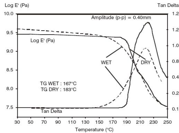
Comparaison sèche/mouillé (14 jours dans l'eau à 70°C)
