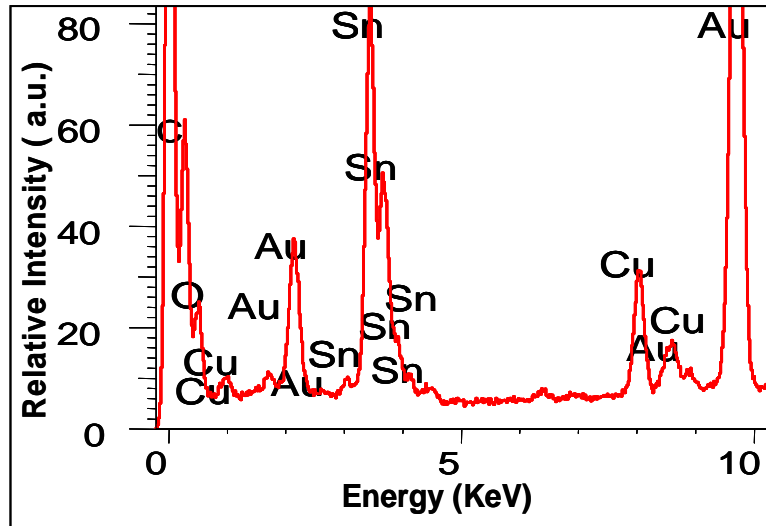
Figure IV-7: Spectres par EDX de couches minces de \text{SnO}_2 dopé 4 at.% Cu déposées à 400\text{ }^\circ\text{C} (2ml/h pendant 1h) et recuit dans l'air à 550\text{ }^\circ\text{C} pour 2h.
