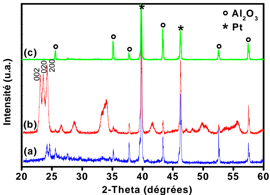
Figure VII-6: Spectres de DRX des couches minces de (a) WO_3 déposées à 350^\circ C ( 1ml/h pendant 1h ) et (b) recuites dans l'air à 500^\circ C pendant 2h , (c) substrat.
