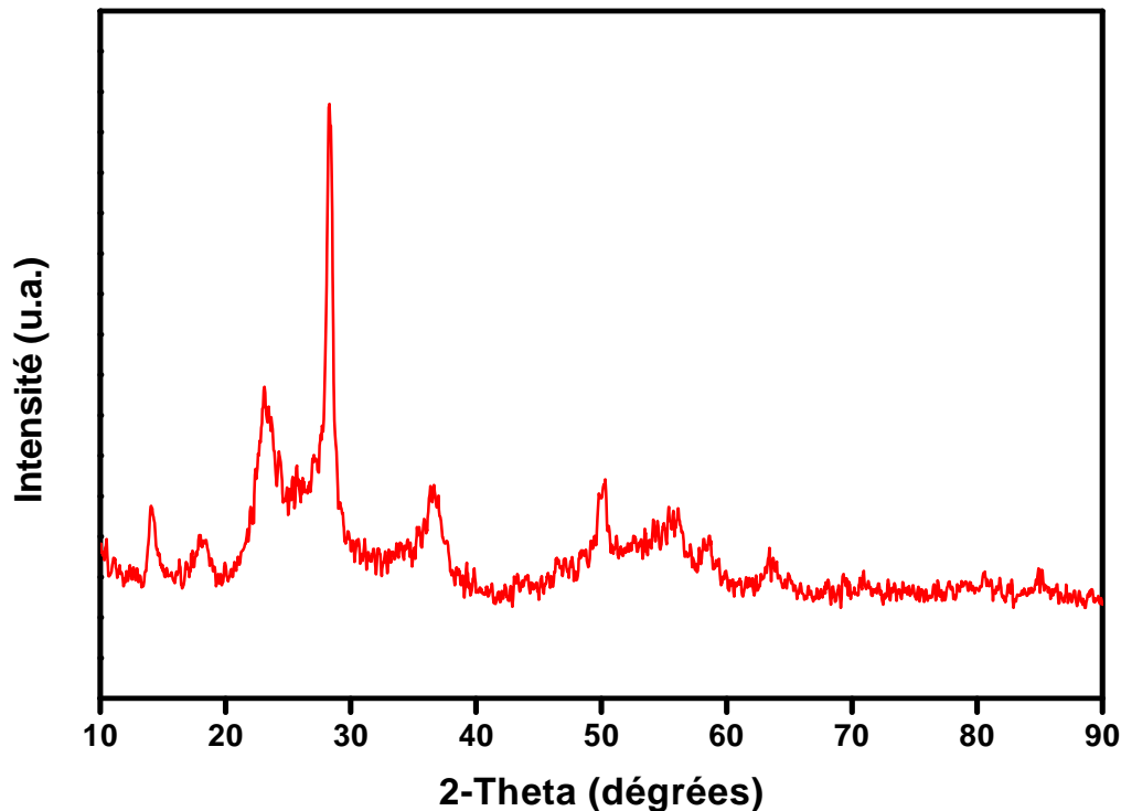
Figure VII-3: Spectres par DRX de poudre de WO_3 \cdot 1/3H_2O obtenue en séchant la solution de PTA à 60°C.
