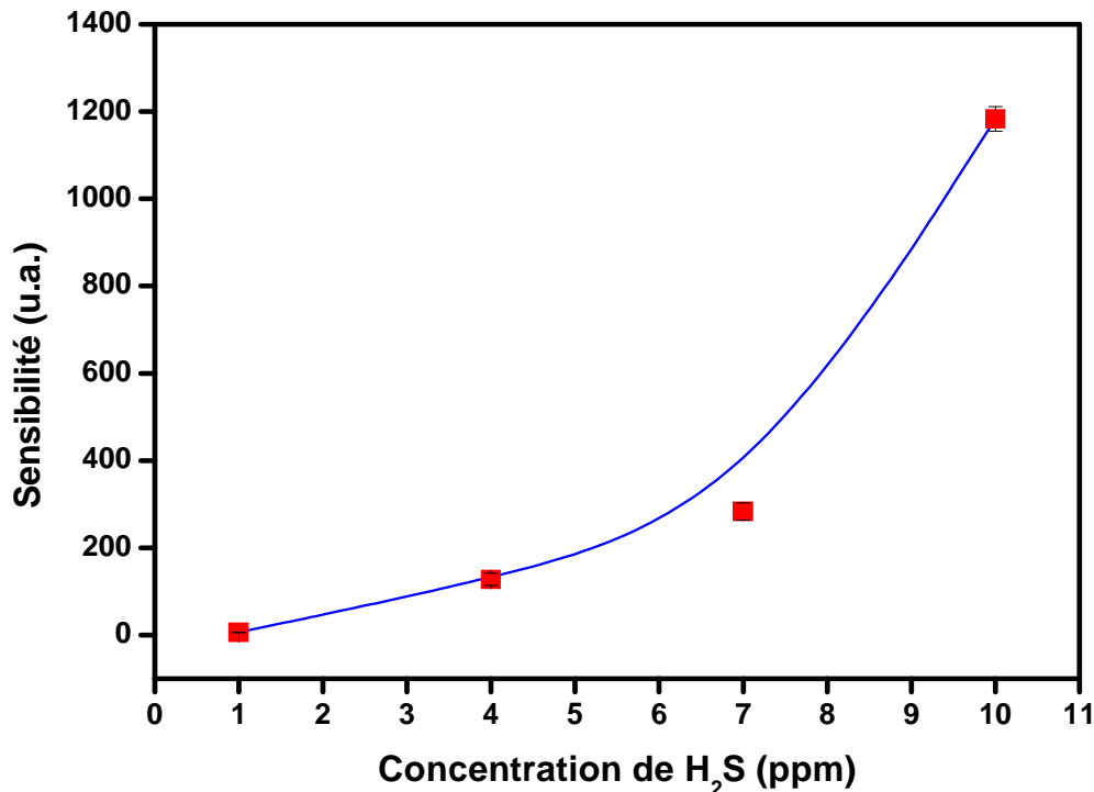
Figure VII-10: La sensibilité de WO 3 en fonction de la concentration de H 2 S pour une température de fonctionnement de 200°C.
