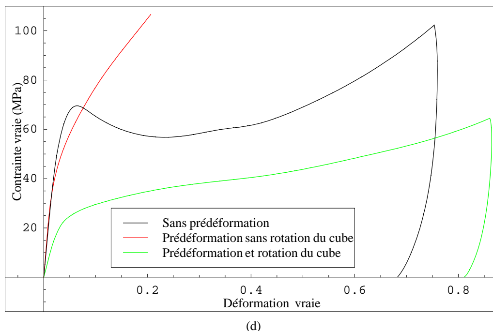
Figure 2.23. Comparaison des seconds chargements avec et sans rotation du cube : (a) à 13% de prédeformation, (b) à 31% de prédeformation, (c) à 52% de prédeformation et (d) à 75% de prédeformation
