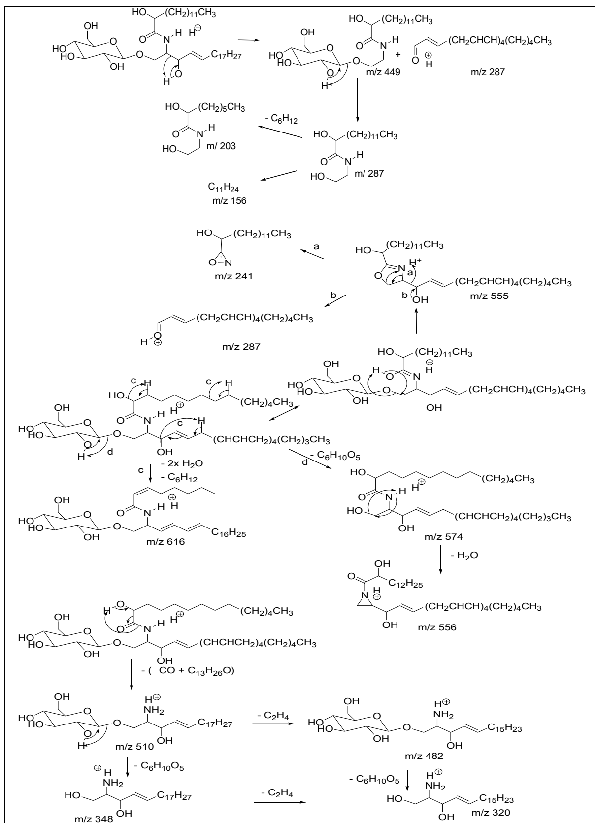
Schéma 15: Quelques ions fragments issus de la msms de l'ion à m/z 736
