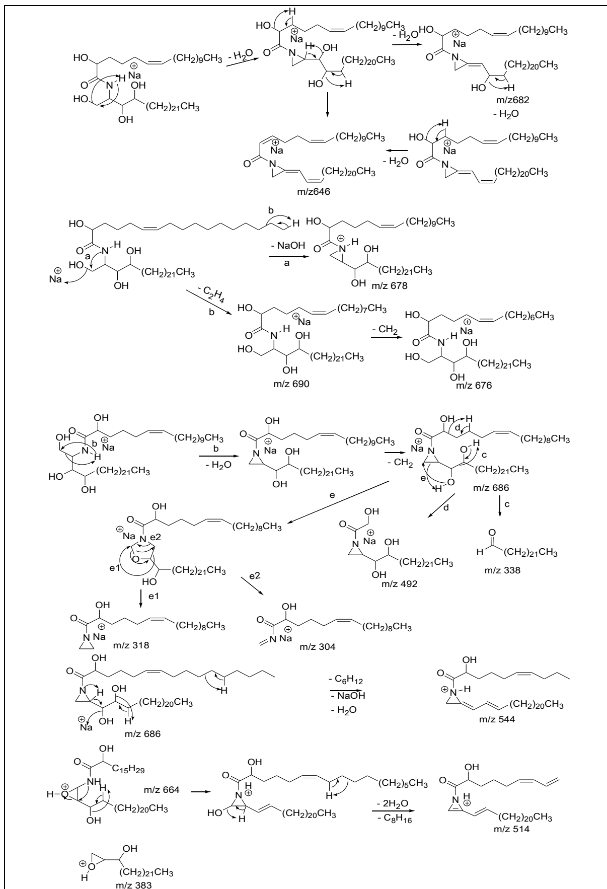
Schéma 11: Quelques ions fragments de composé LP10.
