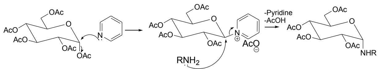
Schéma 36: mécanisme de synthèse de glucosylation.
