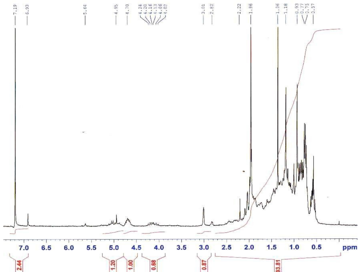
Figure 78: Spectre de RMN ^1\text{H} de 3- O -acétyl-5 \beta ,6 \beta -époxytigmastan-22-en-3 \beta -ol
