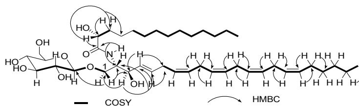
Schéma 12: Corrélations importantes HMBC et COSY de LP11.
