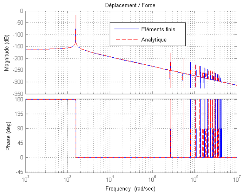
FIGURE 4.19 – M_t = 50Kg , réponse fréquentielle ( \frac{u}{F} )
