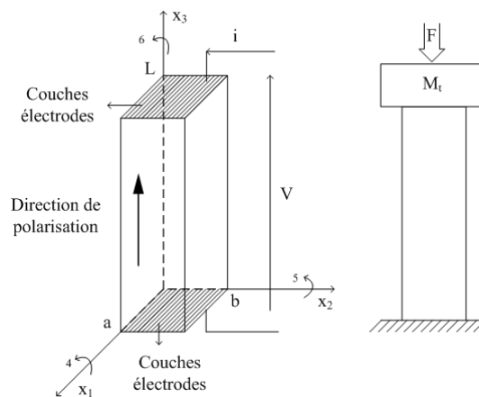
FIGURE 3.4 – Barreau piézoélectrique en mode-33
