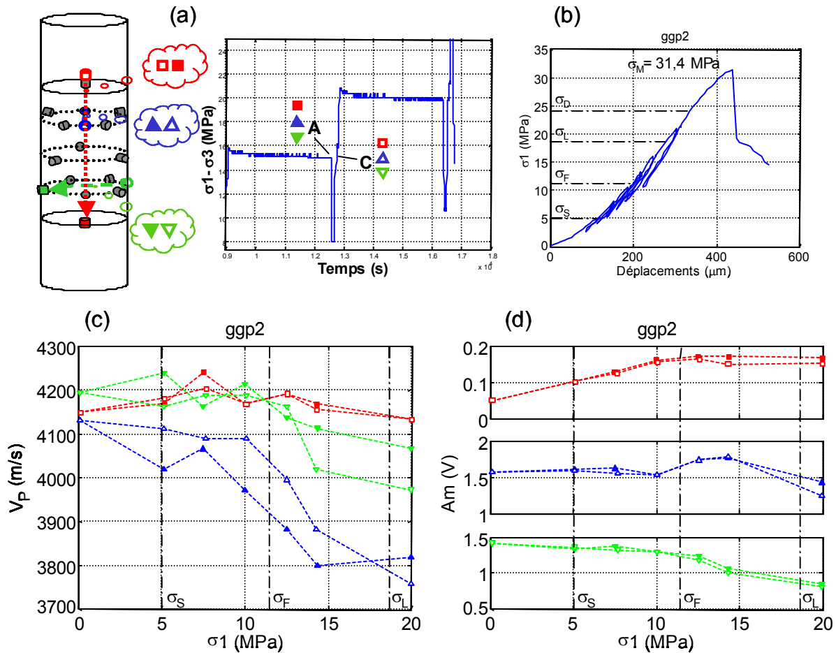
Figure 3.40 : (a) Mesures de vitesses et d'atténuation selon trois rais et signalétique utilisée, essai ggp2. (b) Rappel du comportement mécanique (courbe \sigma_1 - u ) et seuils de contrainte. (c) Evolution des vitesses de propagation des ondes P durant l'essai mécanique selon le rai axial ( \square rouges), le rai transversal haut ( \Delta bleus) et le rai transversal bas ( \nabla verts). Les motifs pleins et les motifs vides correspondent respectivement aux points A_i et C_i de mesure (avec i=1 à 6, numéro de cycle). Les seuils de contraintes sont en pointillés. (d) Evolution des amplitudes maximales selon les trois rais précédents aux points A_i et C_i en fonction de la contrainte \sigma_1 . Les seuils de contraintes sont en pointillés.
