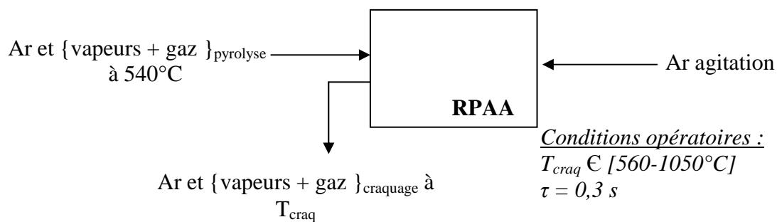
Figure A.XX.1 Principe d'une expérience de craquage
