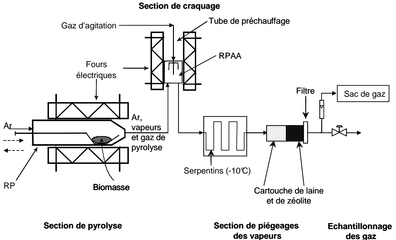
Figure III.9 Montage expérimental de craquage de vapeurs de pyrolyse de biomasse
