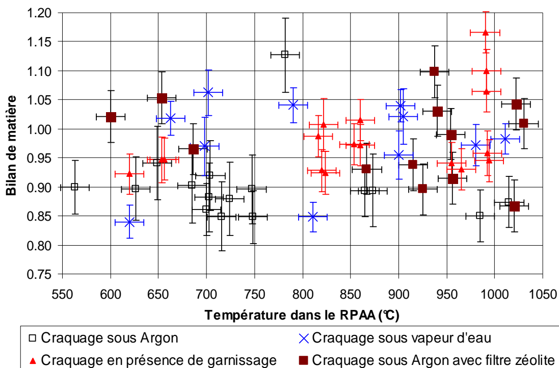
Figure IV.4 Bilans de matière en craquage de vapeurs de pyrolyse de bois sous atmosphère inerte (carrés noirs), sous vapeur d'eau (croix bleues) 50 et en faisant varier la surface de contact (triangles rouges)
