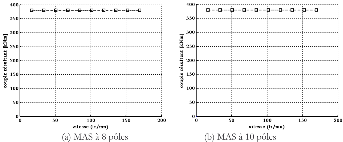
Figure 3.47 : Evolution du couple à flux constant en fonction de la vitesse
