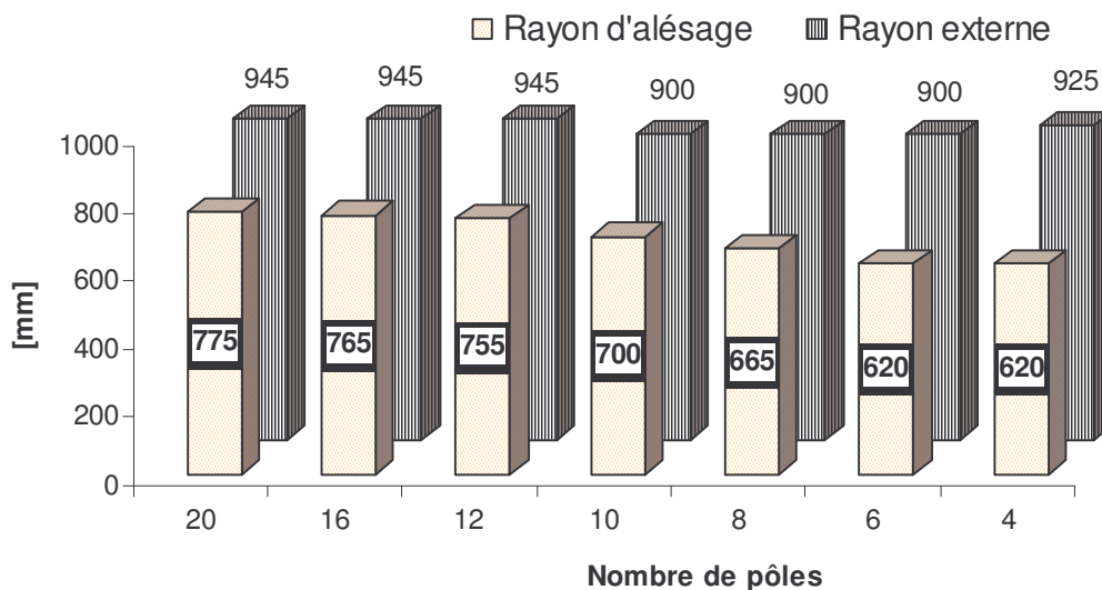
Figure 3.35 : Rayons d'alésage et externe en fonction de la polarité
