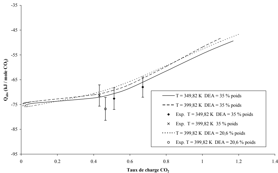
FIG. 82 Chaleurs d'absorption de CO 2 dans des solutions aqueuses de DEA. Comparaison entre courbes calculées et valeurs expérimentales
