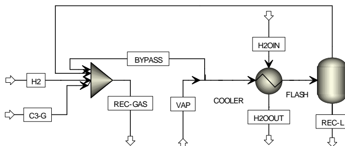
图7.3 液相釜顶冷凝回流流程
