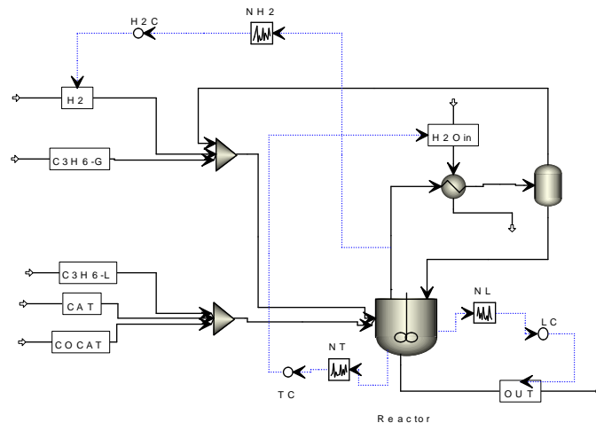
图7.29 加入测量噪声后的动态流程
