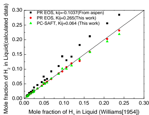
图3.11 丙烯-氢气汽液两相中的摩尔浓度
