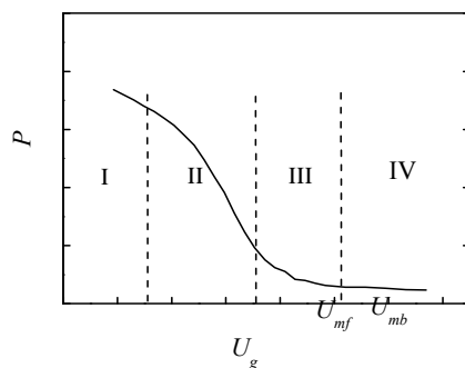
图6.6 搅拌功率与流态化关系分析
