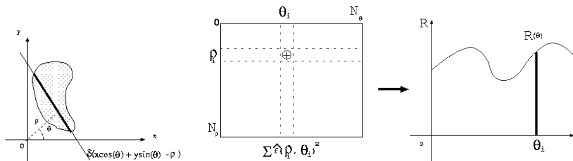
FIG. 1.4 – Définition de la transformée de Radon et calcul de la \mathcal{R} -signature à partir de la matrice de Radon (repris de [TW02]).
