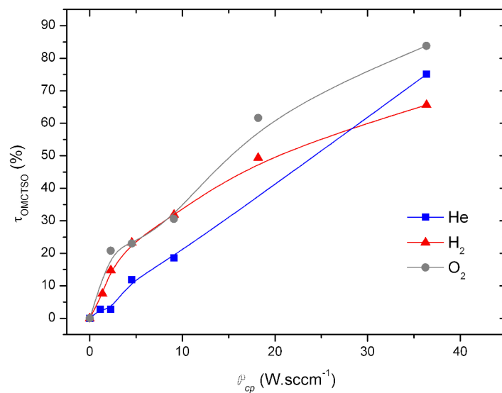
FIGURE 4.16 – Évolution du taux de fragmentation du précurseur dans la décharge en fonction de \mathcal{P}_{cp} .
