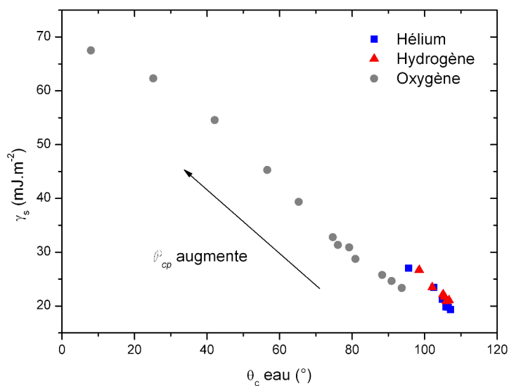
FIGURE 5.1 – Représentation des matériaux obtenus par les trois cas étudiés pour différentes valeurs de \mathcal{P}_{cp} dans l'espace \gamma_s = f(\theta_c^{\text{eau}}) .
