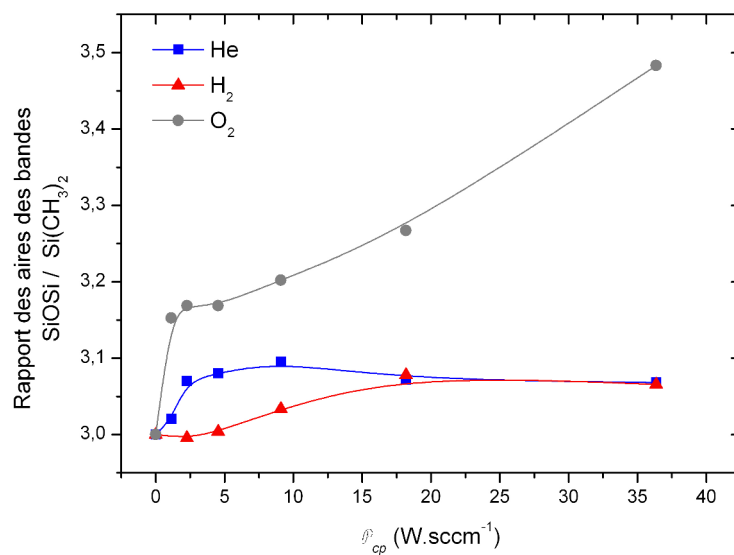
FIGURE 4.17 – Évolution du rapport de la somme des aires des bandes d'absorption des groupements SiOSi sur l'aire de la bande d'absorption des groupements Si(CH 3 ) 2 en fonction de \mathcal{P}_{cp} .
