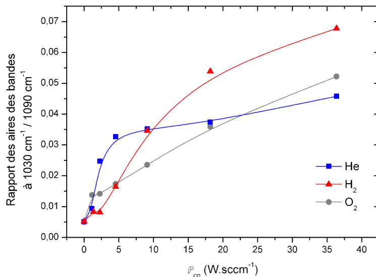
FIGURE 4.18 – Évolution du rapport des aires des bandes d'absorption des vibrations \nu_{as} SiOSi à 1030\text{ cm}^{-1} et 1090\text{ cm}^{-1} en fonction de \mathcal{P}_{cp} .
