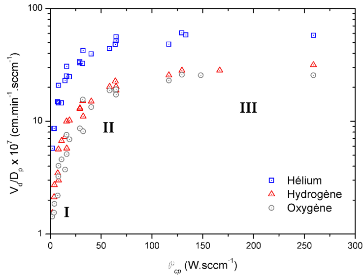
FIGURE 3.6 – Représentation \frac{V_d}{D_p} = f(\mathcal{P}_{cp}) pour les trois cas étudiés.
