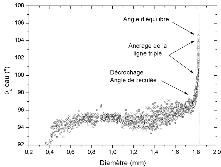
FIGURE 5.7 – Mise en évidence du phénomène d'ancrage de la ligne triple par le suivi de l'angle de contact d'une goutte d'eau de 10\ \mu\text{L} sur une surface de polydiméthylcyclosiloxane plasma au cours de son évaporation.
