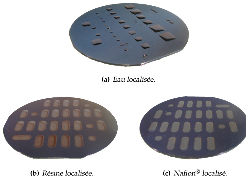
FIGURE 6.1 – Exemples de localisations macroscopiques par simple trempage sur tranches de silicium de 100 mm revêtues de 100 nm polydiméthylcyclo-siloxane plasma traité localement par exposition à un plasma d'hélium.
