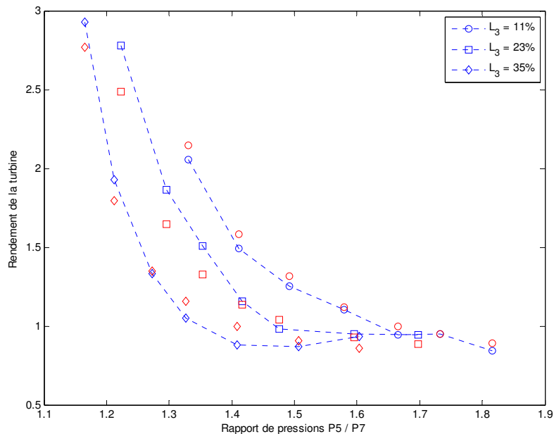
Figure 4.37 – Validation du modèle de rendement global de la turbine, données expérimentales : courbes pointillées, modèle : motifs non reliés. Er_{moy} = 4.3\% , Er_{max} = 8.9\% .
