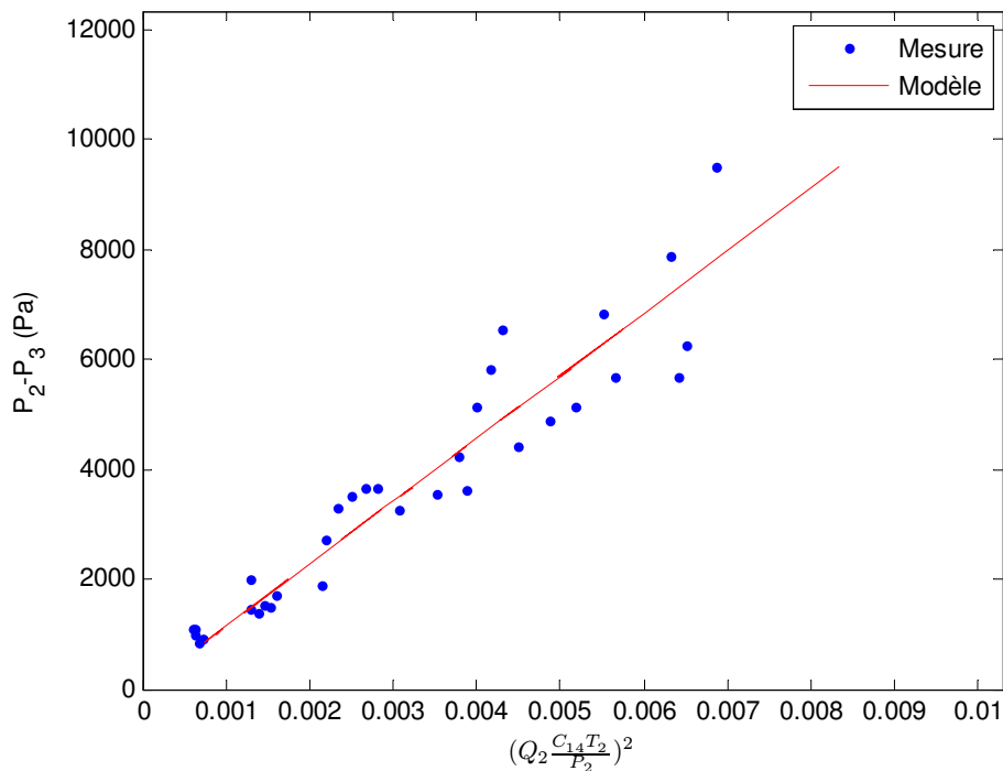
Figure 4.9 – Validation de la perte de charge à travers l'échangeur de refroidissement de l'air comprimé, Er_{\text{moy}} = 5.4\% , Er_{\text{max}} = 8.6\% .
