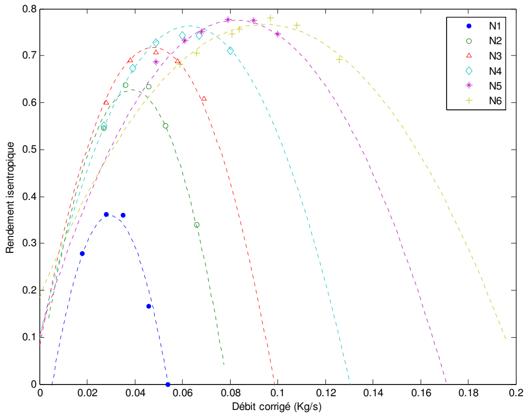
Figure 4.6 – Rendement isentropique du compresseur illustré par des points de mesures, chaque régime de rotation \omega_1=N_i (avec N_1 < N_2 < N_i \dots ) est représenté par un groupe de points, les courbes pointillées représentent les résultats de modélisation.
