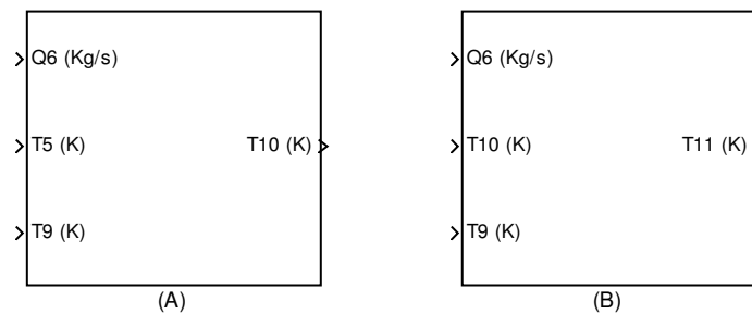
4.25 – Diagramme synoptique du modèle global du conduit de retour d' EGR , (A) sens direct, (B) sens inverse des gaz.
