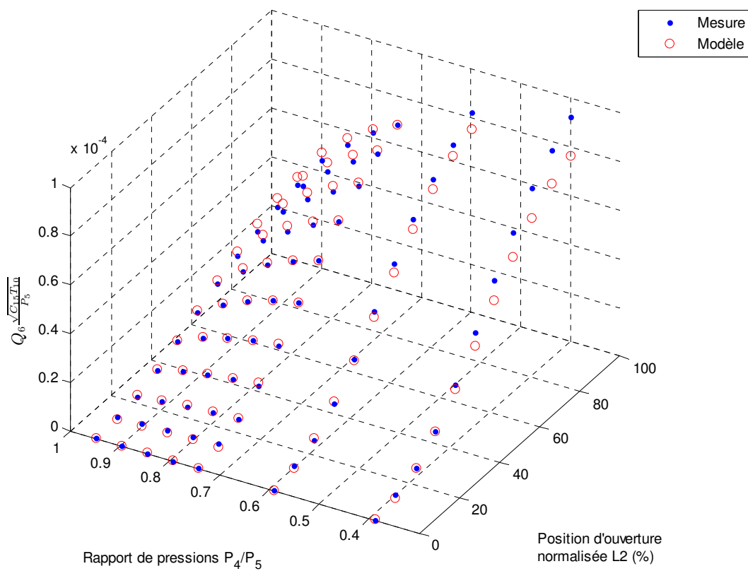
Figure 4.27 – Validation du modèle de débit corrigé des gaz traversant l'électrovanne d'EGR, Er_{moy} = 3.2\% , Er_{max} = 6.9\% .
