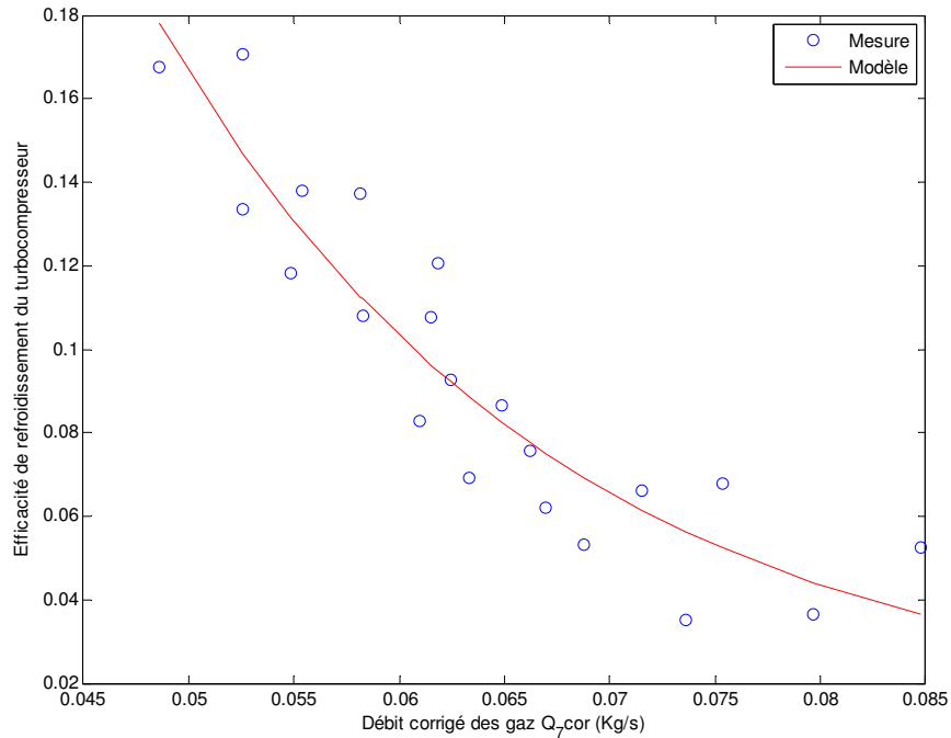
Figure 4.36 – Efficacité de refroidissement de la structure métallique du turbocompresseur, Er_{moy} = 2.2\% , Er_{max} = 3.8\% .
