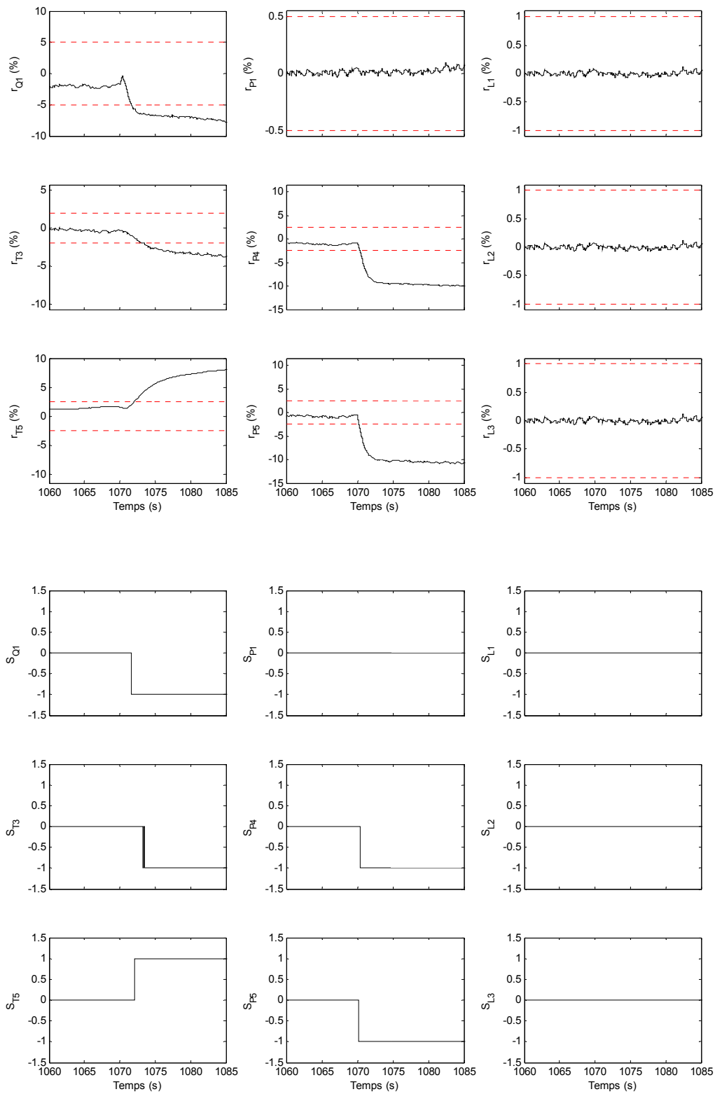
Figure 6.16 – Résultats expérimentaux des résidus et des symptômes correspondants obtenus dans le cas d’une fuite dans le circuit d’échappement du moteur diesel.
