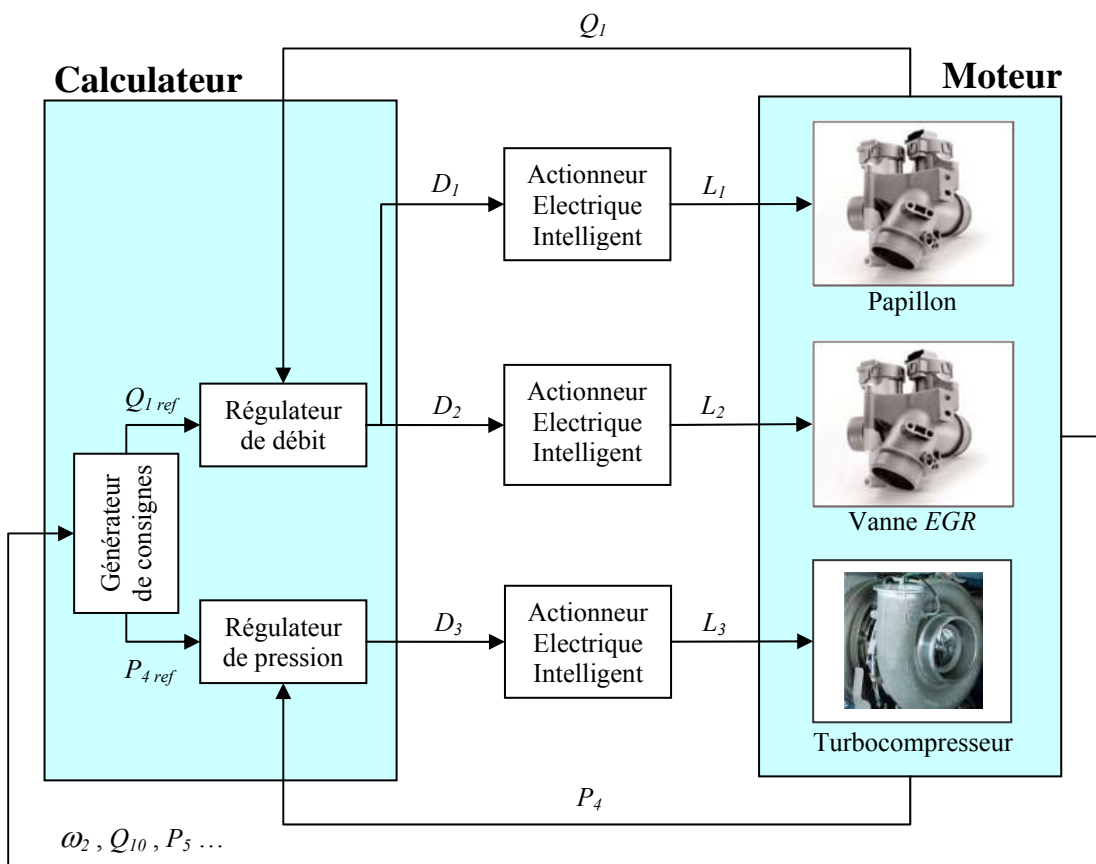
Figure 6.1 – Diagramme synoptique de la gestion de la boucle des gaz du moteur diesel.
