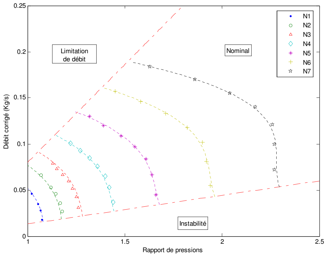
Figure 4.5 – Domaine de fonctionnement du compresseur défini par des points de mesures, chaque régime de rotation \omega_1=N_i (avec N_1 < N_2 < N_i \dots ) est représenté par un groupe de points, les courbes pointillées représentent les résultats de modélisation.
