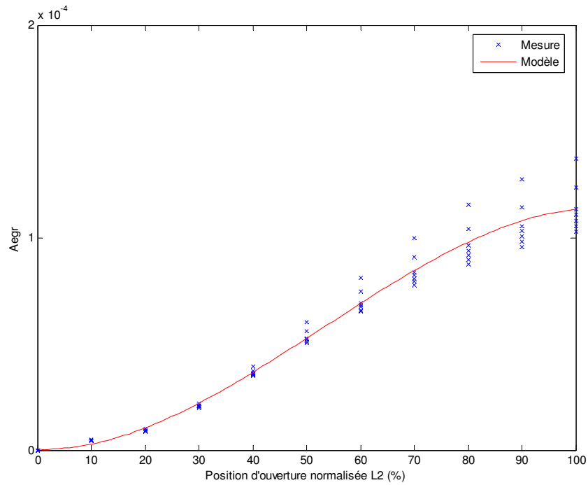
Figure 4.26 – Validation de la fonction A_{egr} de l'électrovanne d'EGR, Er_{moy} = 3.7\% , Er_{max} = 7.9\% .
