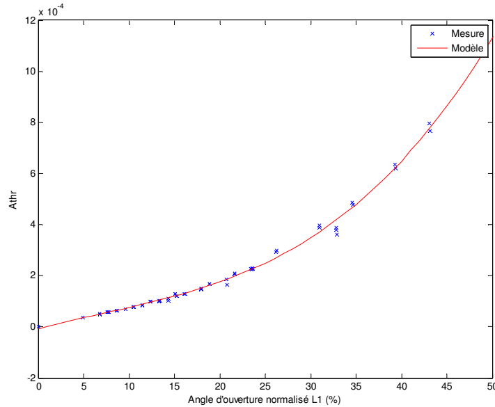
Figure 4.13 – Validation de la fonction A_{thr} du volet d'admission,
