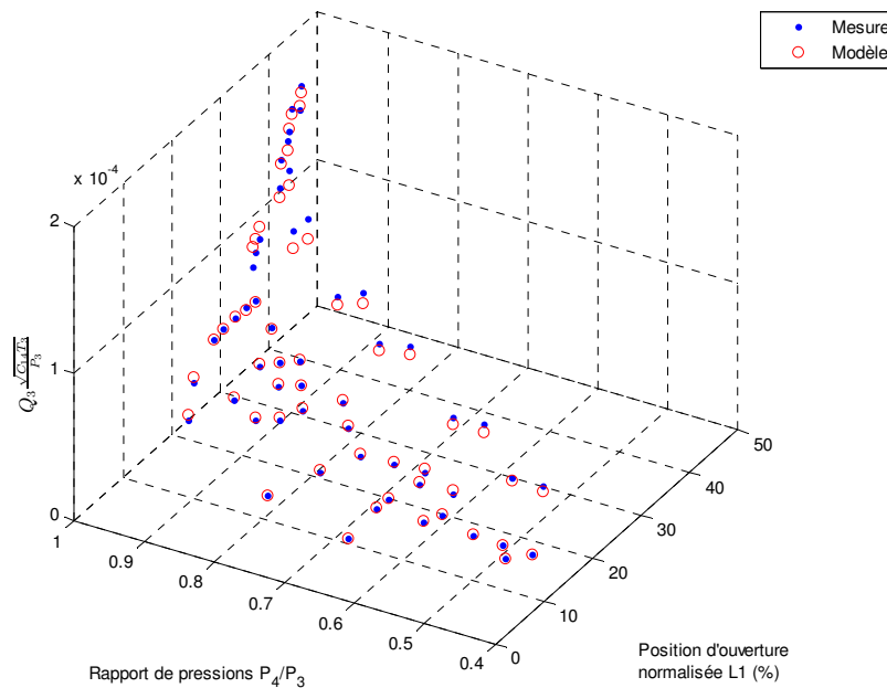
Figure 4.14 – Validation du modèle de débit corrigé du volet d'admission,
