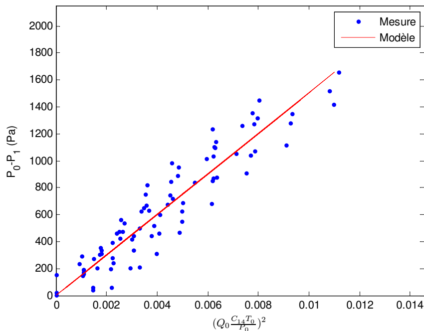
Figure 4.3 – Validation de la perte de charge à travers le filtre à air,
