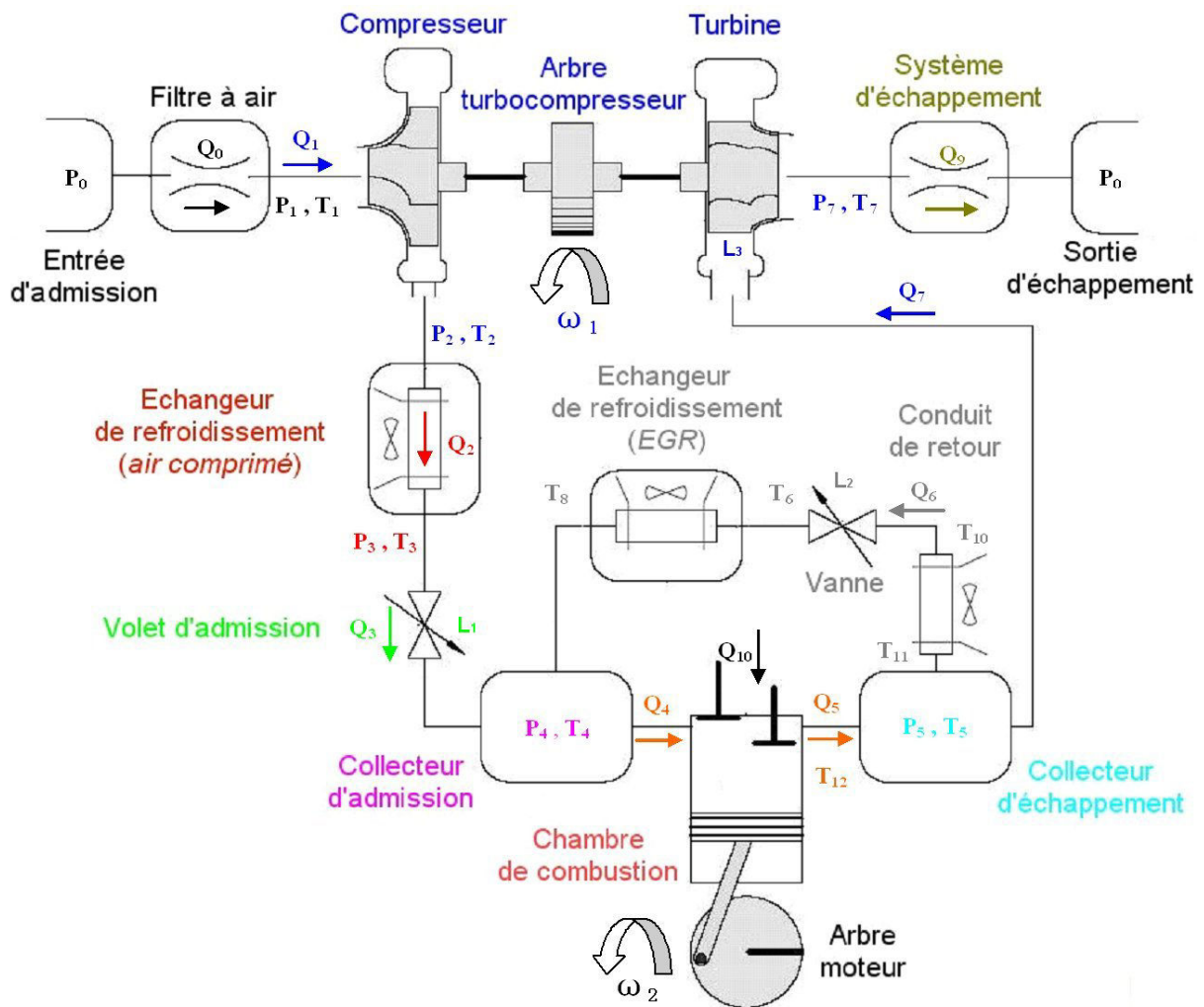
Figure 4.2 – Diagramme schématique de la boucle des gaz du moteur diesel DaimlerChrysler OM646.
