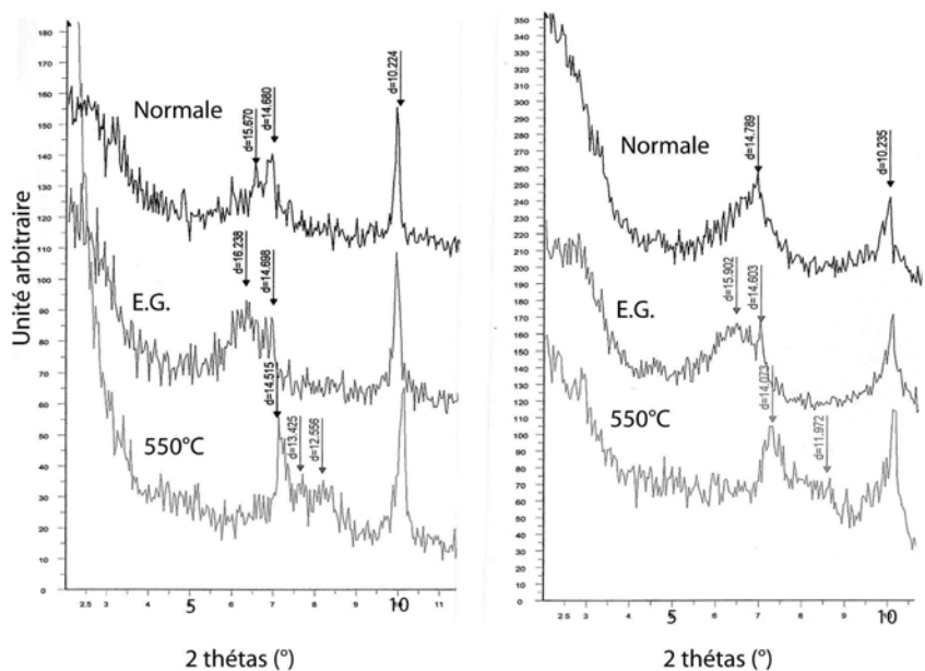
Figure 32: exemples de diffractogrammes de la phase argileuse des Marnes Irisées Inférieures ; normale : lame normale ; E.G. : saturée en éthylène-glycol, 550°C : chauffée à 550°C).
