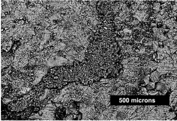
Figure 150: fente remplie de gypse microgrenu recoupant une plage de gypse grenue (imagerie en électrons rétrodiffusés).
