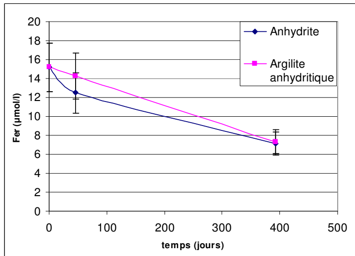
Figure 102: évolution des concentrations en fer dissous dans les batch contenant de la saumure de cavité et des "marnes irisées inférieures".
