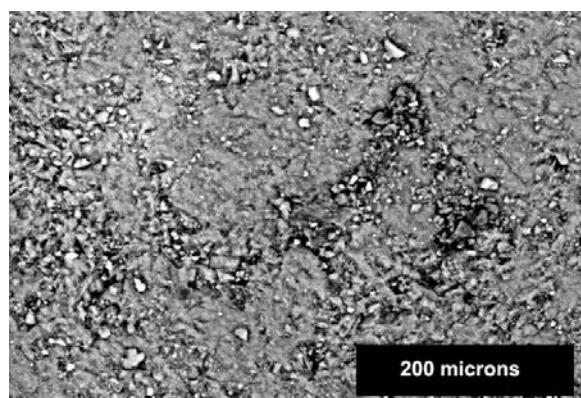
Figure 146: microprismes d'anhydrite (en blanc) diffuse au sein de gypse grenu (imagerie en électrons rétrodiffusés).
