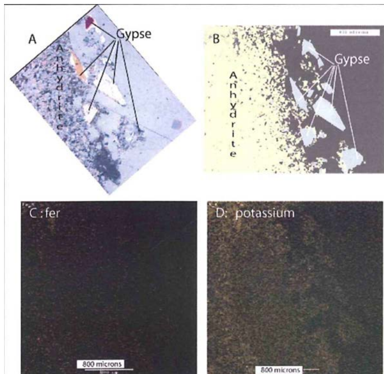
Figure 107 : section de la bordure du faciès anhydrite immergé dans de l'eau pendant 190 jours. A : microscopie optique, B : microscopie en électrons rétrodiffusés ; C : cartographie X du Fer ; D : cartographie X du potassium.
