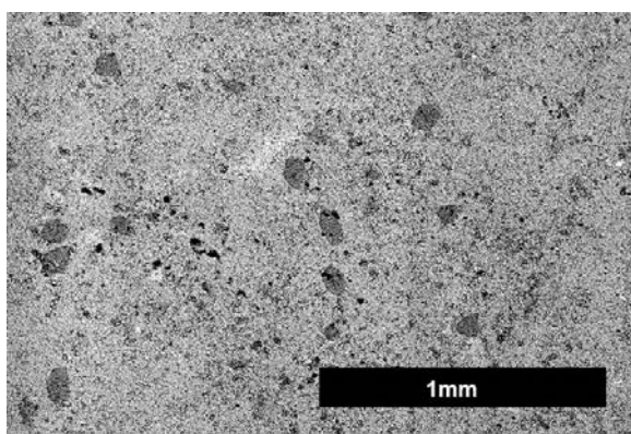
Figure 145: texture grenue du gypse recoupée par des nodules de dolomite (gris sombre). (imagerie en électrons rétrodiffusés).
