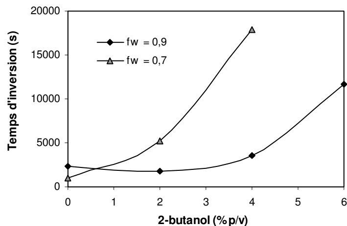
Figure V-1 : Influence de la concentration d'alcool sur le temps d'inversion ( fw=0,7 ) ou de déclenchement de l'inversion ( fw=0,9 )
