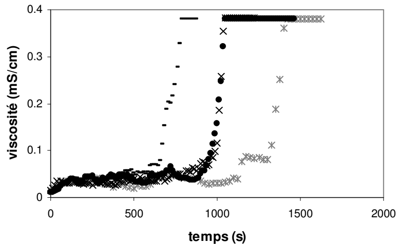
Figure IV-13 : Reproductibilité du temps de propagation des émulsions. f_w = 0,9 , HLD = 1,84
