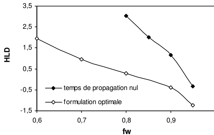
Figure IV-16 : HLD requis pour que l'inversion soit immédiate
