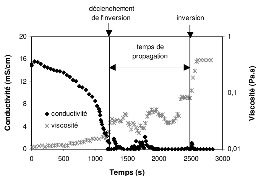
Figure IV-11 : Suivis conductimétrique et rhéologique d'un système à fw 0,9
