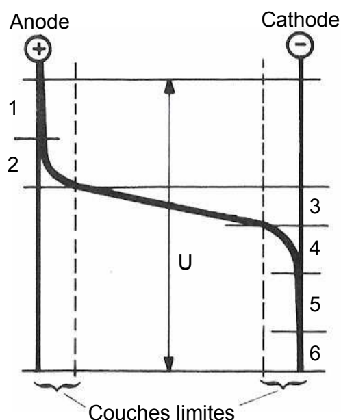
Figure 1-2 : Evolution du potentiel électrique à l'intérieur d'une cellule [Coeuret et Stork 1993].
