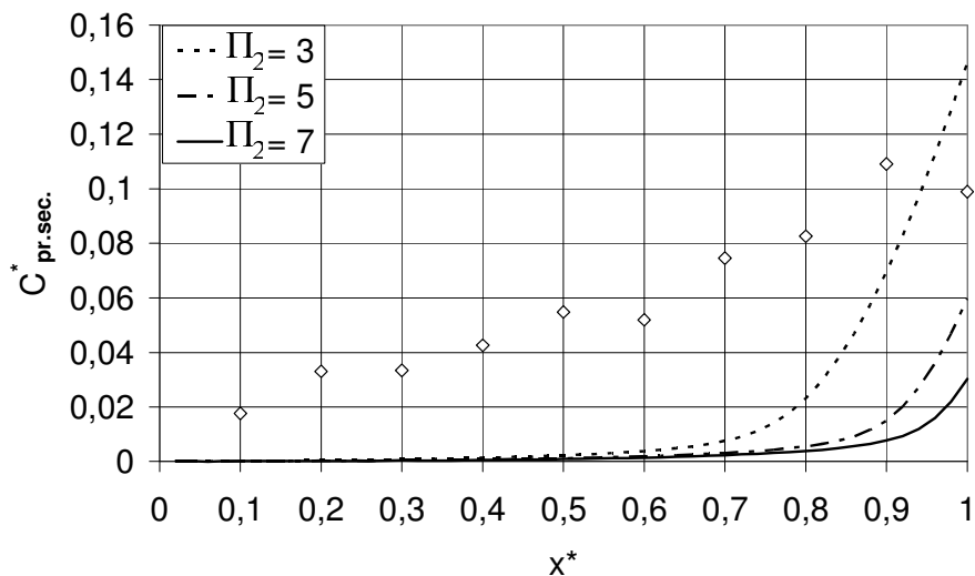
Figure 4-41: Comparaison entre les concentrations adimensionnelles des sous-produits à partir des mesures expérimentales ( \square )- C_{A0}=0,1 M, Q_V=0,2 ml/min, C_{KF}=0,01 M- et celles obtenues à partir du modèle pour \Pi_1=80 et pour \Pi_2=3, 4, 5, 7 et 14 , le long du réacteur.
