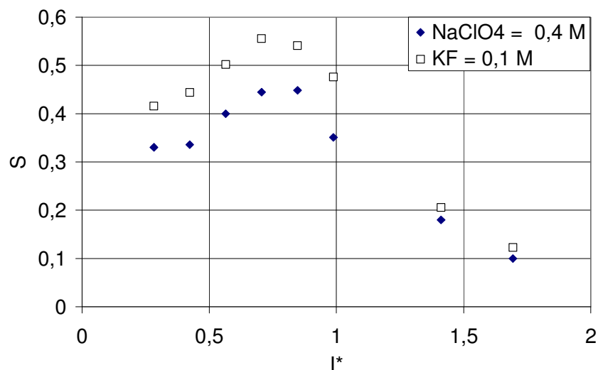
Figure 4-10: Variation de la sélectivité en fonction de I^* pour une concentration initiale en réactif de 0,01 M dans le méthanol en présence de 0,1 M de KF ou de 0,4 M de NaClO 4 et pour un débit du liquide de 0,6 ml/min.
