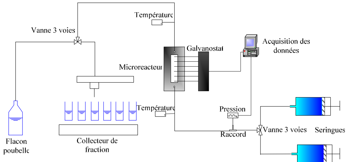
Figure 4-5: Dispositif expérimental.
