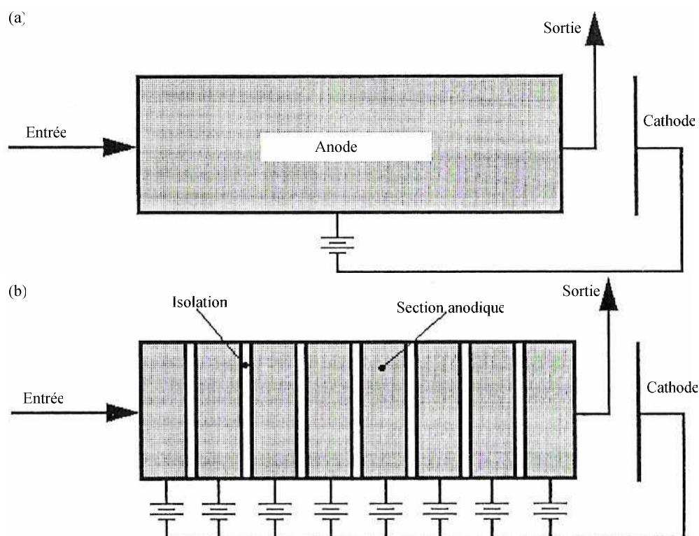
Figure 1-8 : Comparaison entre un réacteur électrochimique à lit fluidisé (a) et le réacteur à électrode segmentée (b) [Matlosz 2001].
