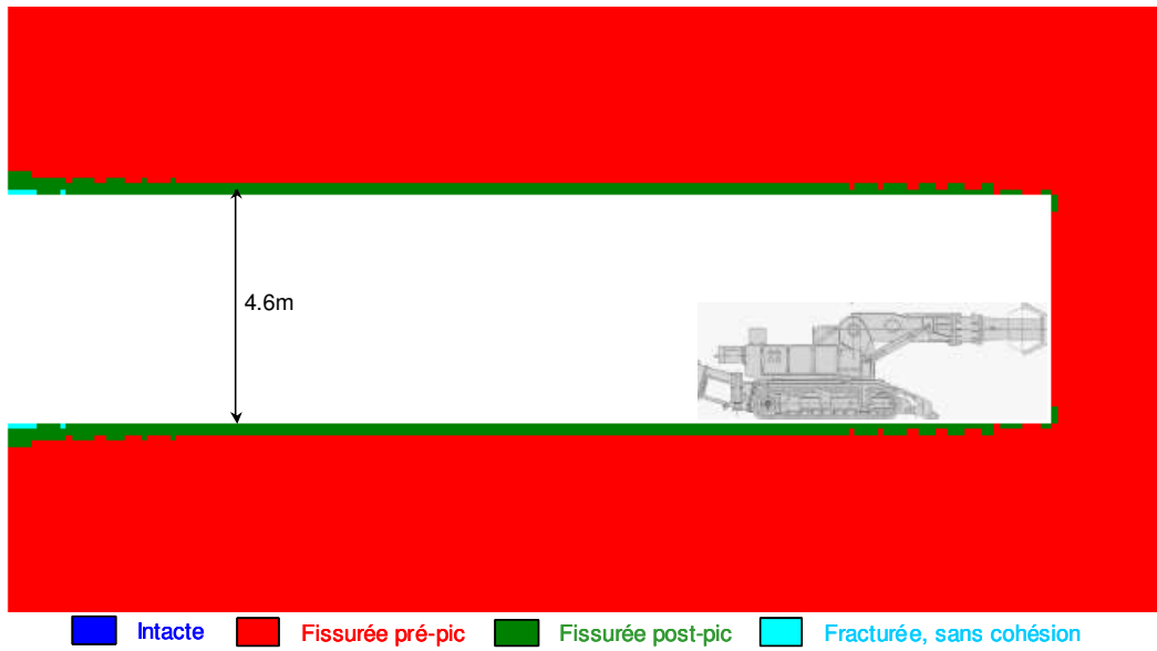
Figure 7.44 - Résultats de la première modélisation axisymétrique de la galerie GMR
