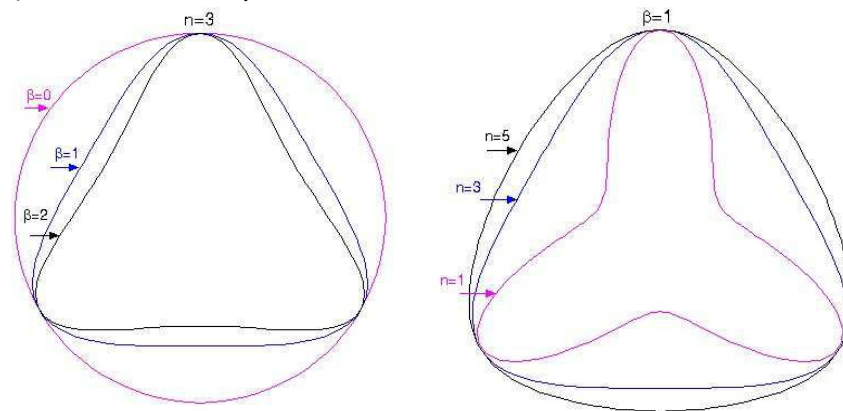
La convexité du critère est assurée pour \beta \leq 1
