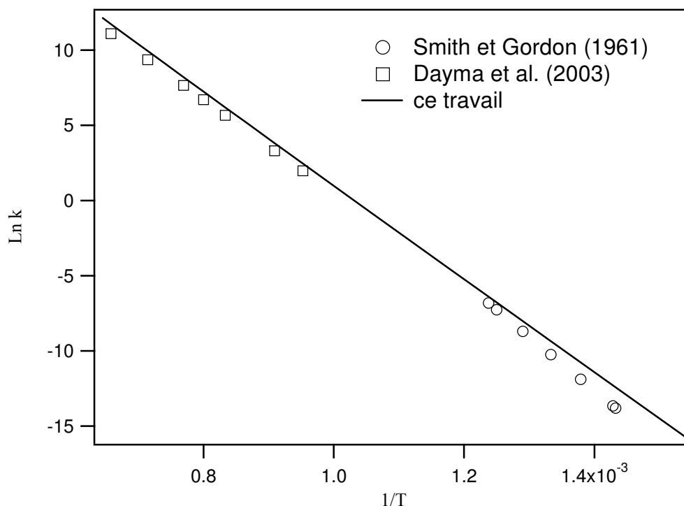
Figure 39 : Comparaison entre la constante calculée et les données de la littérature pour la réaction \text{CHX} \rightarrow \text{CHXD} + \text{H}_2 .
