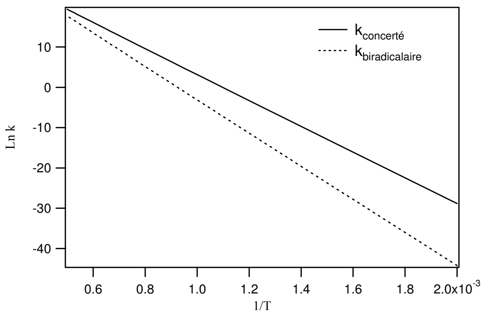
Figure 37 : Comparaison entre les constantes de vitesse obtenues pour la réaction cyclohexène \rightarrow 1,3-butadiène + éthylène selon un mécanisme concerté ou biradicalaire (voir texte). Avec 500 K < T < 2000K.
