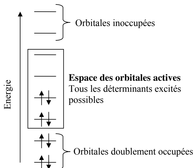
Figure 6 : Illustration de la répartition des OM dans le formalisme CASSCF.
