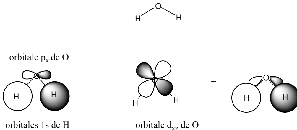
Figure 3 : OM formées par combinaison entre l'orbitale 1s de H et l'orbitale p_x de O. L'inclusion de l'orbitale d_{xz} de O améliore la description de la liaison O-H dans H_2O (adapté de Cramer (2004)).
