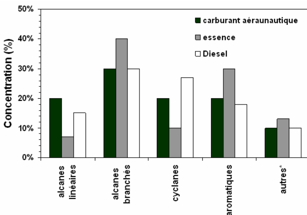
Figure 1 : Concentration des différentes classes d'hydrocarbures dans les carburants usuels : essences, Diesel et carburants aéronautiques. Adapté de Westbrook (2005).
