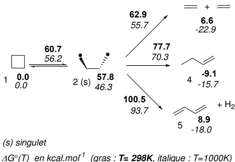
Figure 1 : Schéma de décomposition du cyclobutane. Conformations de plus basses énergies libres au niveau CBS-QB3.
