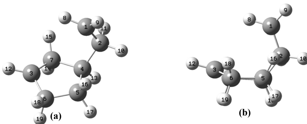
Figure 26 : Géométrie au niveau UB3LYP/cbsb7 de l'état de transition impliqué dans la réaction \text{NBN} \rightarrow \text{BR2} . (a) vue de \frac{3}{4} dessus, (b) vue de coté.
