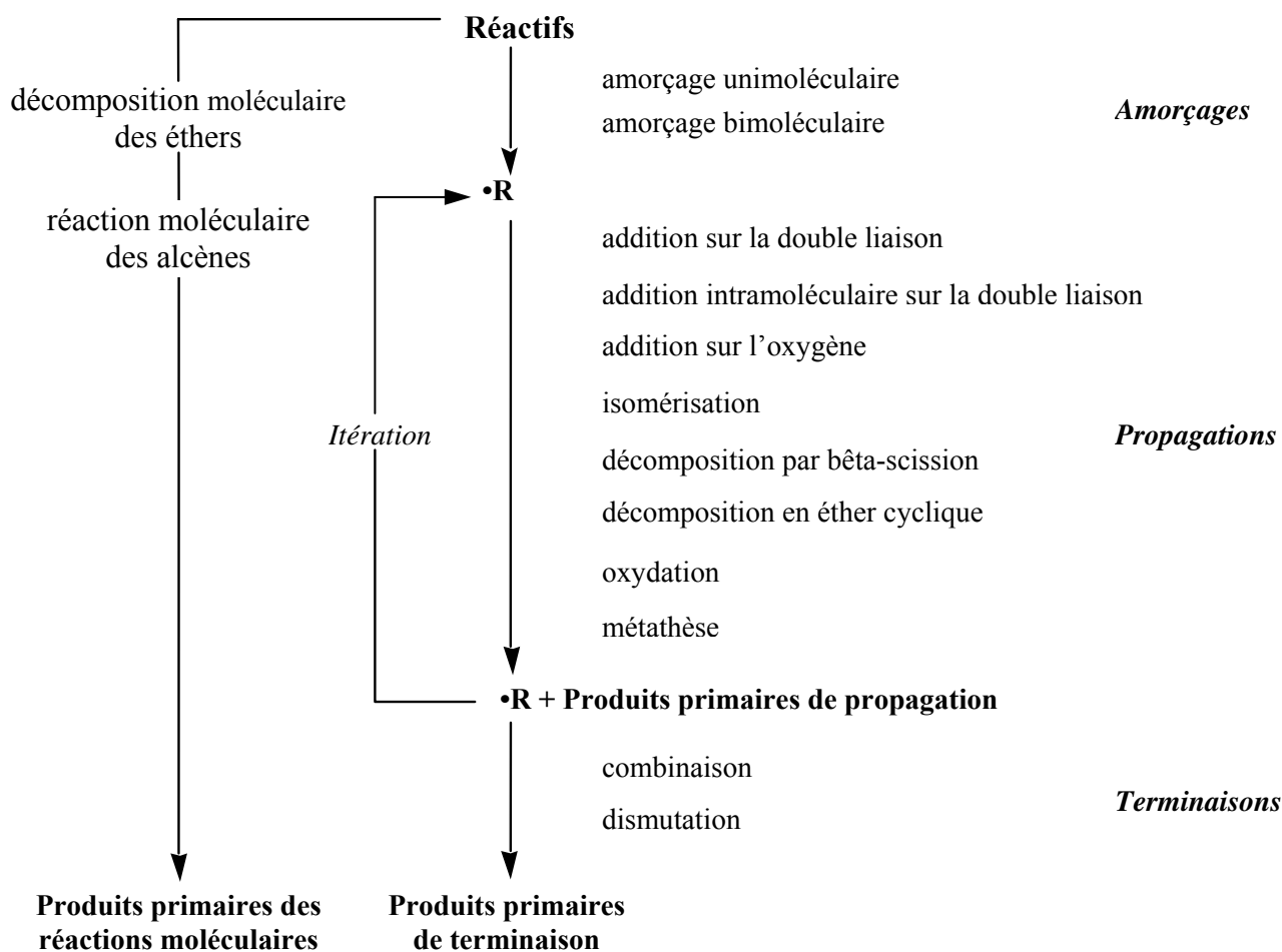
Figure 7 : Algorithme de génération exhaustive du mécanisme primaire
