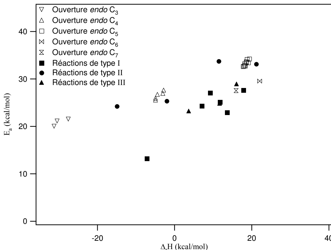
Figure 25 : Corrélation de type Evans-Polanyi établie pour les réactions d'ouverture endo de radicaux alkyles monocycliques et bicyclics selon le type de réaction envisagé (voir texte).
