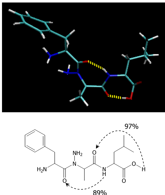
Figure 54 : Visualisation des liaisons hydrogène dans l'oligomère II-1.
