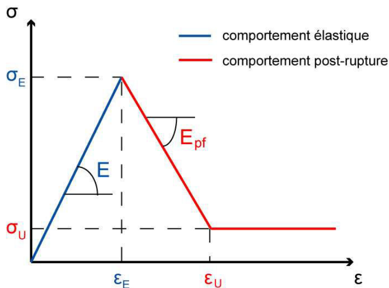
Figure 3.7. Loi de comportement de type « amortissement de contrainte »
