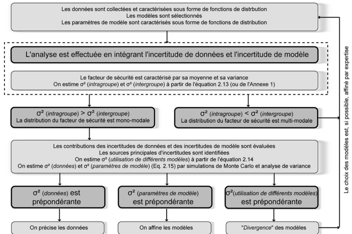
Figure 2.13. Méthodologie pour la prise en compte et le traitement des diverses sources d'incertitudes rencontrées dans une analyse
