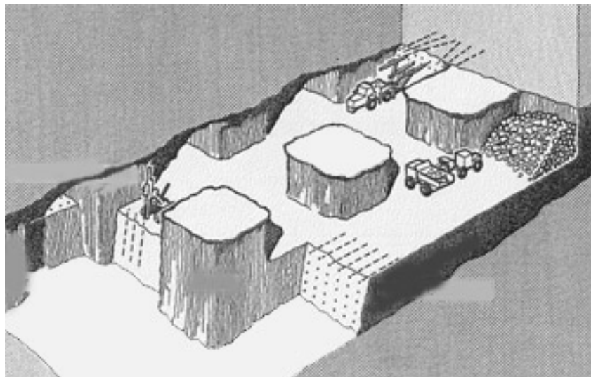
Figure 2.4. Exploitation partielle par chambres et piliers abandonnés (source : Stassen, 1982)
