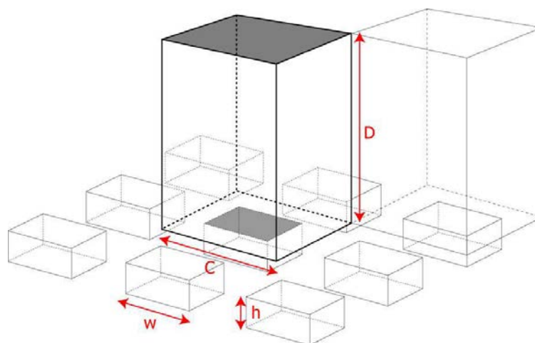
Figure 3.3. Notations utilisées pour les dimensions géométriques
