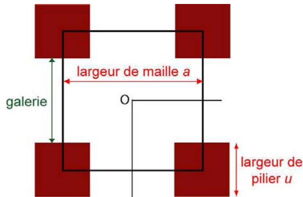
Figure 3.21. Notations et géométrie utilisée dans le modèle de la plaque reposant sur quatre piliers
