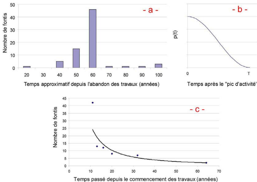
Figure 2.21. Evolution temporelle des fontis en Pennsylvanie de l'Ouest (a, Dyne, 1998), Modèle proposé pour l'évolution du nombre de fontis après le pic d'activité (b, Richards et al., 2002), et Décroissance du nombre de fontis à Holwell (Grande-Bretagne) (c, Swift et Reddish, 2002)
