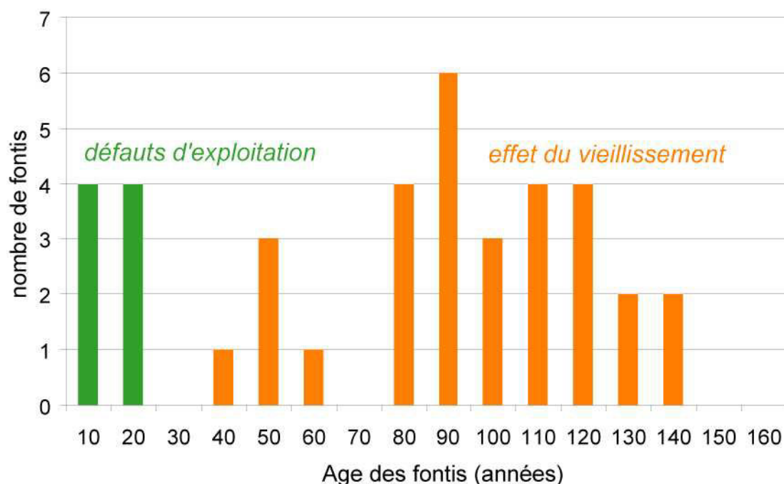
Figure 2.22. Evolution des fontis au droit de la mine de Siemianowice
