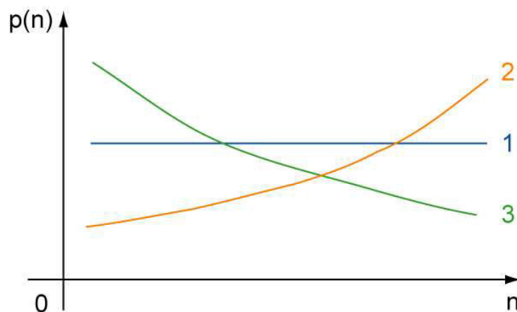
Figure 2.2. Evolutions de la probabilité d'un événement dommageable durant l'année n , conditionnellement à la non-occurrence de cet événement jusqu'à la fin de l'année n-1 (d'après Durville, 2004)
