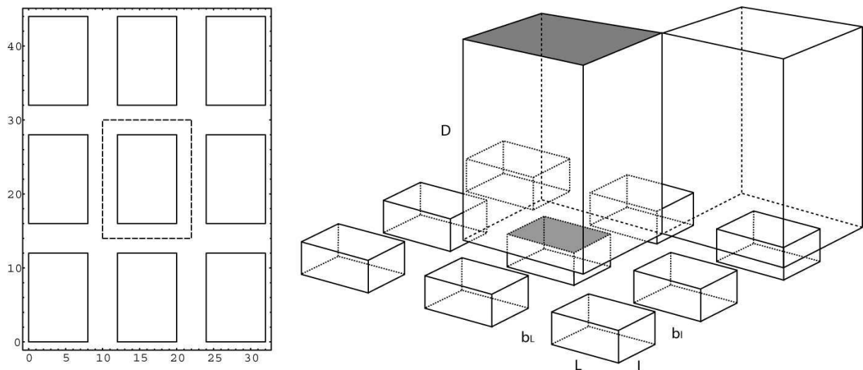
Figure 2.6. Système de neuf piliers utilisé pour l'étude (a) et Modèle de l'aire tributaire (b)
