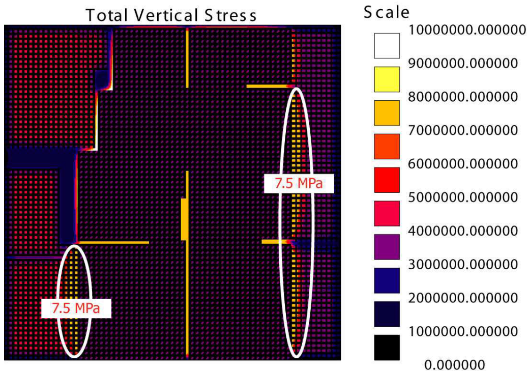
Figure 3.9. Contrainte verticale qui s'exerce sur les piliers (en Pa) après affaiblissement des piliers du Secteur C
