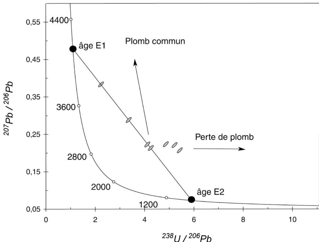
Figure A5-2 : Diagramme concordia Tera-Wasserburg (Tera et Wasserburg, 1972). Les rapports isotopiques ne sont pas corrigés du plomb commun.
