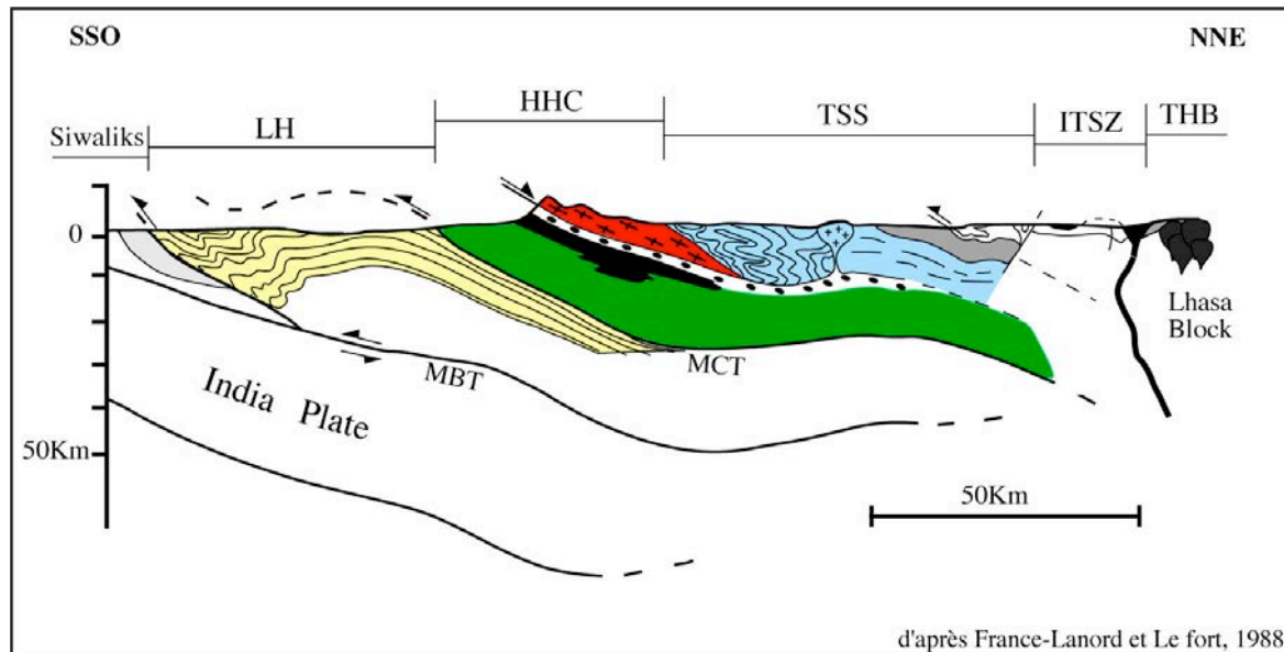
Figure 1.2 : Coupe géologique schématisée de l'Himalaya du Népal Central. THB : Batholite du Trans-Himalaya, ITSZ : Zone de Suture de l'Indus-Tsangpo, TSS : Séries sédimentaires Téthysiennes, HHC : Haut Himalaya Cristallin, LH : Moyen Pays, MCT : Main Central Thrust, MBT : Main Boundary Thrust. Modifiée d'après France-Lanord et Le Fort (1988).
