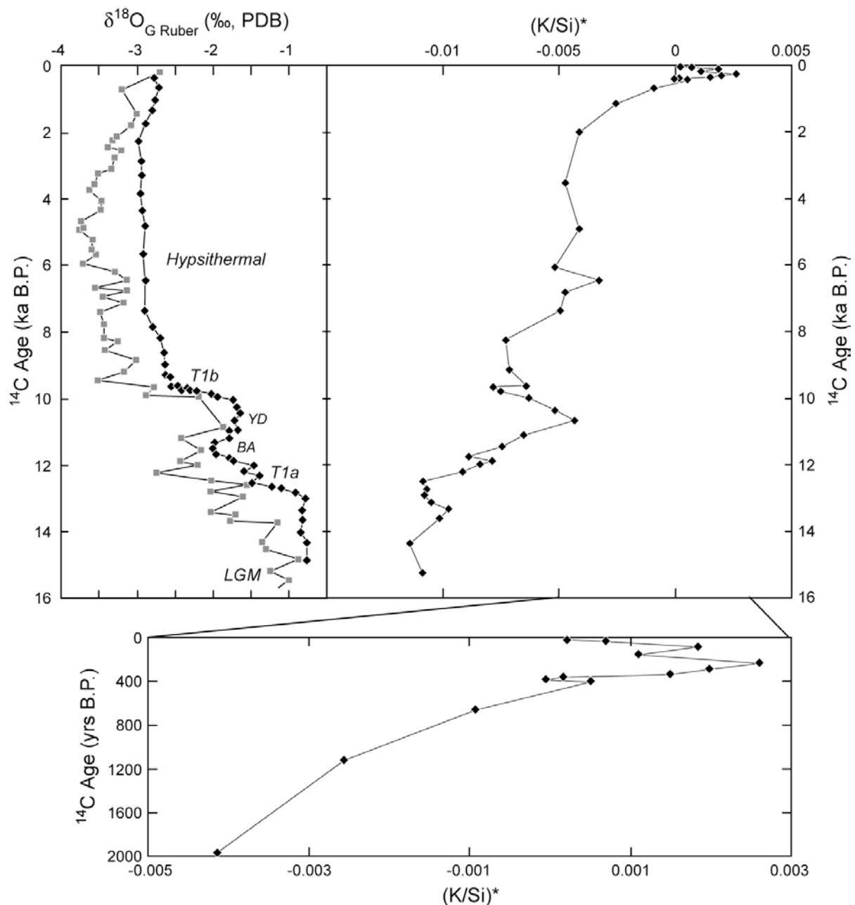
Figure 3.20 : Evolution temporelle du rapport (\text{K/Si})^* des sédiments du Cône du Bengale comparée à l'évolution du \delta^{18}\text{O} des foraminifères planctoniques. Les données de \delta^{18}\text{O} des sédiments de la carotte 120KL (diamants noirs) et de la carotte 126KL (carrés gris) sont issues de Weber et al. (1997). Au cours des derniers 16 ka, le rapport (\text{K/Si})^* montre deux périodes d'augmentation brutale. La première, entre 13 et 11 ka, correspond à la déglaciation documentée par le \delta^{18}\text{O} des foraminifères. La seconde, au cours du dernier millénaire, ne correspond pas à un changement climatique majeur et est probablement liée à une activité anthropique intense dans le bassin.
