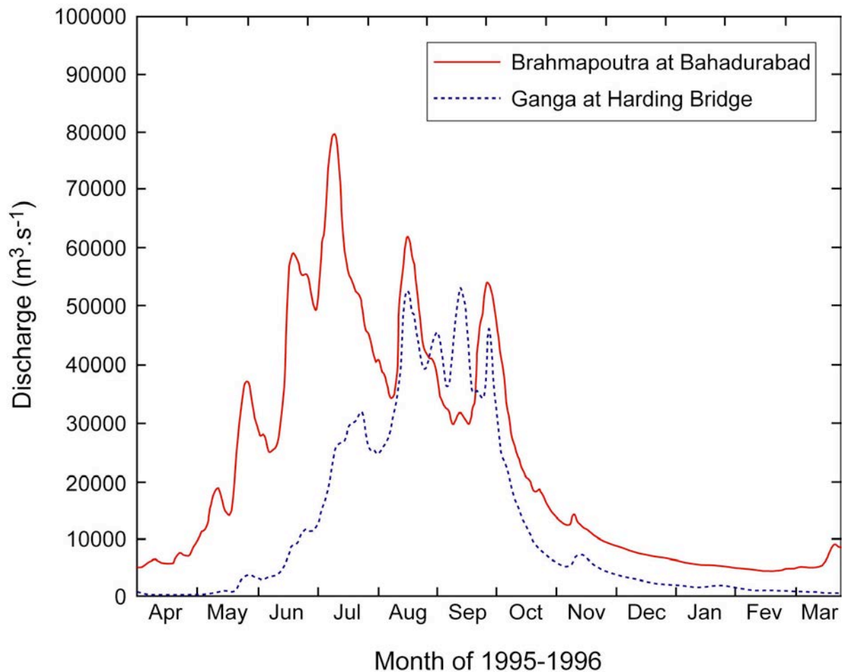
Figure 1.7 : Hydrogramme du Brahmapoutra à Bahadurabad (Bangladesh) et du Gange à Hading Bridge (Bangladesh) pour l'année hydrologique 1995-1996. L'essentiel du débit est imputable à la période de la mousson d'été (Juin-Septembre). Le retard de l'augmentation de débit du Gange est classique et correspond à une arrivée plus tardive de la mousson sur l'Ouest de la chaîne Himalayenne. La localisation précise des sites de mesure est indiquée sur la figure 1.3. Les données sont issues du rapport RSP (RSP, 1996).
