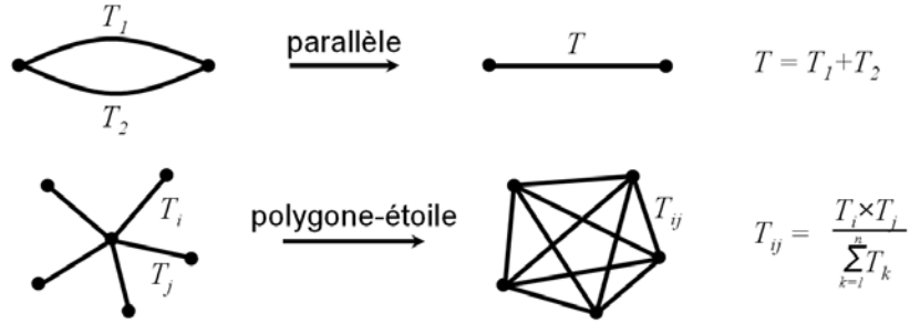
FIG. 4.3 – Transformations électriques (parallèle et polygone-étoile) et les équations associées
