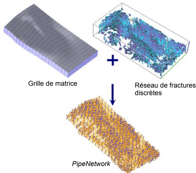
FIG. 2.24 – Génération d’un PipeNetwork à partir d’un modèle fracturé constitué d’une grille basée blocs et d’un réseau de fractures discrètes
