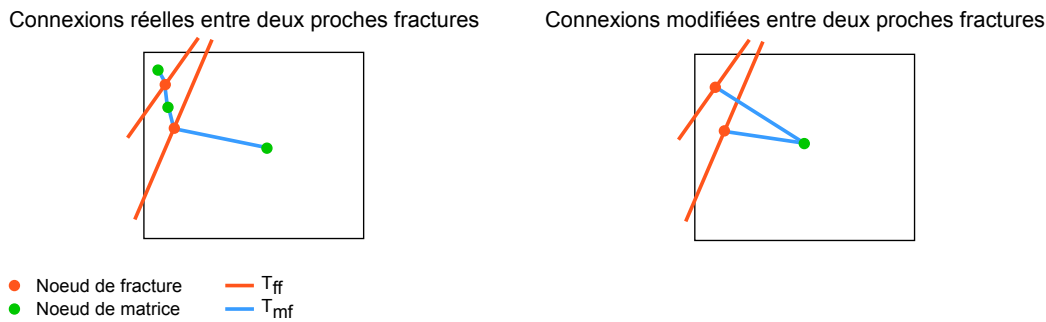
FIG. 2.38 – Altération des échanges entre fractures proches
