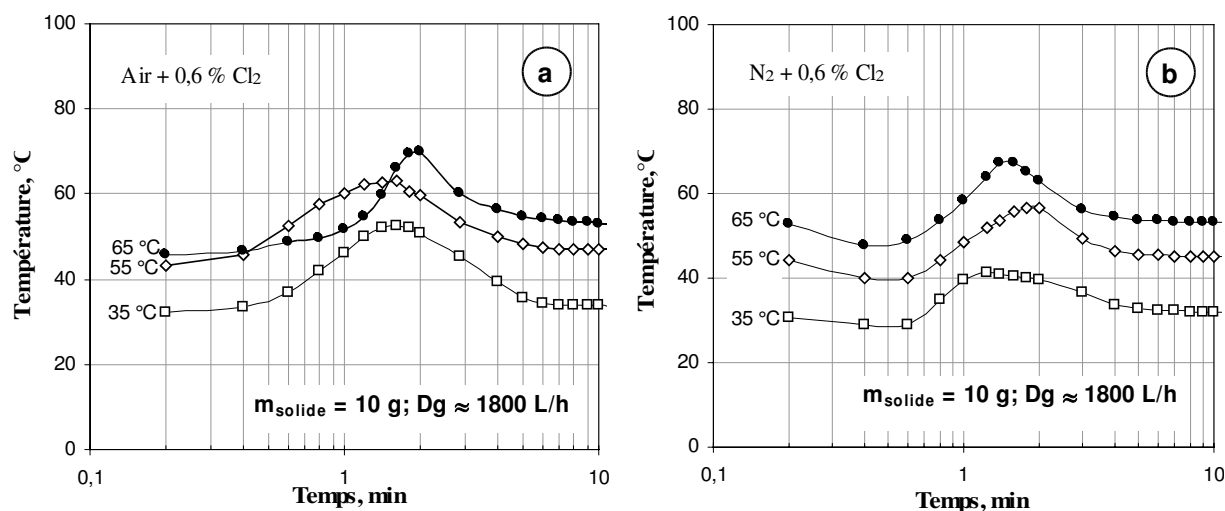
Figure VI. 13. Résultats tracés en échelle semi-logarithmique de la température en fonction du temps lorsque la teneur en chlore dans les mélanges gazeux utilisés (air + Cl 2 ), (N 2 + Cl 2 ) est de 0,6 %.
