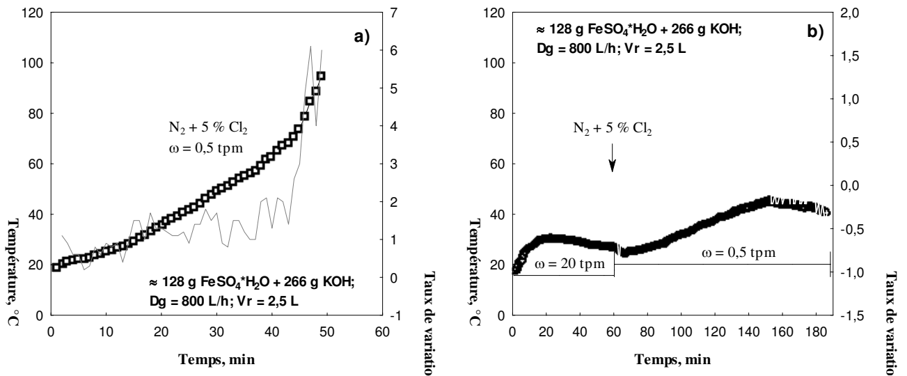
Figure IV. 8. Effet du mode opératoire sur le déroulement de la synthèse lors de l'usage d'azote comme diluant pour les séries de tests où l'introduction de (\text{N}_2 + \text{Cl}_2) est respectivement : a) directe et b) différée.
