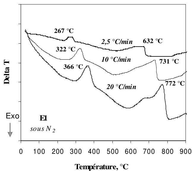
Figure III. 11. Courbes d'ATD pour le traitement de FeSO 4 ·H 2 O (E1) sous N 2 aux vitesses de chauffe de 2,5 ; 10 et 20 °C.min -1 .
