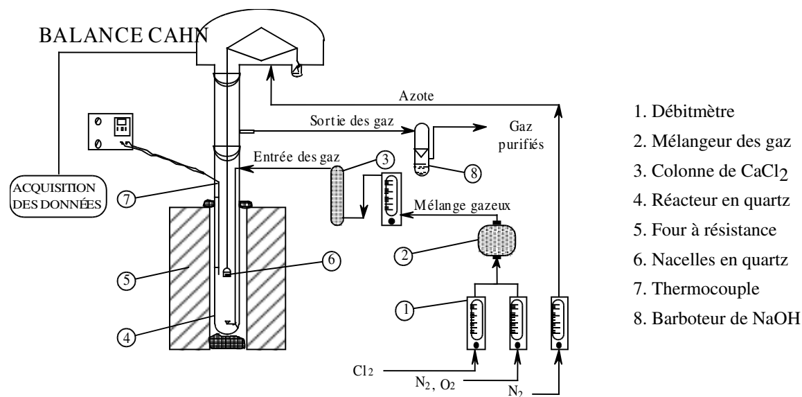
Figure II. 2. Schéma de l'appareillage d'analyse thermogravimétrique.
