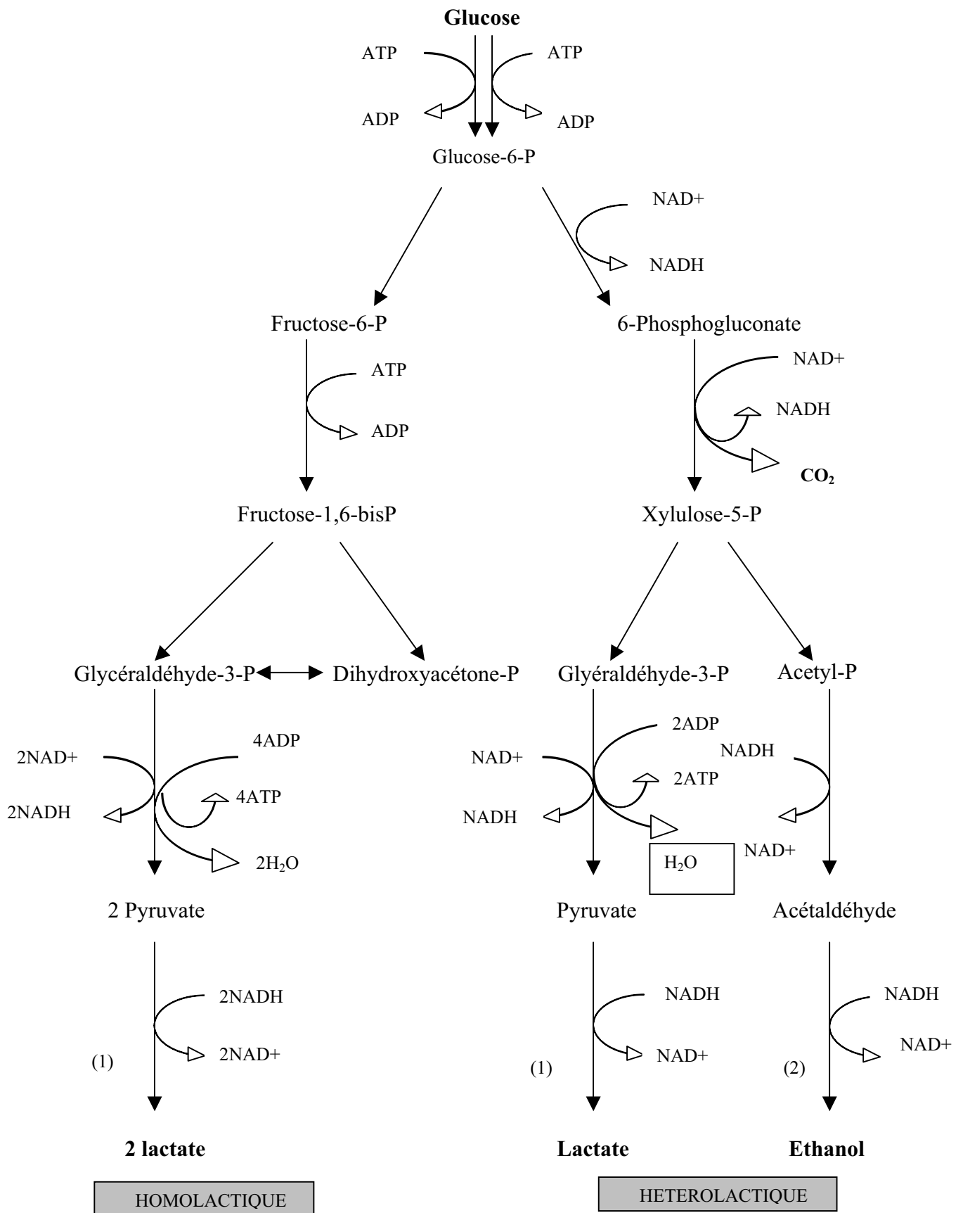
Figure 2.4. Principales voies du métabolisme du glucose par les bactéries lactiques: P, phosphate; ADP, adenosine 5'-diphosphate; ATP, adenosine 5'-triphosphate; NAD + , nicotinamide adénine dinucléotide; NADH, nicotinamide adénine dinucléotide; (1), lactate déshydrogénase; (2), alcool déshydrogénase (Wee et al. , 2006a).
