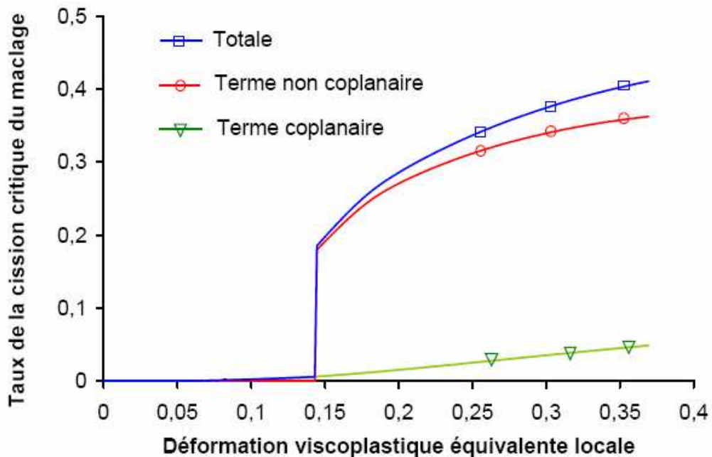
Figure II. 10: Évolution de la valeur des deux termes (coplanaires et non coplanaires) du taux de la cission critique du maclage \dot{\tau}_c^{(I)} pour le système de macle primaire en fonction de la déformation viscoplastique équivalente locale.
