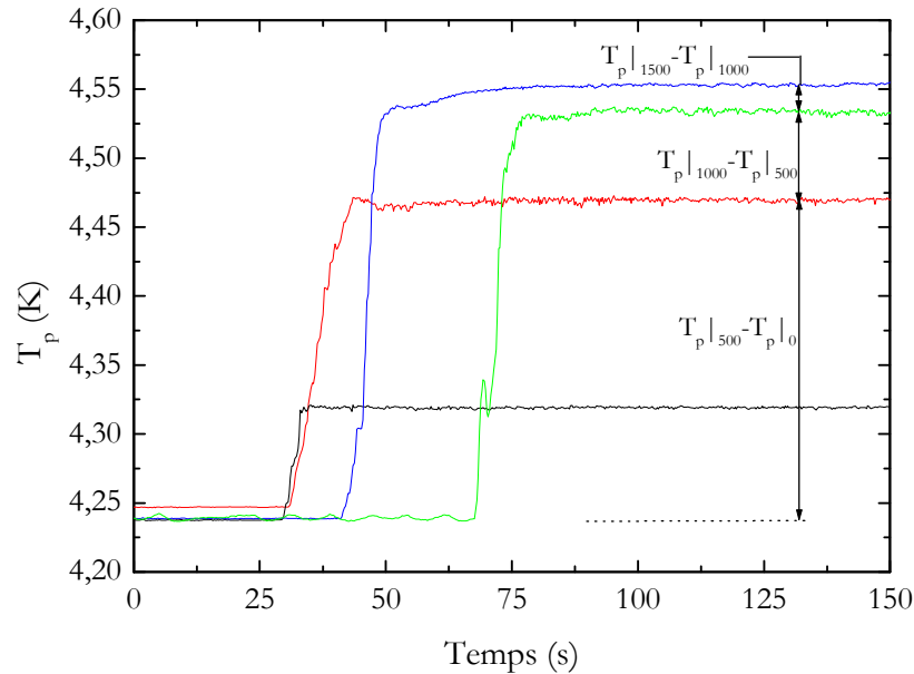
Figure V.2. Réponse temporelle de la sonde de température Ge située à z=0,07 m pour différentes densités de flux de chaleur : – 100 \text{W/m}^2 , – 500 \text{W/m}^2 , – 1000 \text{W/m}^2 , – 1500 \text{W/m}^2 .
