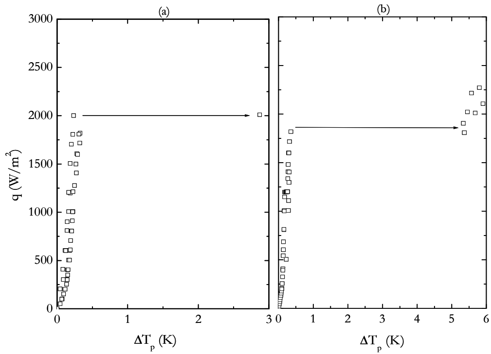
Figure V.29. Courbes d'ébullition jusqu'à l'apparition de la crise d'ébullition près de l'entrée du tube d'essai Ø10 : (a) z=0,07 m, (b) z=0,3 m.
