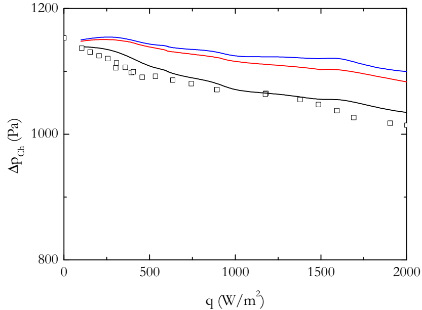
Figure IV.9. Évolution de la chute de pression \Delta p_{\text{Ch}} avec le flux de chaleur q pour le tube d'essai \text{Ø}10 prédite par : – modèle homogène, – corrélation de Friedel et Huq, – corrélation de Levy.
