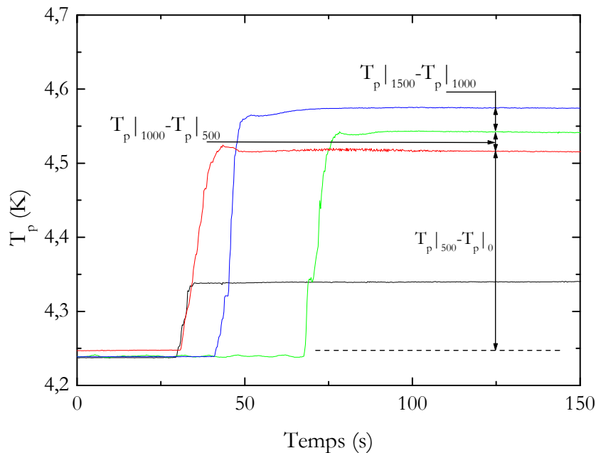
Figure V.3. Réponse temporelle de la sonde de température Ge située à z=0,3 m pour différentes densités de flux de chaleur : – 100 \text{W/m}^2 , – 500 \text{W/m}^2 , – 1000 \text{W/m}^2 , – 1500 \text{W/m}^2 .
