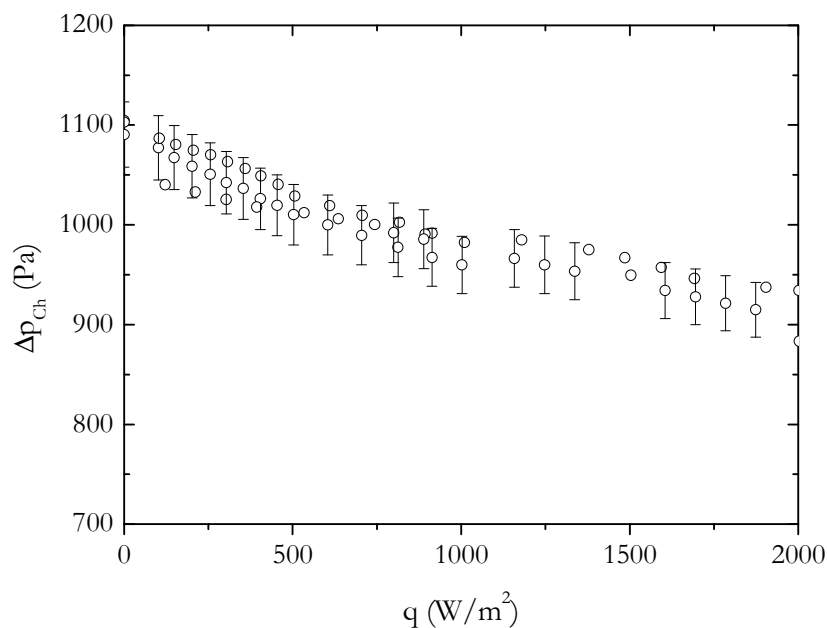
Figure IV.2. Évolution de la différence de pression \Delta p_{\text{Ch}} le long de la partie chauffée en fonction du flux de chaleur q pour le tube \text{Ø}10 .
