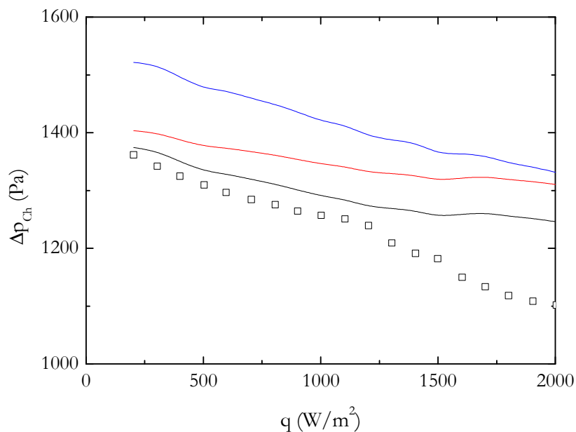
Figure IV.10. Évolution de la chute de pression \Delta p_{\text{Ch}} avec le flux de chaleur q pour le tube d'essai \text{Ø}14 prédite par : – modèle homogène, – corrélation de Friedel et Huq, – corrélation de Levy.
