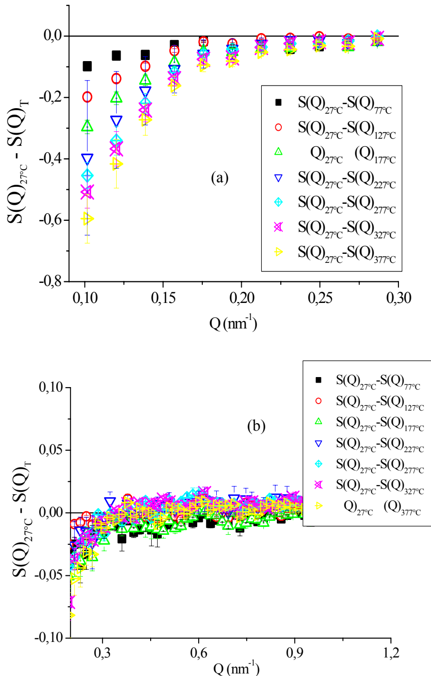
Figure IV-51 : Différence S_{27}(Q) - S_T(Q) , calculée à chaque température T du processus de dévitrification mesuré par DNPA, en fonction de Q , entre 77 et 377^\circ\text{C} : (a) Tout le domaine de Q . (b) Aux grandes valeurs de Q .
