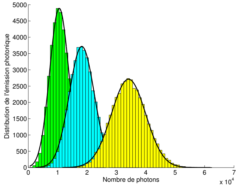
Figure 4.06 – Distribution expérimentale de l'émission photonique pour \delta = 1ms .
