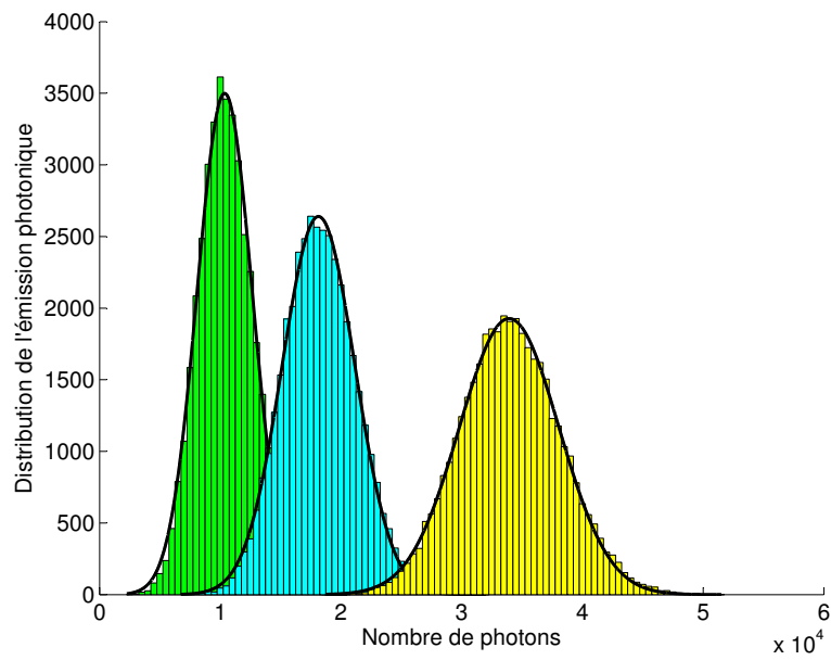
Figure 4.07 – Distribution expérimentale de l'émission photonique pour \delta = 2ms .
