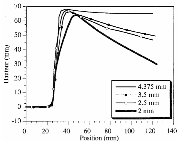
Figure 6.9 – Profils après retour élastique de l'essai «Omega» pour différentes tailles d'éléments [19].
