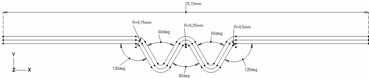
Figure 3.8 – Géométrie et données dimensionnelles de la pièce.
