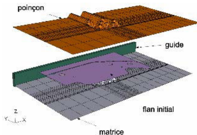
Figure 3.24 – Outils d'emboutissage.
