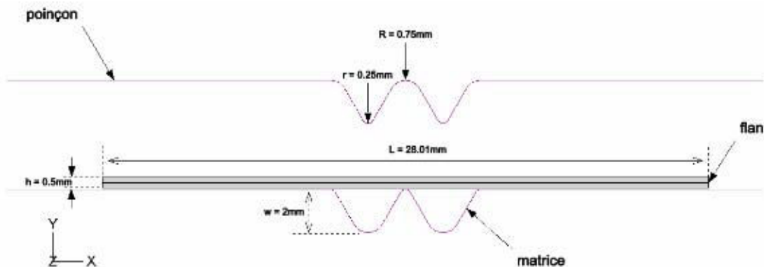
Figure 3.9 – Outils d'emboutissage.
