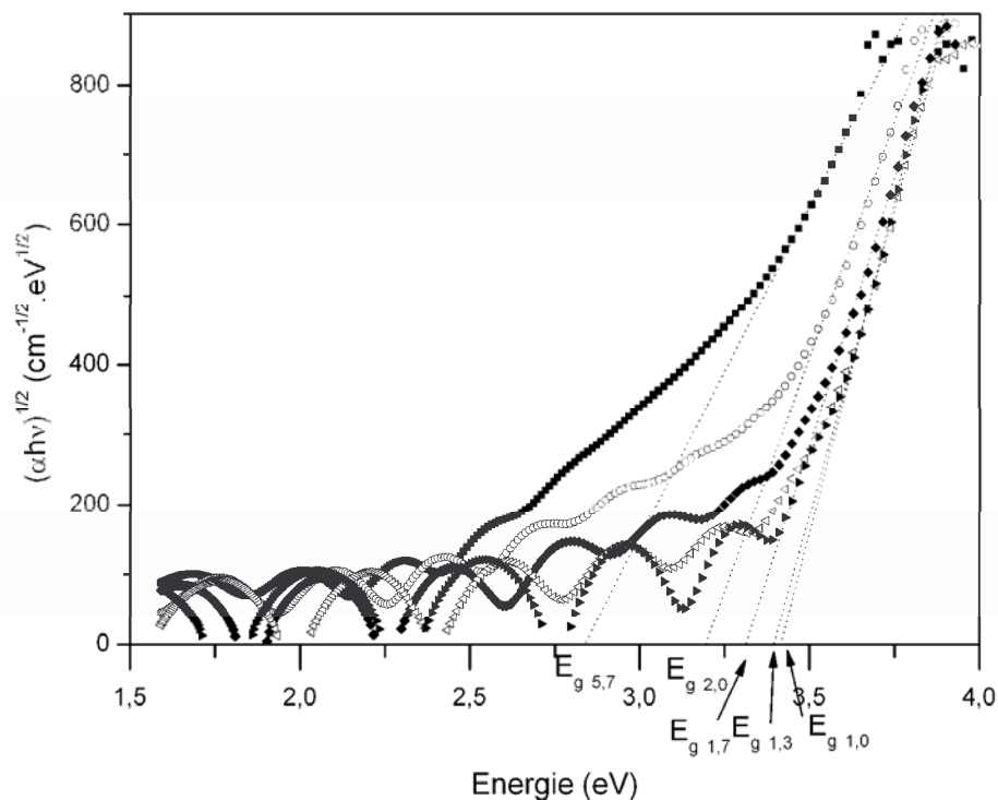
Figure 4-29 : Courbes de T_{auc} (\alpha hv)^{1/2} en fonction de l'énergie des photons pour les revêtements de TiO_{2-x}N_y de diverses teneurs en azote (■ 5,7 ○ 2,0 ◆ 1,7 ◁ 1,3 et ► 1,0 % at. N)
