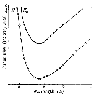
FIG. 1.7 – Spectre infrarouge de la transmittance d'un cristal de \text{Bi}_2\text{Te}_3 suivant les polarisations \vec{E} // \vec{c} et \vec{E} \perp \vec{c}
