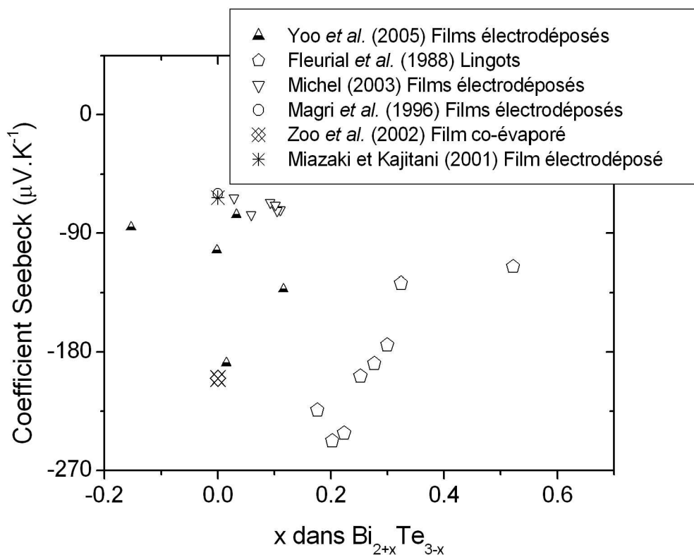
FIG. 1.17 – Variation du coefficient Seebeck en fonction de la composition en bismuth (x) dans Bi_{2\pm x}Te_{3\mp x}
