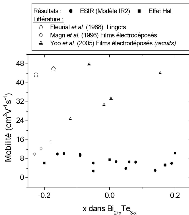
FIG. 3.54 – Evolution comparée de la mobilité pour différentes compositions de films électrodéposés de Bi_2Te_3 par ellipsométrie spectroscopique infrarouge (ESIR, via le modèle IR2) et par des mesures électriques (effet Hall).
