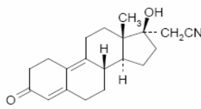
Dienogest
