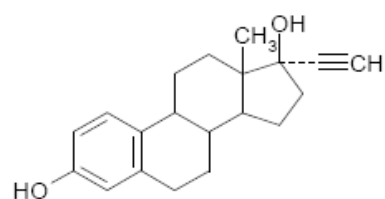
17- \alpha -ethinylestradiol
