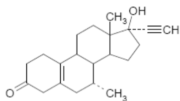
Tibolone
