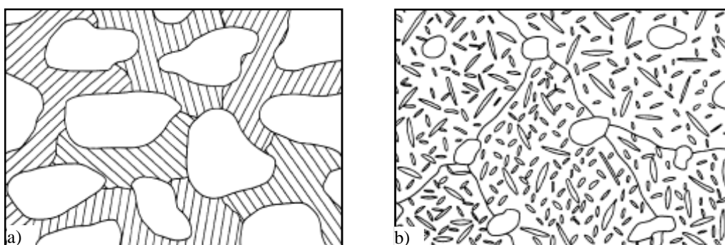
Figure II.21 Représentation schématique d'une microstructure qui est susceptible d'être sensible au fatigue-dwell (a) et d'une microstructure moins sensible au phénomène fatigue-dwell (b) [Gorman 2001]
