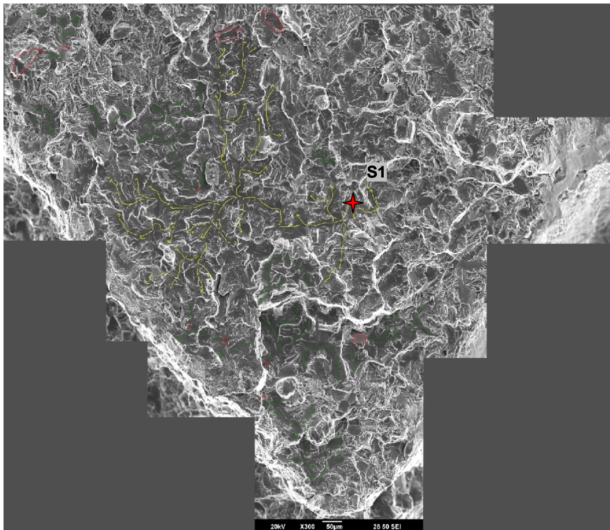
Figure BI260.6 Identification du site d'amorçage dans la région R2 (S1): site d'amorçage principal; en vert- des sites de réamorçage lors de la propagation de la fissure ; en rouge- les stries de fatigue
