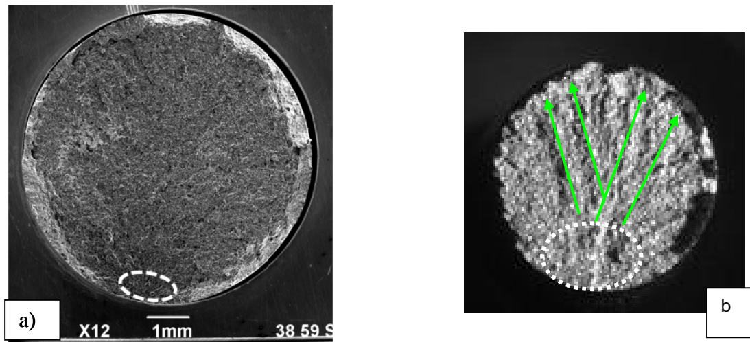
Figure CI10.1 a) Macrographie électronique, b) schéma : zone brillante et marques de chevrons
