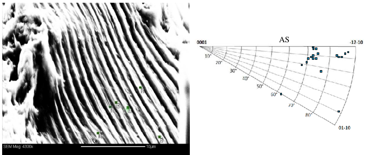
Figure IV.22 Orientations cristallographiques sur les stries de fatigue
