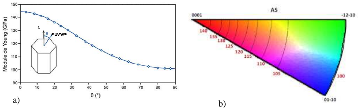
Figure IV.28 a) Evolution du module d’Young de la phase \alpha en fonction de l’angle entre l’axe c et l’axe de sollicitation [Fisher 1964] ; b) triangle standard cartographié en iso-courbes du module d’Young [GPa]
