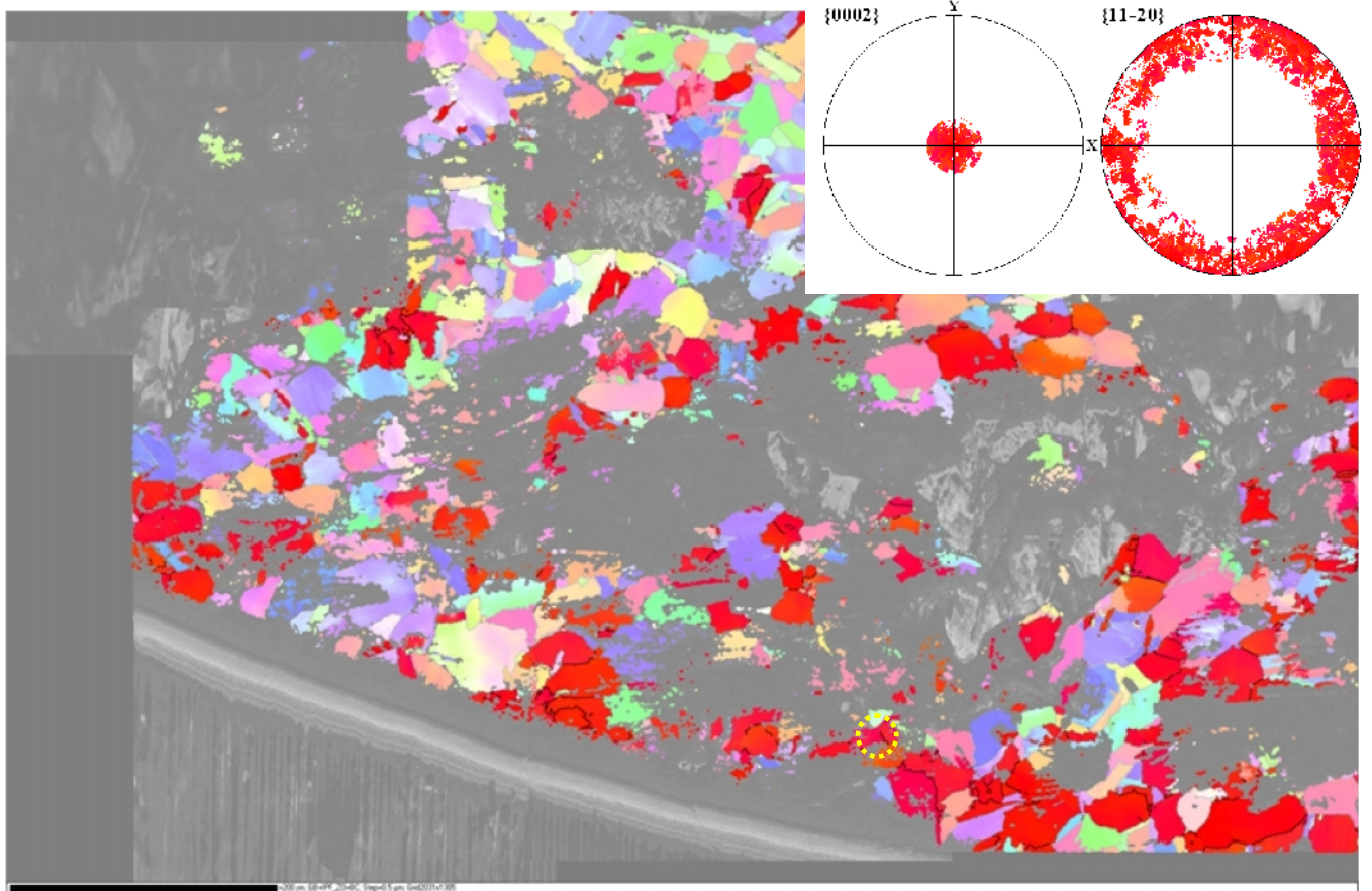
Figure 6.11 Cartographie EBSD dans la région R2, site d'amorçage S4- sélection des grains ayant l'axe c à 25^\circ de AS
