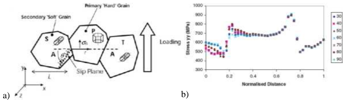
Figure IV.29 a) Représentation de l’orientation cristallographique de trois grains voisins et b) la variation de la contrainte le long de la ligne AA [Dunne 2008]
