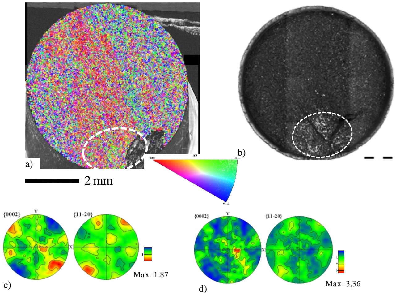
Figure BI260.10 Cartographie EBSD de la section transverse
