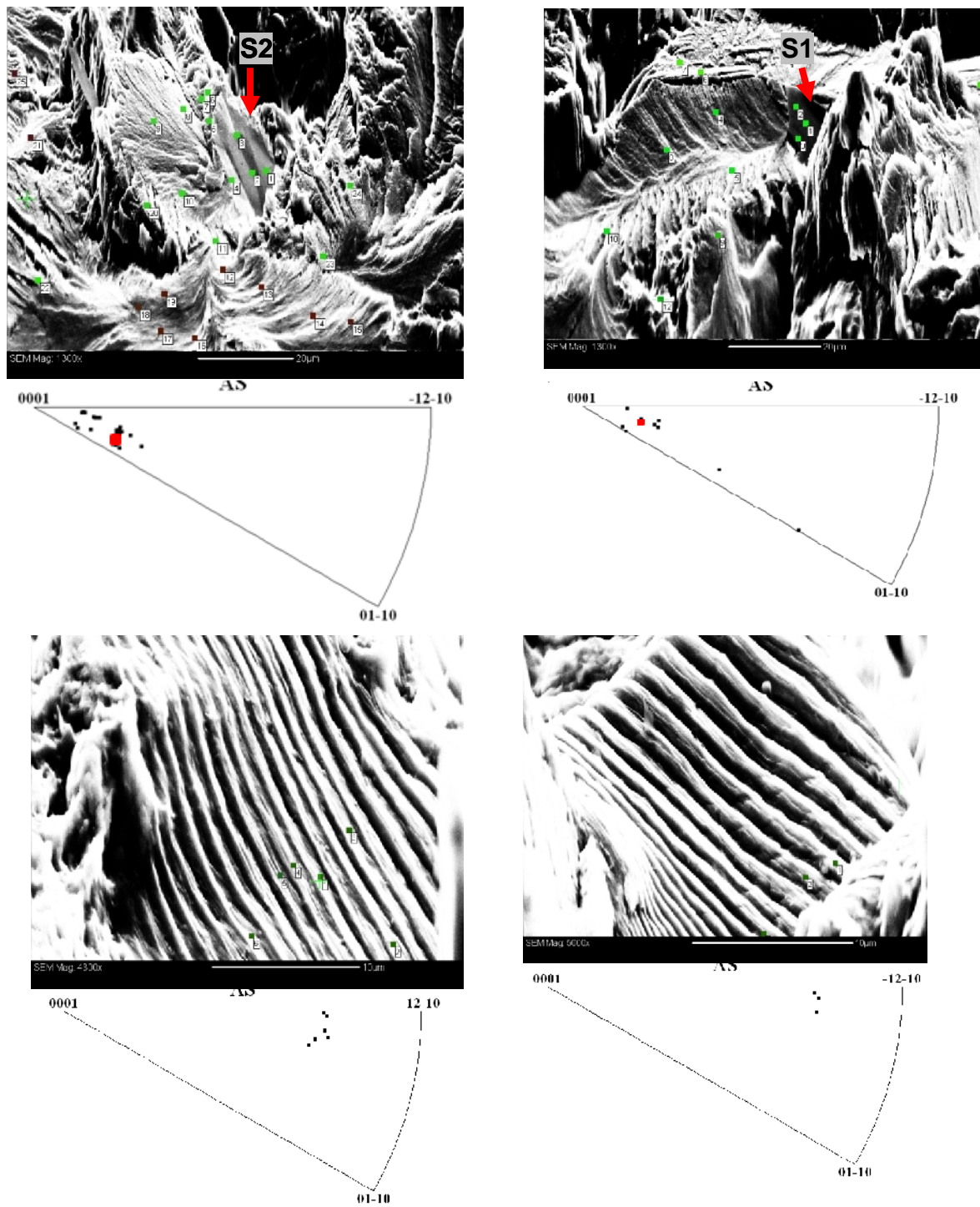
Figure 6.8 Analyses EBSD sur la surface de rupture (mode manuel)
