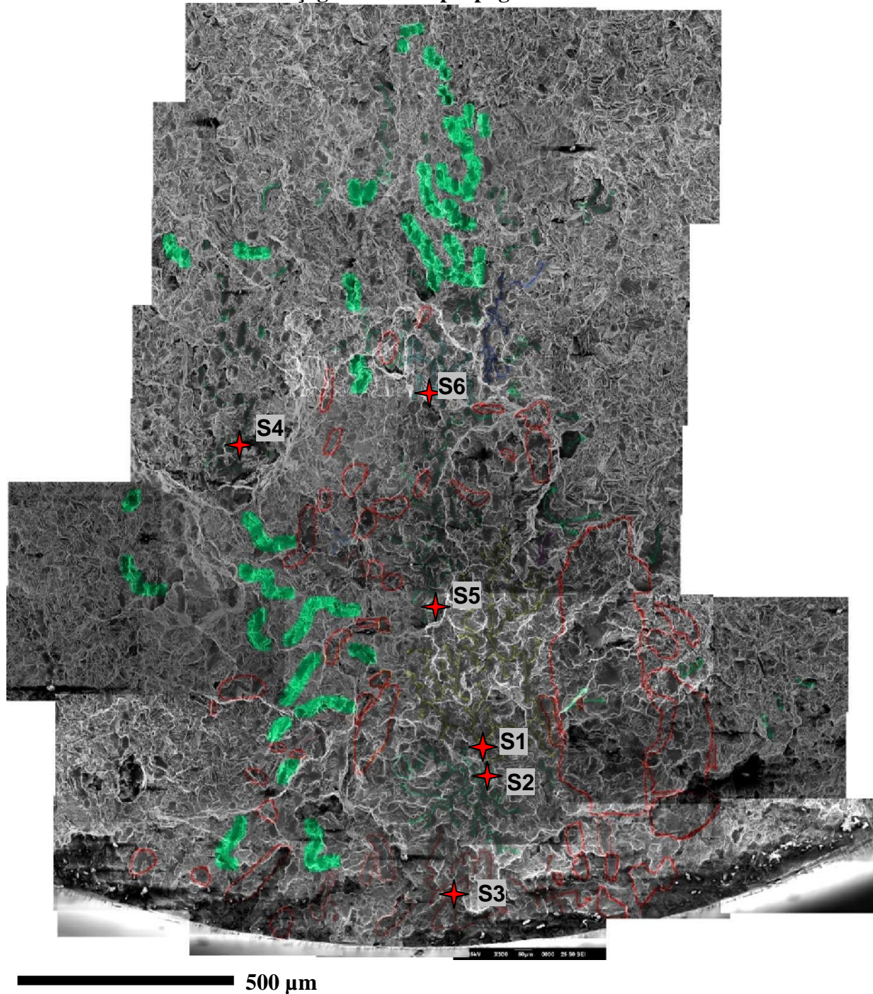
Figure 5.4 Identification des sites d'amorçage S1 : site d'amorçage principal, S2- S6 : sites d'amorçage secondaires ; en vert- des sites de réamorçage lors de la propagation de la fissure ; contour rouge- les stries de fatigue
