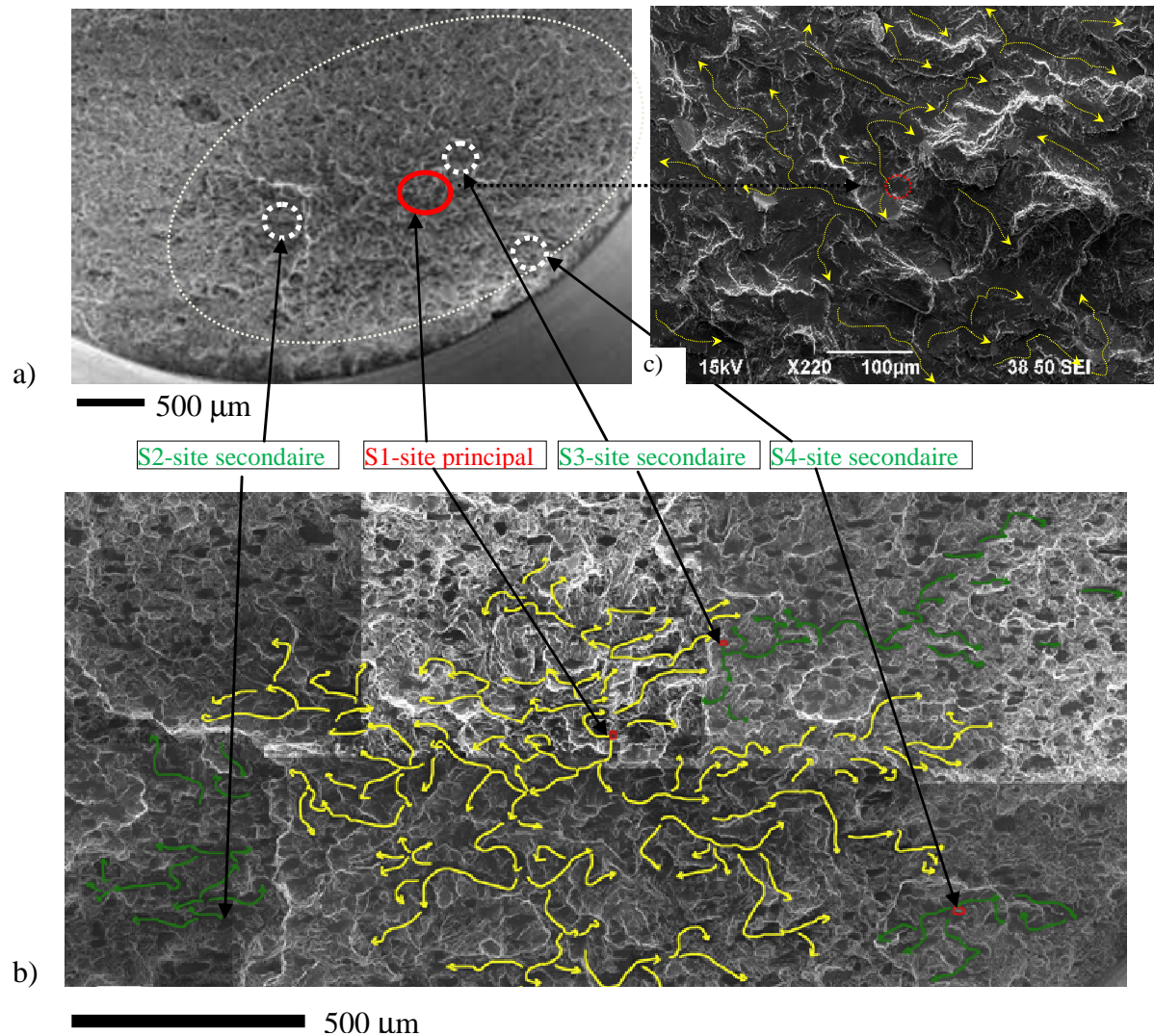
Figure IV.19 Fractographie au MEB de l'Epr 3
