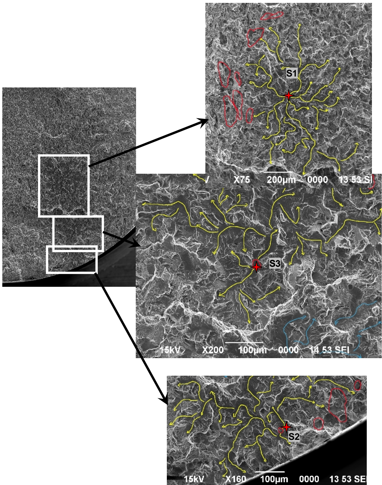
Figure CE130.3 Identification des sites d'amorçage de la région R1 et R3 : S1- site d'amorçage principal, S2 et S3- sites d'amorçage secondaires ; contour rouge- les stries de fatigue
