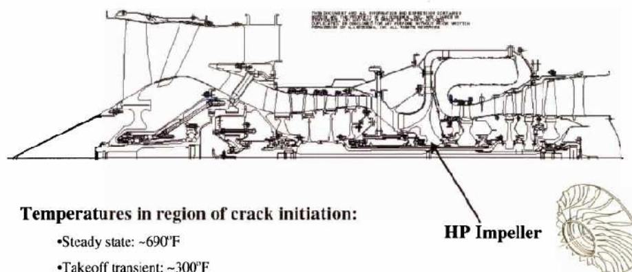
Figure II.1 Pièces critiques fabriquées en alliage de titane (« impeller »)
