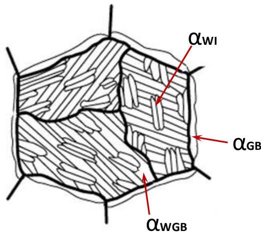
Figure I.2 Représentation schématique d'un ex-grain- \beta transformé [Kobayashi 1988]
