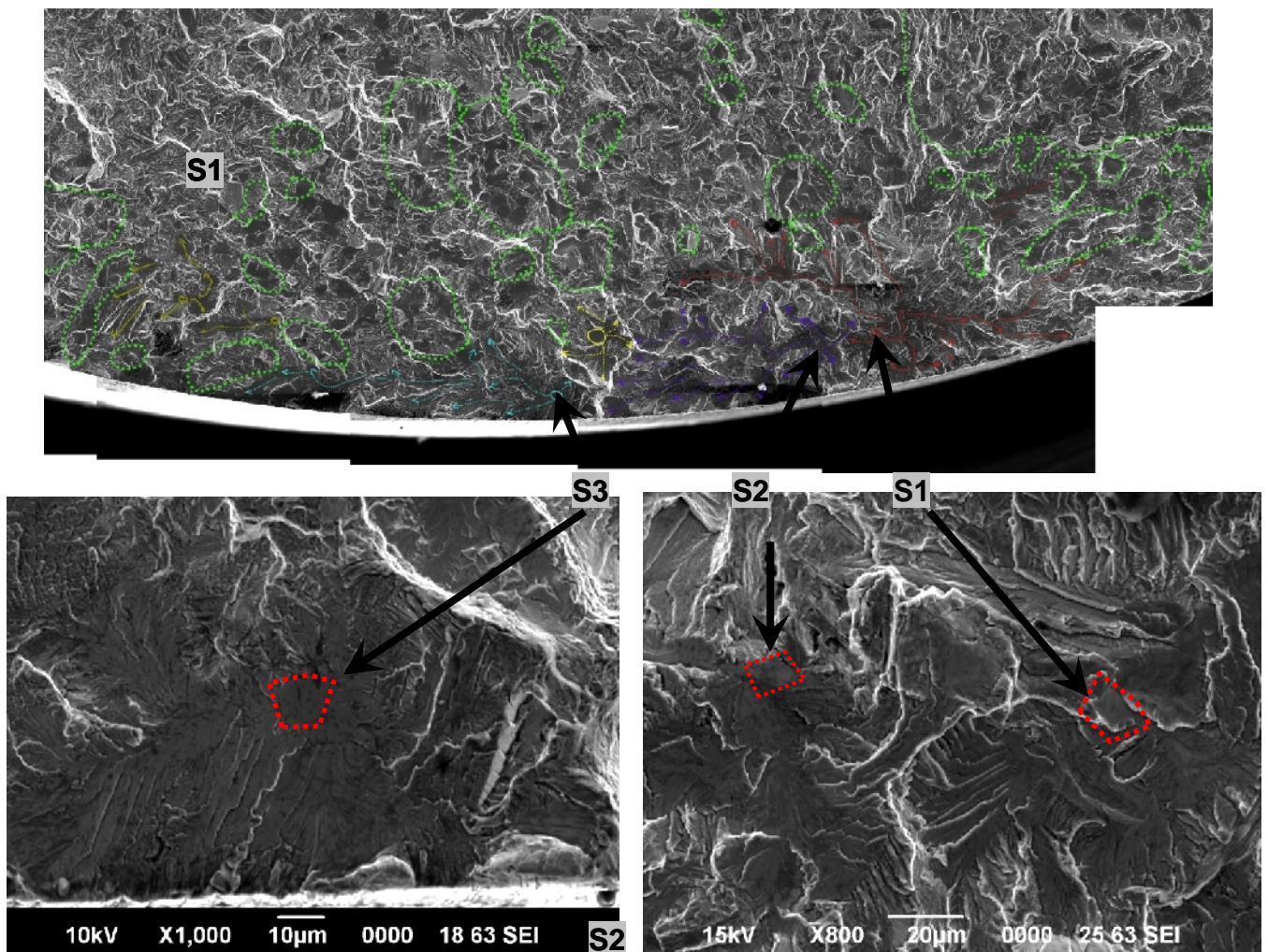
Figure DE260.2 Sites d'amorçage primaire S1 et des sites secondaires S2, S3 délimités par les lignes pointillées rouges
