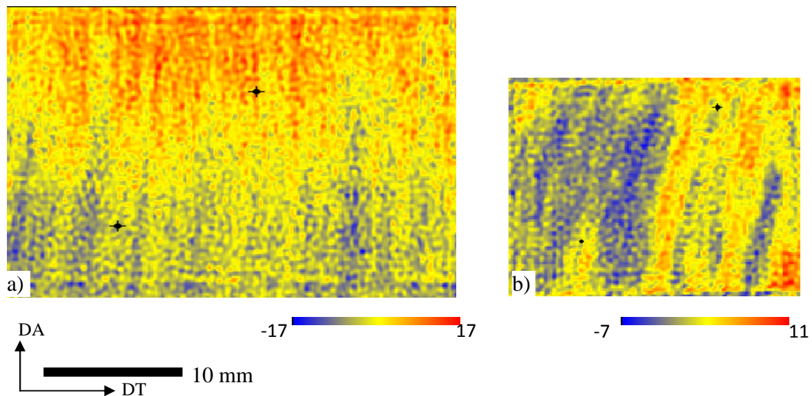
Figure III.8 La variation du signal rétrodiffusé autour de la valeur moyenne pour (a) l'échantillon UA1_HN à 5mm sous la surface d'analyse et (b) UB1_LN à 6 mm sous la surface d'analyse [Toubal 2006, Toubal 2007]
