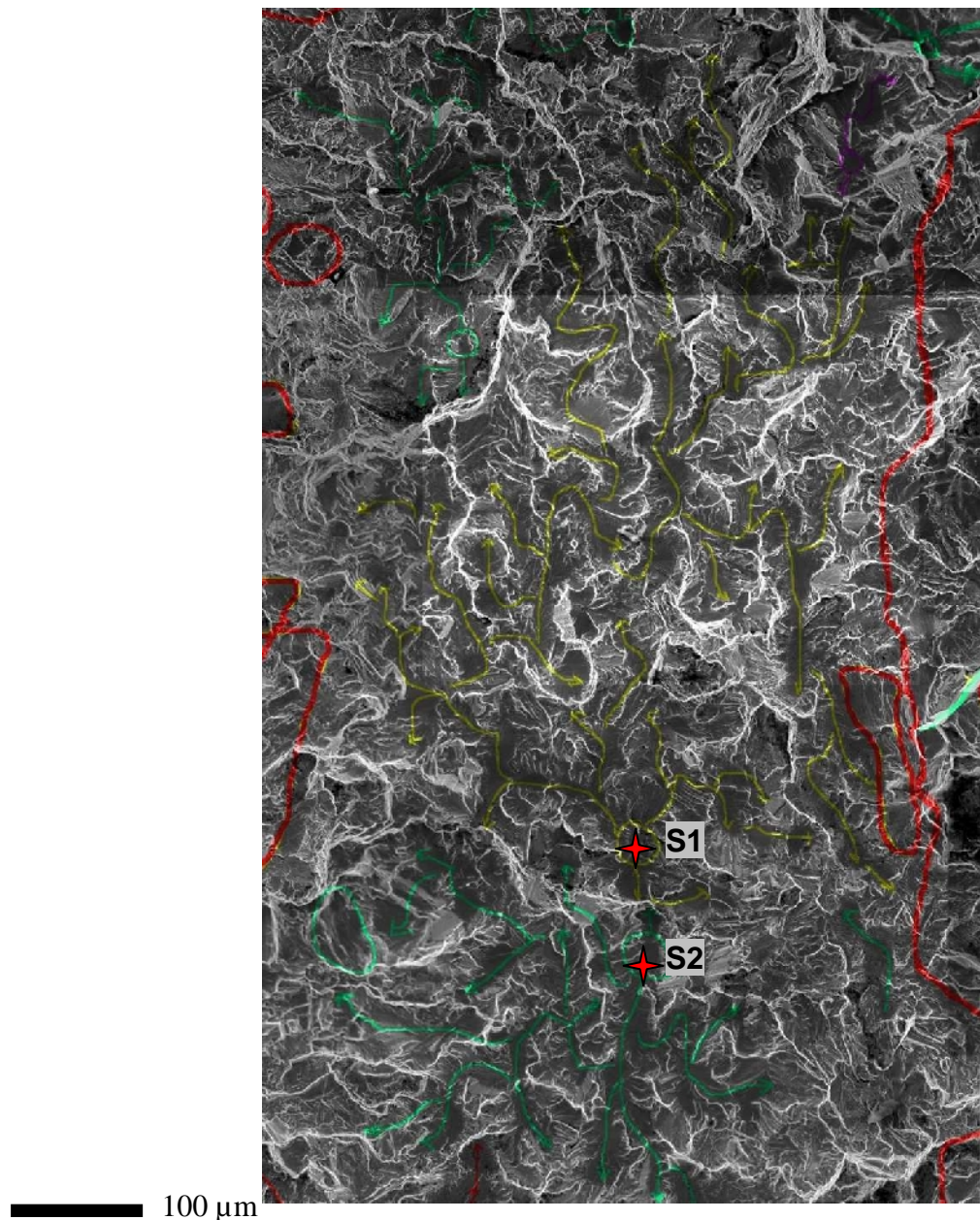
Figure 5.5 Amorçage et propagation de la fissure (site d'amorçage S1 en rouge et propagation par quasi-clivage en jaune, site d'amorçage S2 en rouge et propagation par quasi-clivage en vert). zones à stries entourées par des lignes rouges
