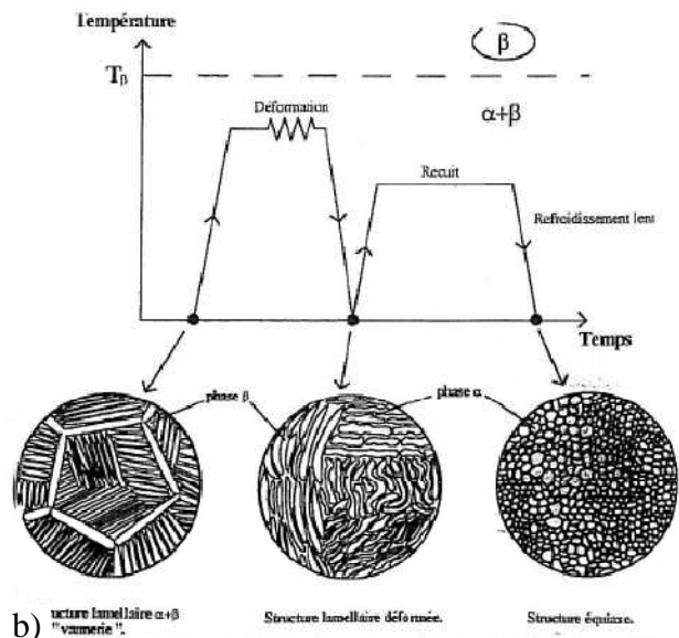
Figure I.4 a) Microstructure équiaxe, alliage Ti6242 [Lütjering 2007] ; b) Schéma d'obtention d'une microstructure équiaxe [Dumanovski 1997]
