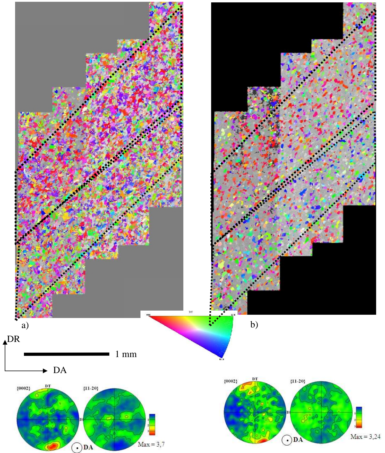
Figure R1.3 Microtexture et texture locale des grains \alpha_S (a) et des grains \alpha_P (b)
