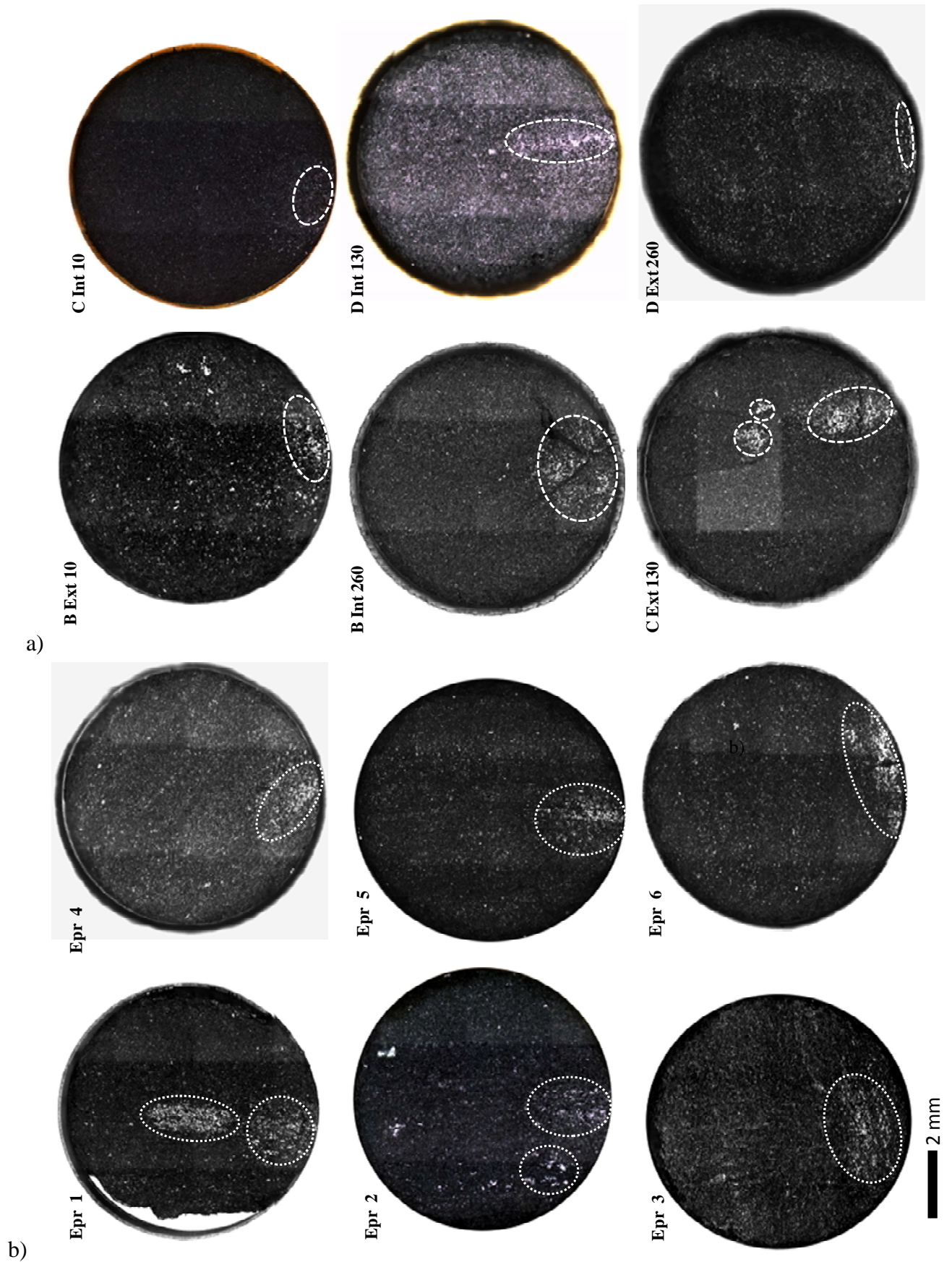
Figure IV.17 Macrographie optique (a) des six éprouvettes en provenance du cylindre central; (b) des six éprouvettes en provenance de la zone morte
