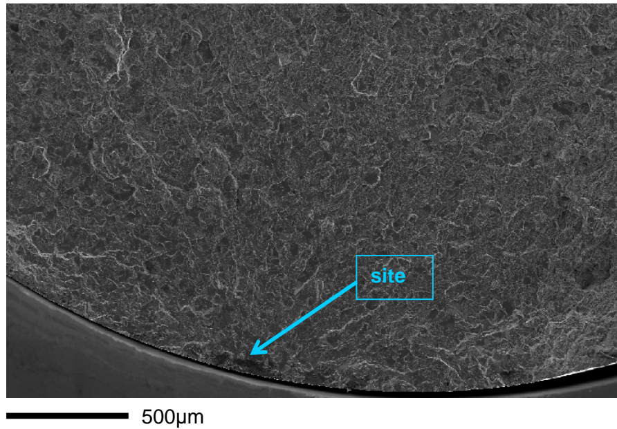
Figure CI10.2 Situation du site d'amorçage sur la zone de clivage
