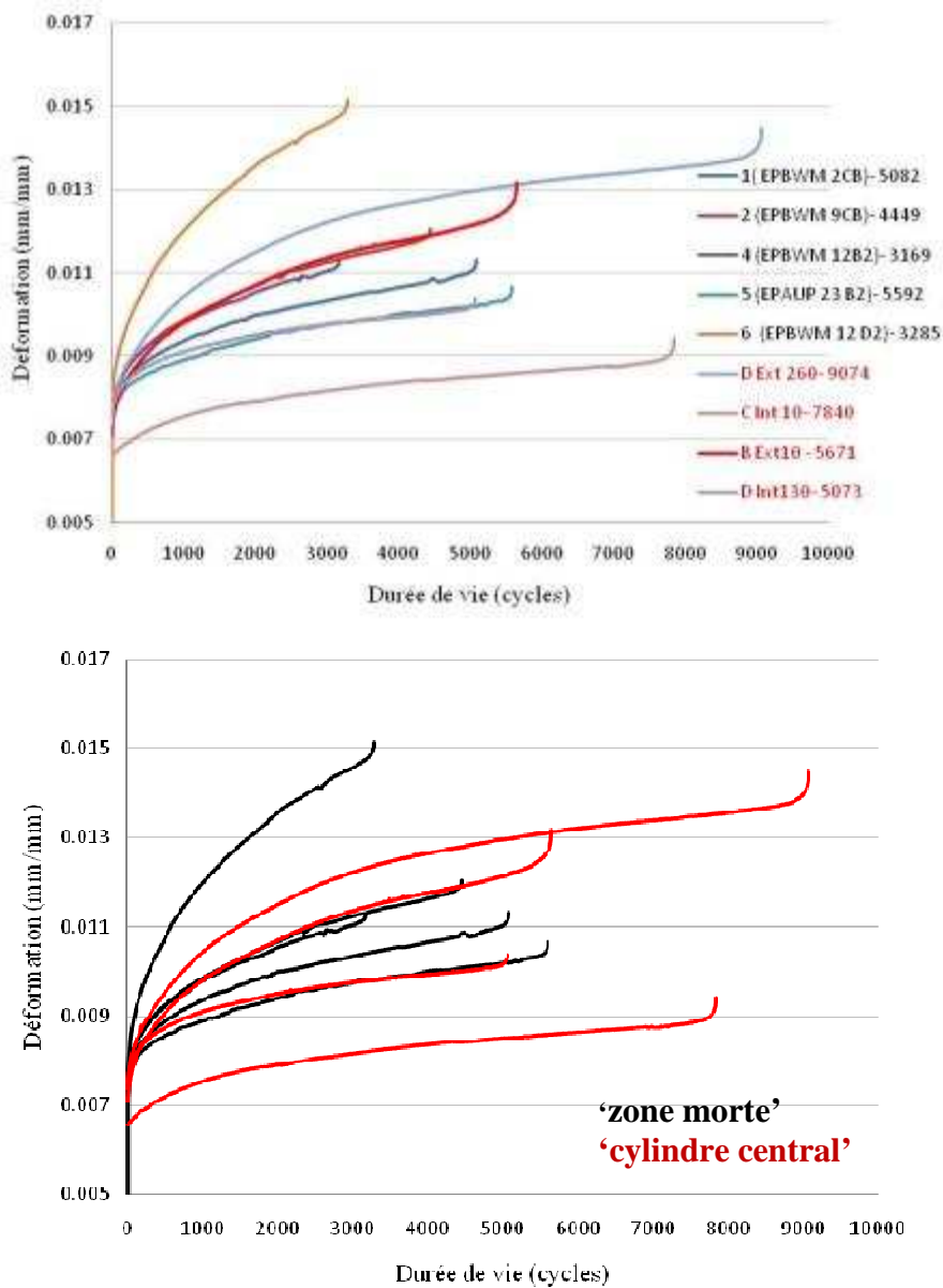
Figure IV.12 Evolution de la déformation en fonction du nombre de cycles en fatigue-fluage ; a) représentation pour chaque échantillon, b) représentation en fonction de la zone de prélèvement des éprouvettes
