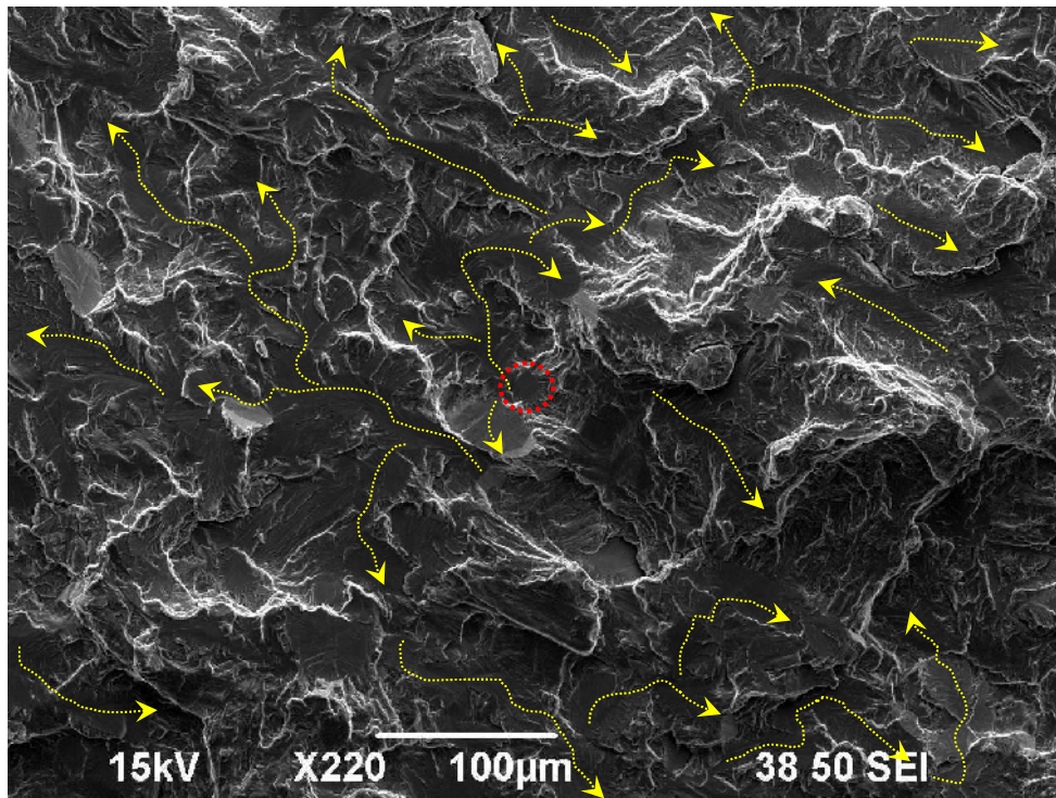
Figure 3.5 Amorçage et propagation de la fissure (site d'amorçage SI en rouge et propagation par quasi-clivage en jaune).
