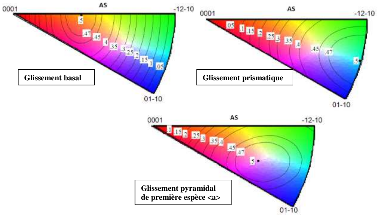
Figure IV.27 Figures de pôles inverses des direction de sollicitations et iso-lignes de facteur de Schmid pour les systèmes de glissement basal, prismatique et pyramidal I <a>
