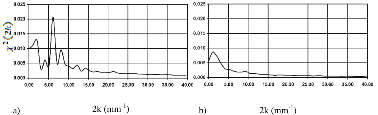
Figure III.7 La variation de la puissance rétrodiffusée \chi^2(2k) en fonction de 2k pour les échantillons A_HN (a) et B_LN (b) [Humbert 2009]
