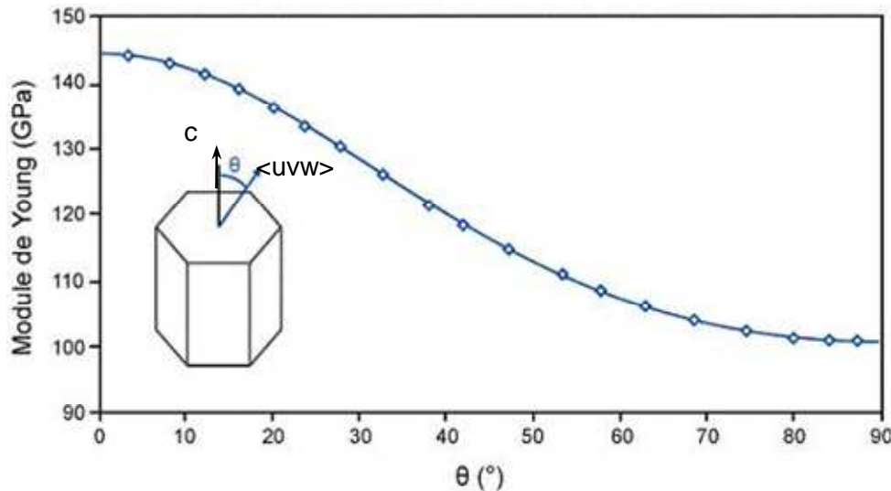
Figure I.1 Valeur du module de Young à température ambiante en fonction de l'orientation du réseau hexagonal vis-à-vis de la direction de sollicitation [Fisher 1964]
