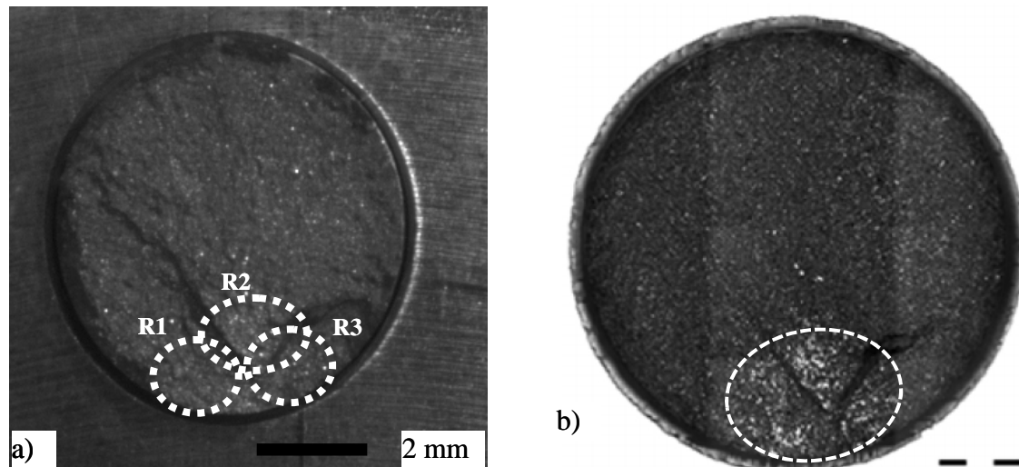
Figure BI260.1 a) Macrographie, b) Micrographie optique
