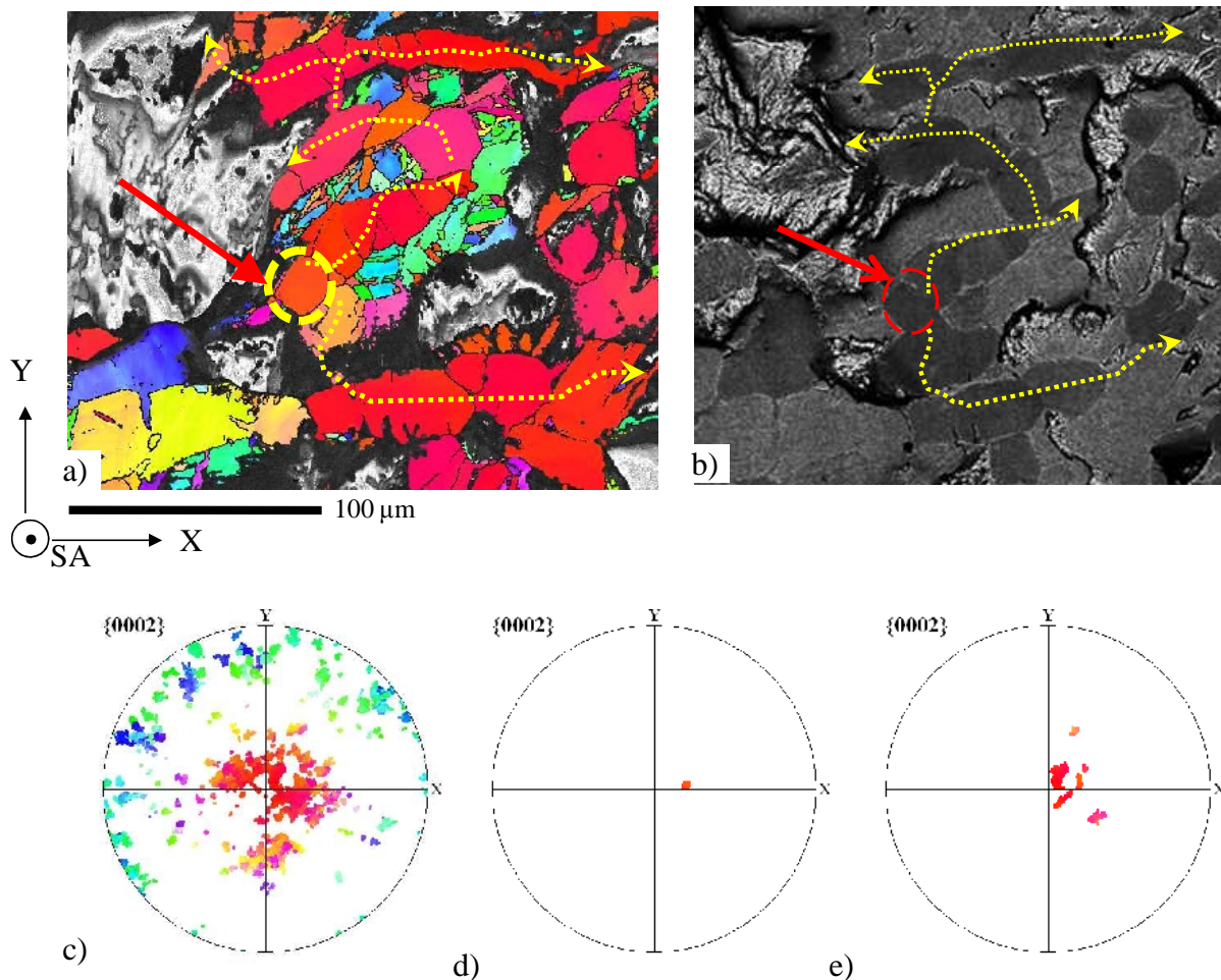
Figure 3.12 a) Cartographie d'orientations au niveau du site principal d'amorçage et des grains permettant la propagation par quasi-clivage ; b) la microstructure au niveau du site principal d'amorçage; c) figure de pôles \{00.2\} de tous les orientations ; d) figure de pôles \{00.2\} du site d'amorçage ; e) figure de pôles \{00.2\} des grains \alpha_P sur le chemin de propagation de la fissure.
