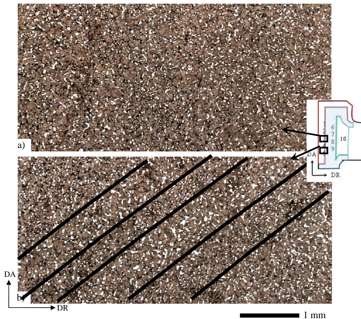
Figure II.14 Distribution et morphologie des grains \alpha_P dans la tranche : a) zone de forte déformation, b) zone de déformation intermédiaire
