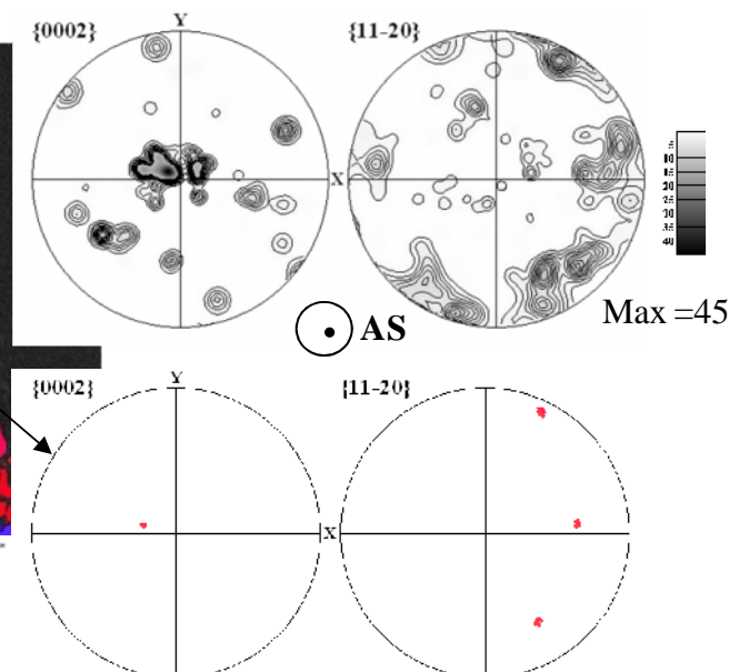
Figure 6.12 Cartographie EBSD dans la région R1, site d'amorçage S2
