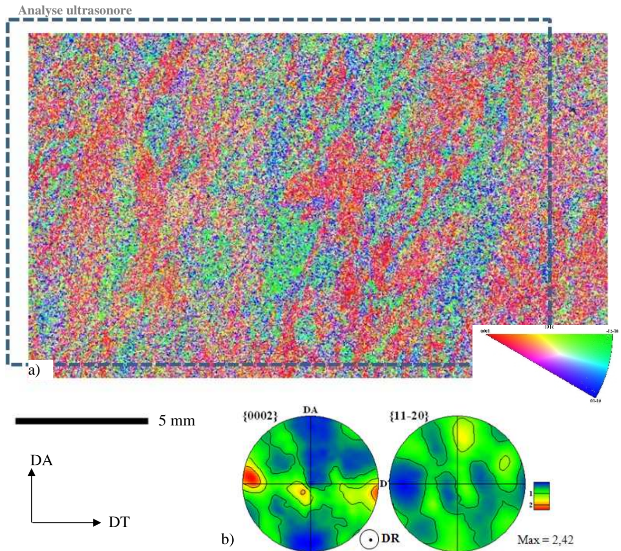
Figure III.10 (a) La cartographie d'orientations et (b) les figures de pôles associées pour l'échantillon UB1_LN
