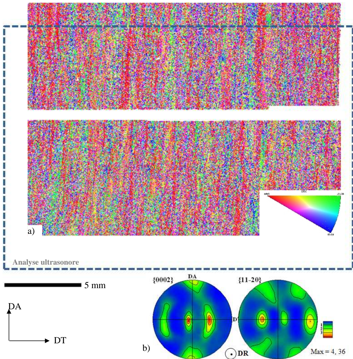
Figure III.9 (a) La cartographie d'orientations et (b) les figures de pôles associées pour l'échantillon UA1_HN
