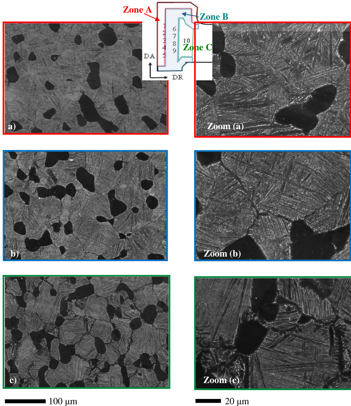
Figure II.13 Microstructures présentes au sein de la tranche
