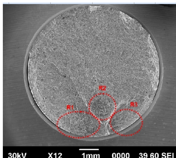
Figure BI260.2: Microscopie électronique de l'éprouvette B Int 260 identifiant les zones brillantes R1, R2, R3
