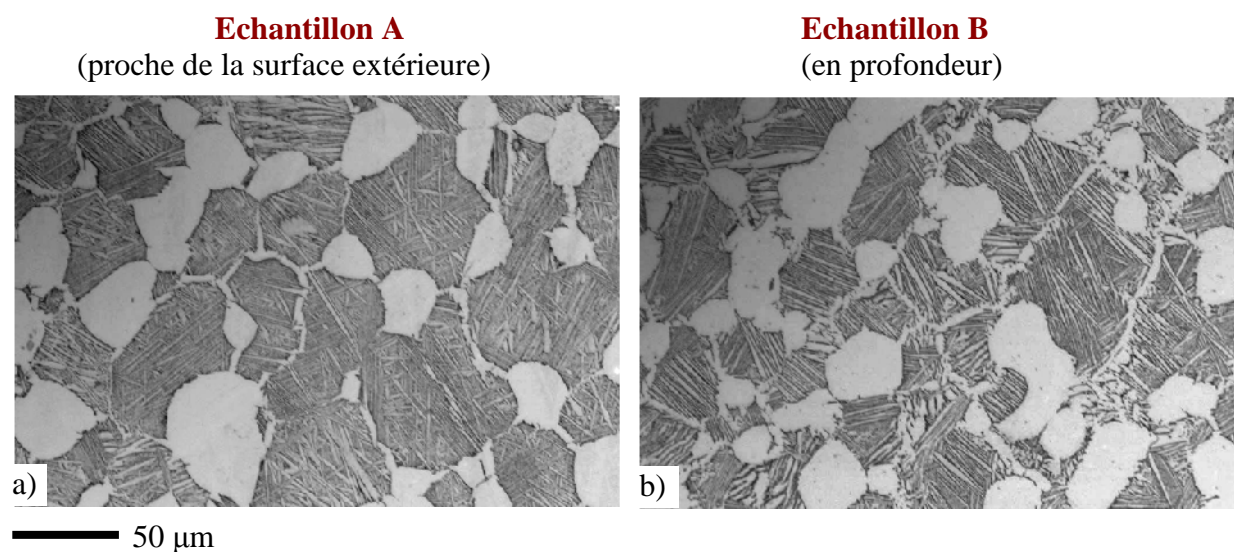
Figure II.8 Microstructure bimodale des deux échantillons A (a) et B (b) ('zone morte', microscopie optique)
