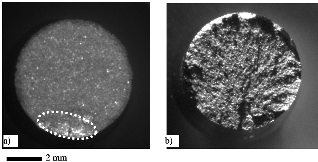
Figure 6.1 a) Macrographie, b) Le relief sur la surface de rupture
