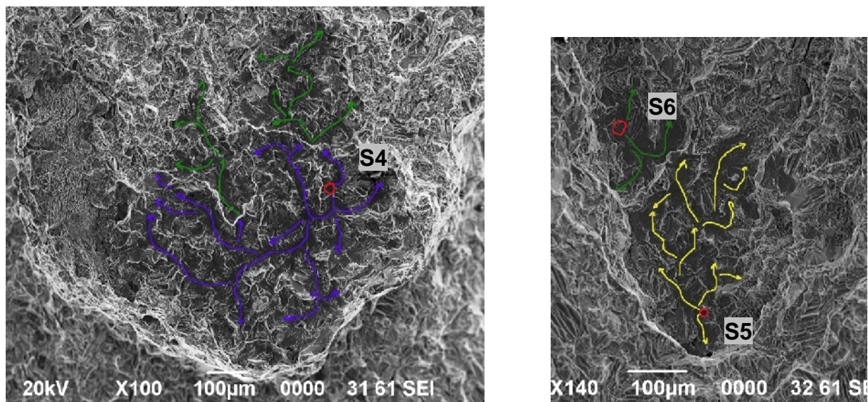
Figure CE130.2 Identification des sites d'amorçage secondaires (S4, S5, S6) des régions R2 et R3
