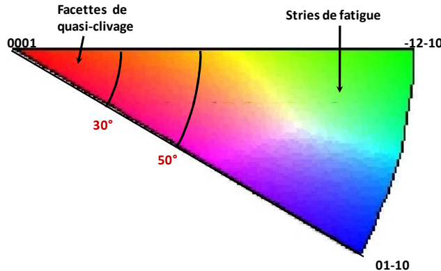
Figure IV.26 Triangle standard montrant les domaines dans lesquels la direction de sollicitation favorise le quasi-clivage et les stries de fatigue
