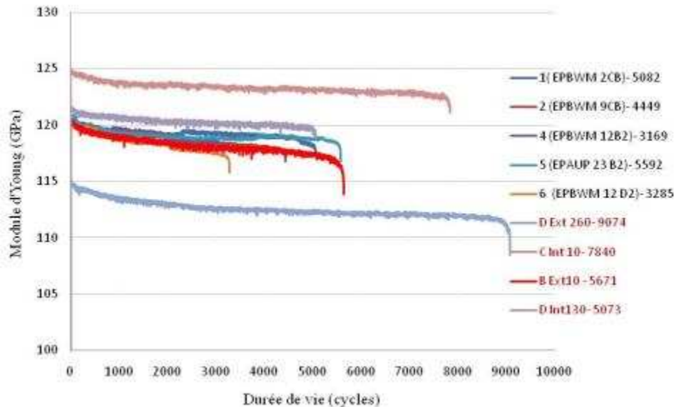
Figure IV.13 Evolution du module d'Young en fonction du nombre de cycles
