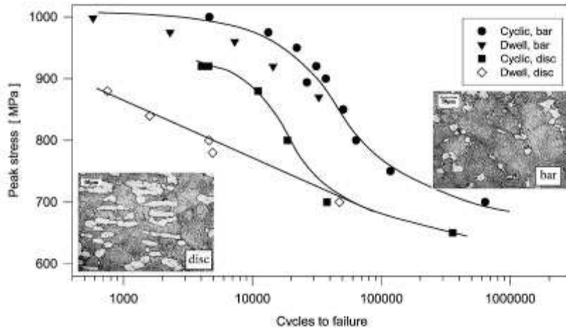
Figure I.12 Tests de fatigue d'un IMI 834 [Bache 1997]
