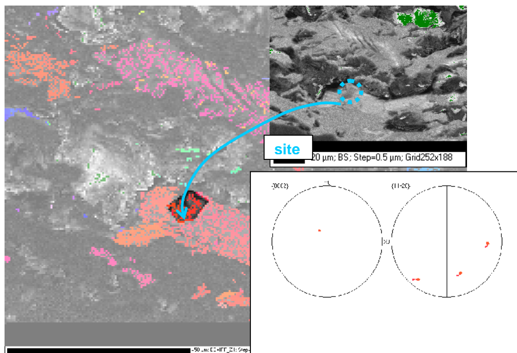
Figure CI10.5 Cartographie automatique sur le site d'amorçage de la fissure
