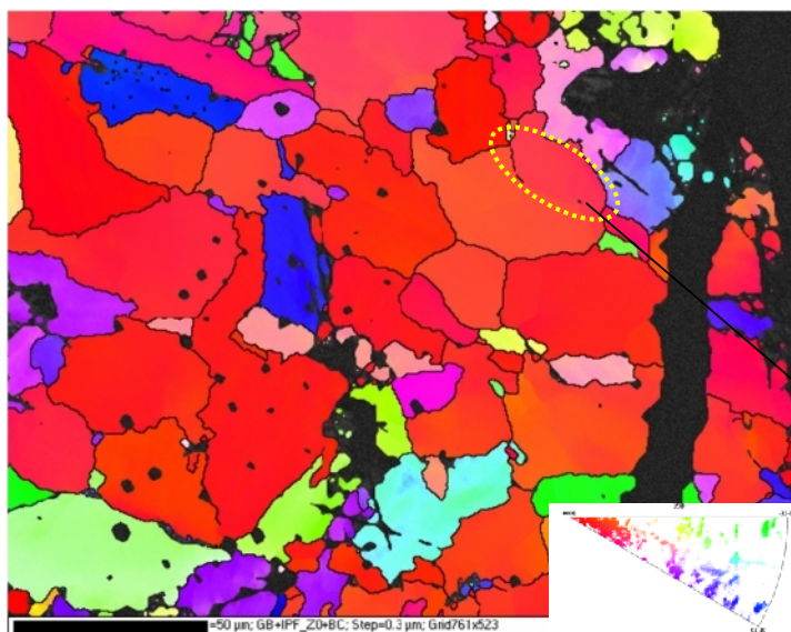
Figure 6.12 Cartographie EBSD dans la région R1, site d'amorçage S2
