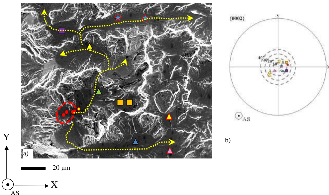
Figure IV.20 Indexation en mode manuel du site principal d'amorçage et des grains permettant la propagation par quasi-clivage : a) localisation des mesures EBSD, b) figure de pôles \{00.2\}
