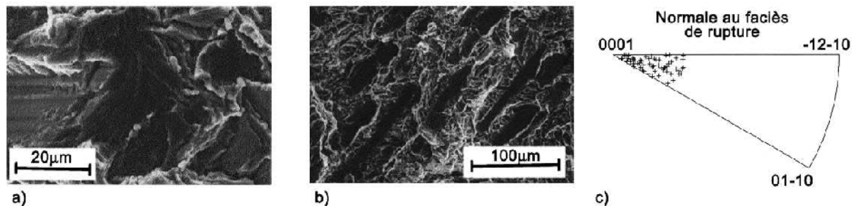
Figure I.13 Observation des faciès de rupture: a) dans la barre, b) dans le disque c) projection de l'orientation des grains clivés sous forme de figure de pôles inverse [Bache 1997]
