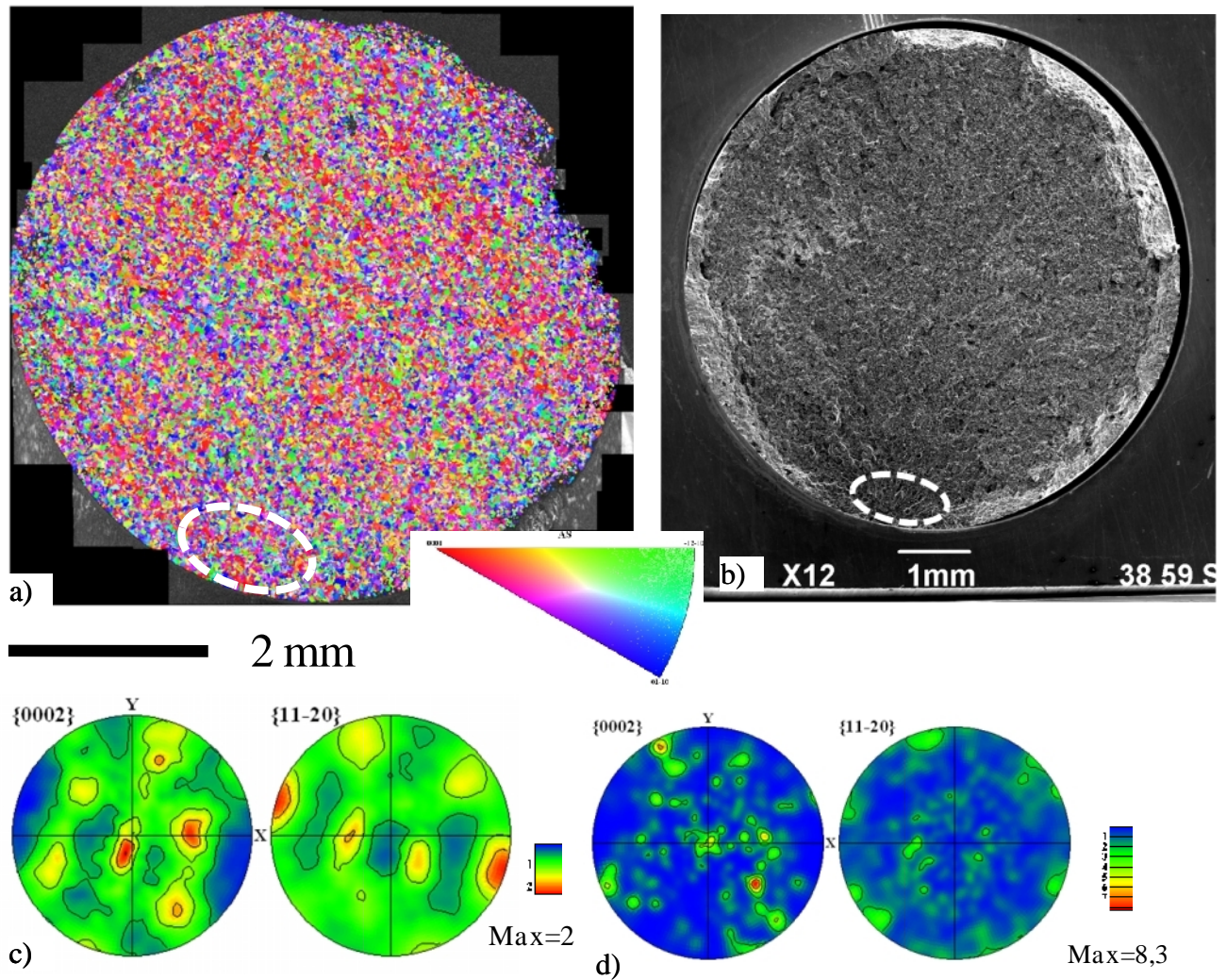
Figure CI10.17 Cartographie EBSD de la section transverse
