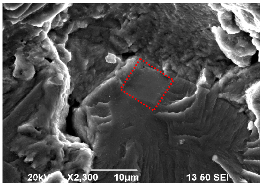
Figure 1.6 Amorçage et propagation de la fissure (site d'amorçage S1 en rouge et propagation par quasi-clivage en jaune)
