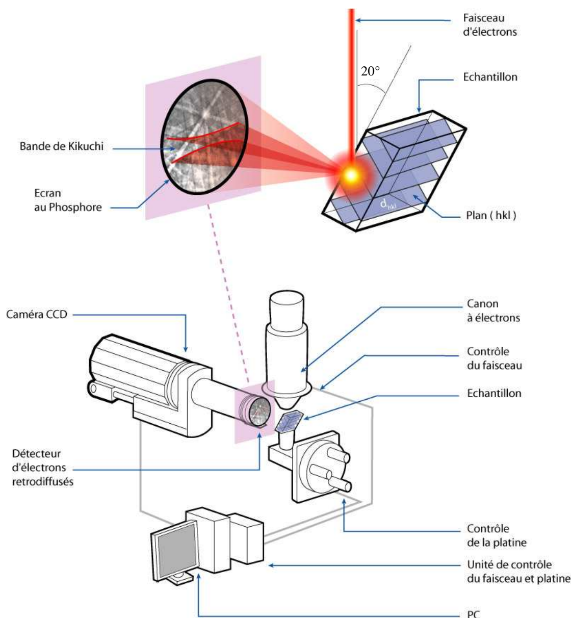
Figure M2.1 Principe de l'EBSD
