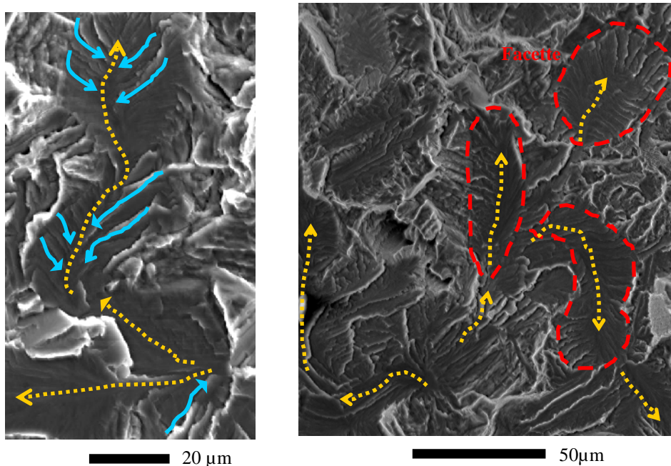
Figure IV.14 Analyse des facettes de quasi-clivage pour identifier le sens de propagation de la fissure
