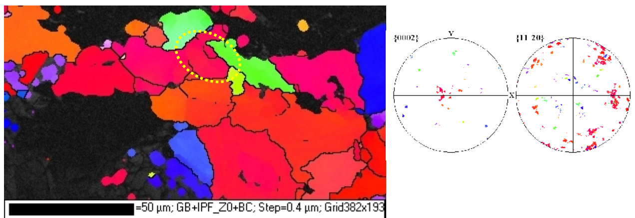
Figure 6.11-1 Cartographie EBSD dans la région R2, site d'amorçage S4
