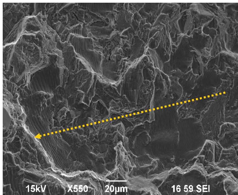
Figure CI10.11 Stries en propagation de la fissure (flèche : sens de la propagation)
