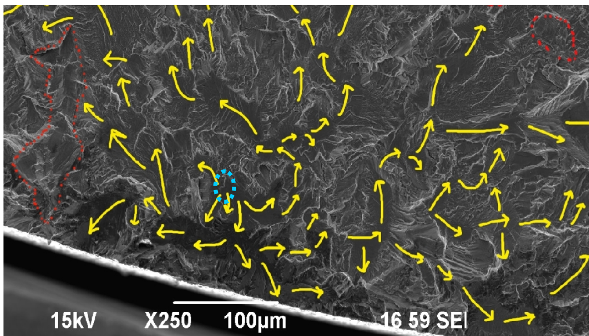
Figure CI10.3 Amorçage et propagation de la fissure (site d'amorçage en bleu et propagation du clivage en jaune).
