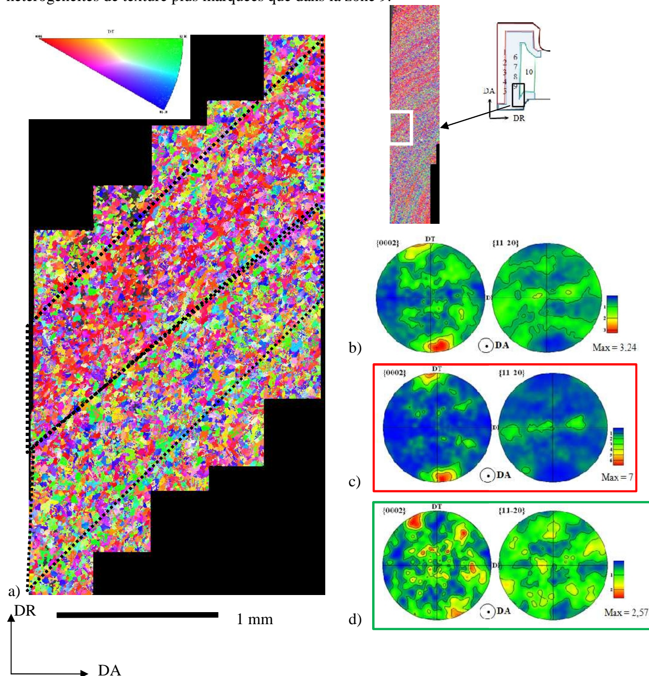
Figure R1.1 Représentation de la texture dans la zone A:
