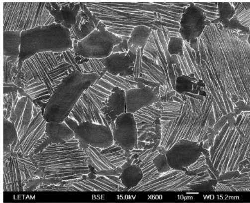
Figure CE130.5 Microstructure de la zone polie, 100 \mu\text{m} sous le site principal S1
