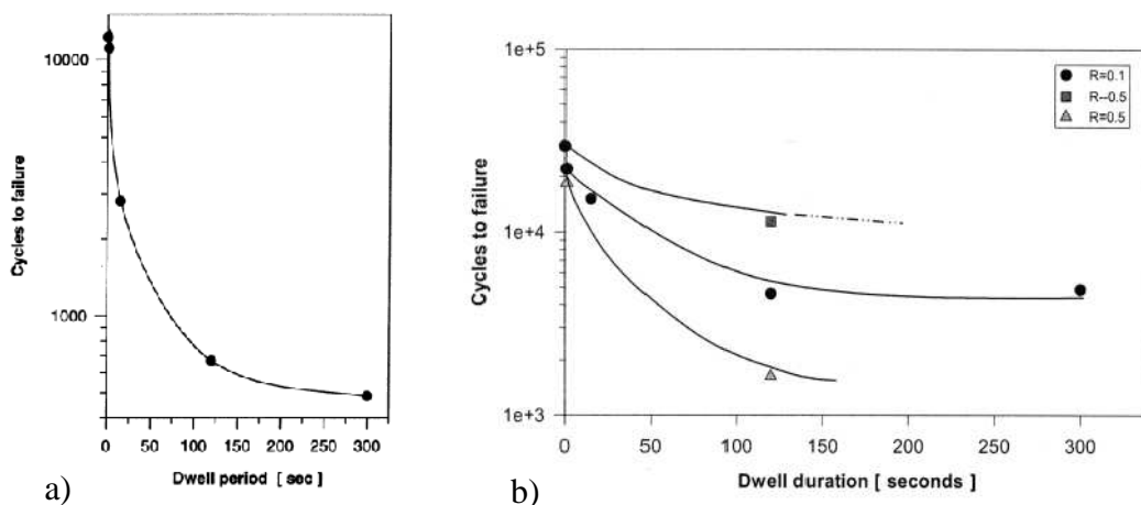
Figure I.10 Influence du temps de maintien de la charge lors d'un essai de fatigue-dwell; a) de 880 MPa sur l'alliage IMI 834 [Bache 1997] b) influence du rapport de charge R [Evans 2006]
