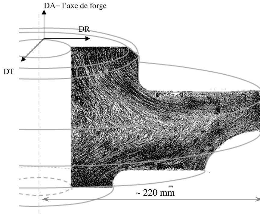
Figure II.12 La macrographie de la tranche après «blue etching» (post-traitement de l'image)
