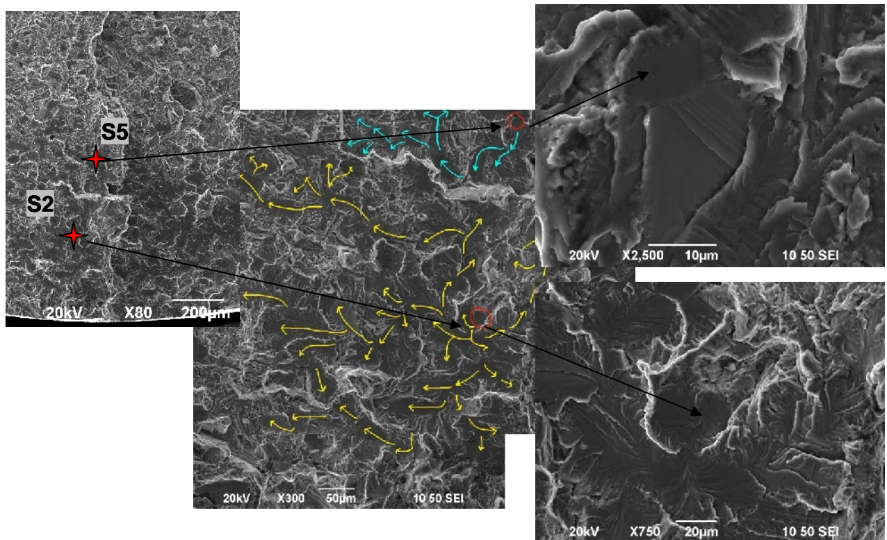
Figure 6.5 Région R1- sites d'amorçage secondaires S2 et S5 ; la propagation par quasi-clivage est marquée par les flèches jaunes
