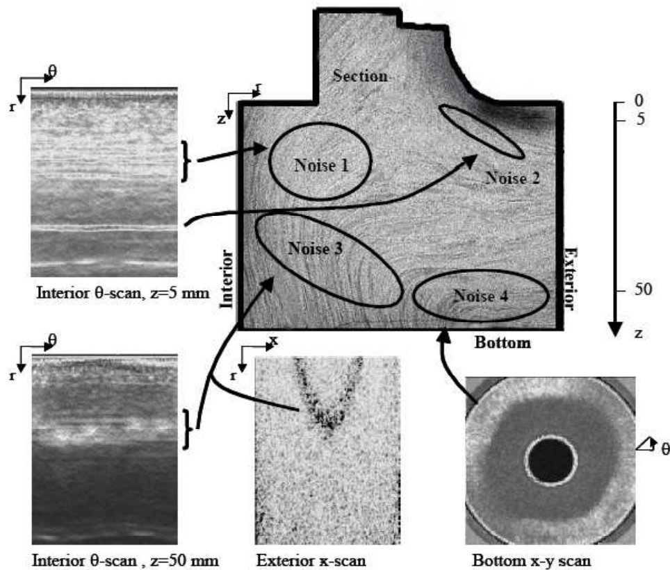
Figure I.19 Localisation des sources du signal rétrodiffusé [Bescond 2004]
