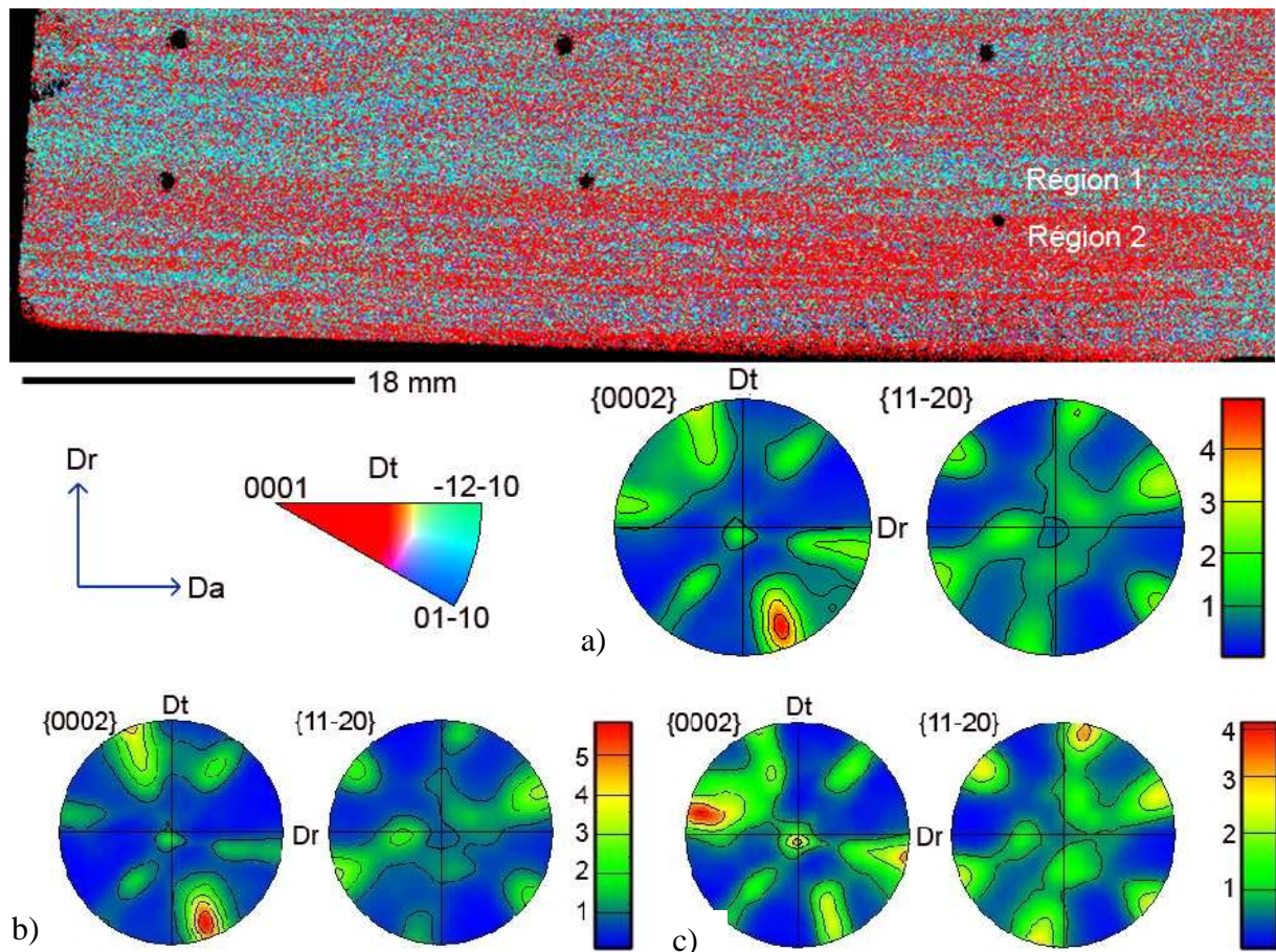
Fig. I.17 Cartographie EBSD montrant la présence de macrozones au sein d'une billette IMI 834 [Germain-2005b]
