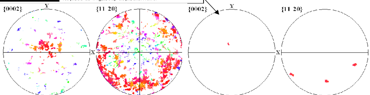
Figure 6.14 Cartographie EBSD dans la région R3, site d'amorçage S3
