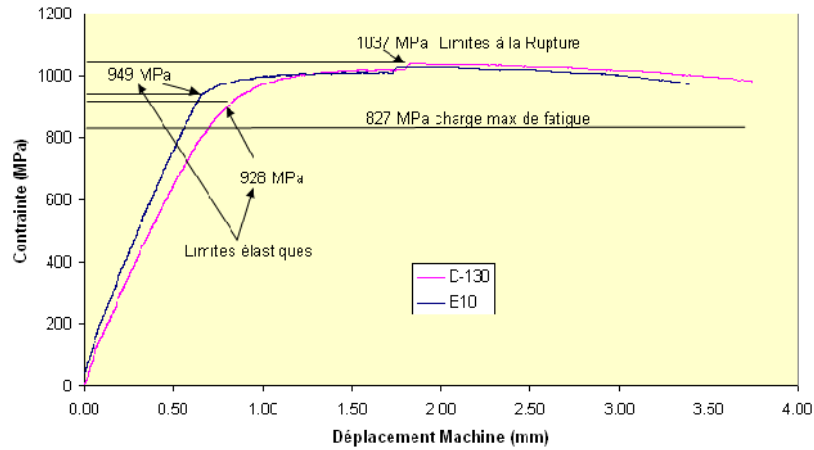
Figure IV.10 Courbes de traction sur deux éprouvettes prélevées dans le cylindre central (l'axe de sollicitation est parallèle à la direction tangentielle du disque)
