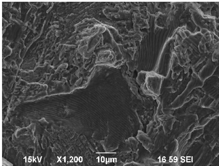
Figure CI10.10 Exemple d'une zone à stries
