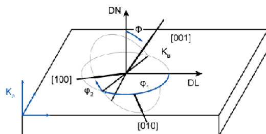
Figure M1.2 Définitions des angles d'Euler
