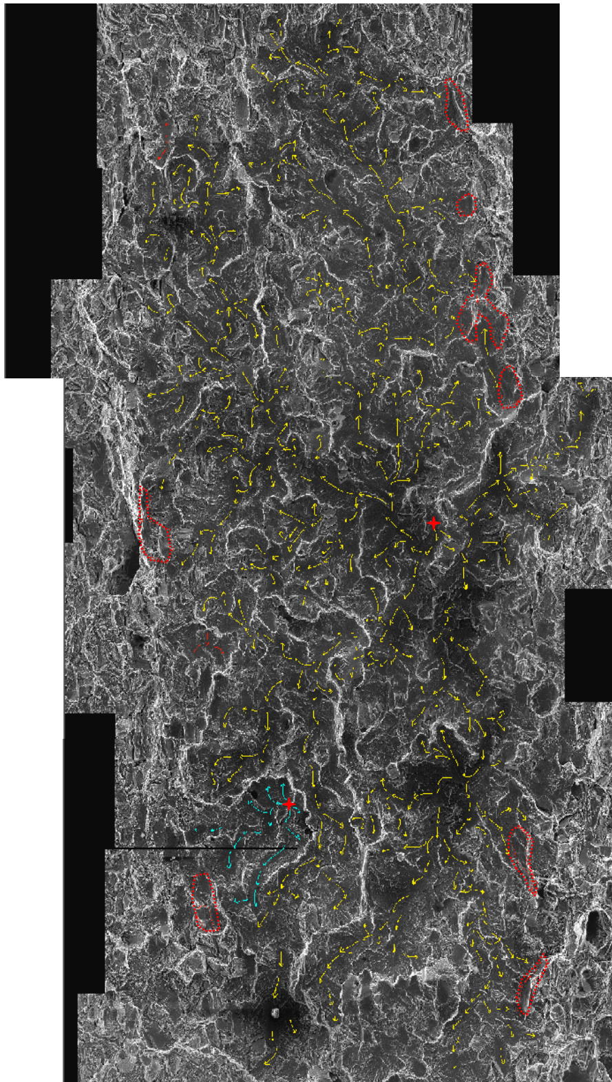
Figure 1.5 Ensemble de la zone brillante en identifiant l'amorçage, la propagation de la fissure par du quasi-clivage et par des stries
