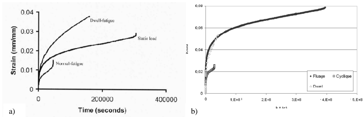
Figure I.9 Déformation accumulée pendant a) un essai de fatigue, 2 min fatigue-dwell et fluage à froid pour alliage Ti-6242 bimodal ( \sigma_{max} = \sim 0,95 \sigma_y ) [Sinha 2004] ; b) un essai de fatigue, 80s fatigue-dwell et fluage à froid pour alliage Ti-6242 lamellaire ( \sigma_{max} = 1,05 \sigma_y ) [Lefranc 2008]
