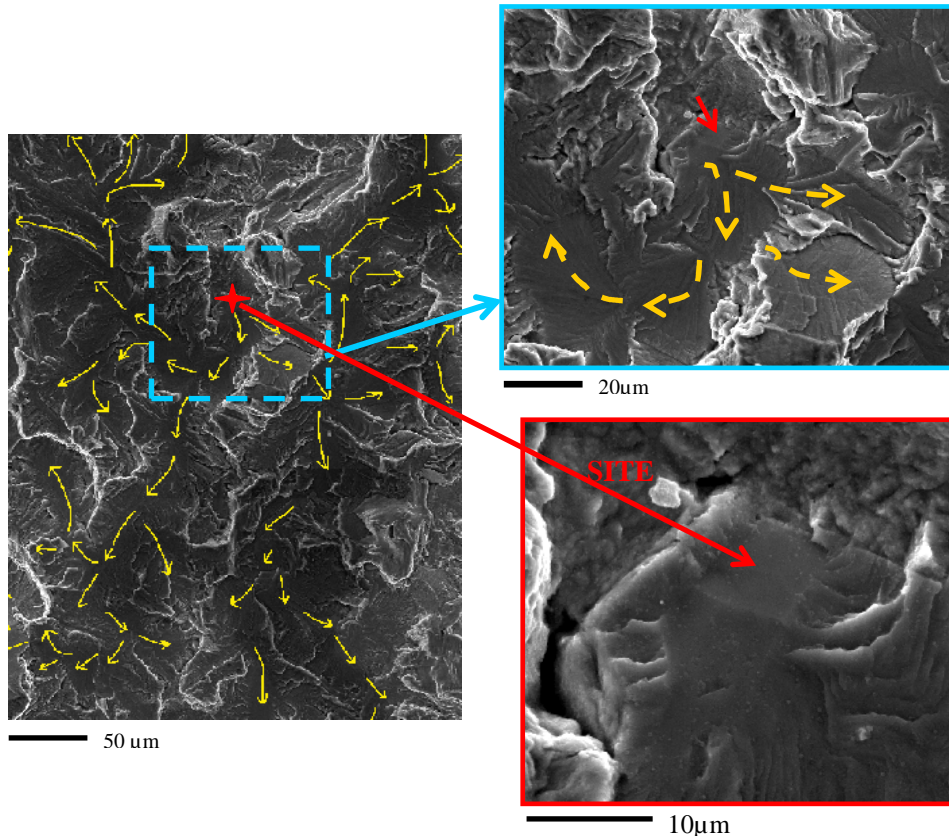
Figure IV.15 Identification du site d'amorçage de la fissure
