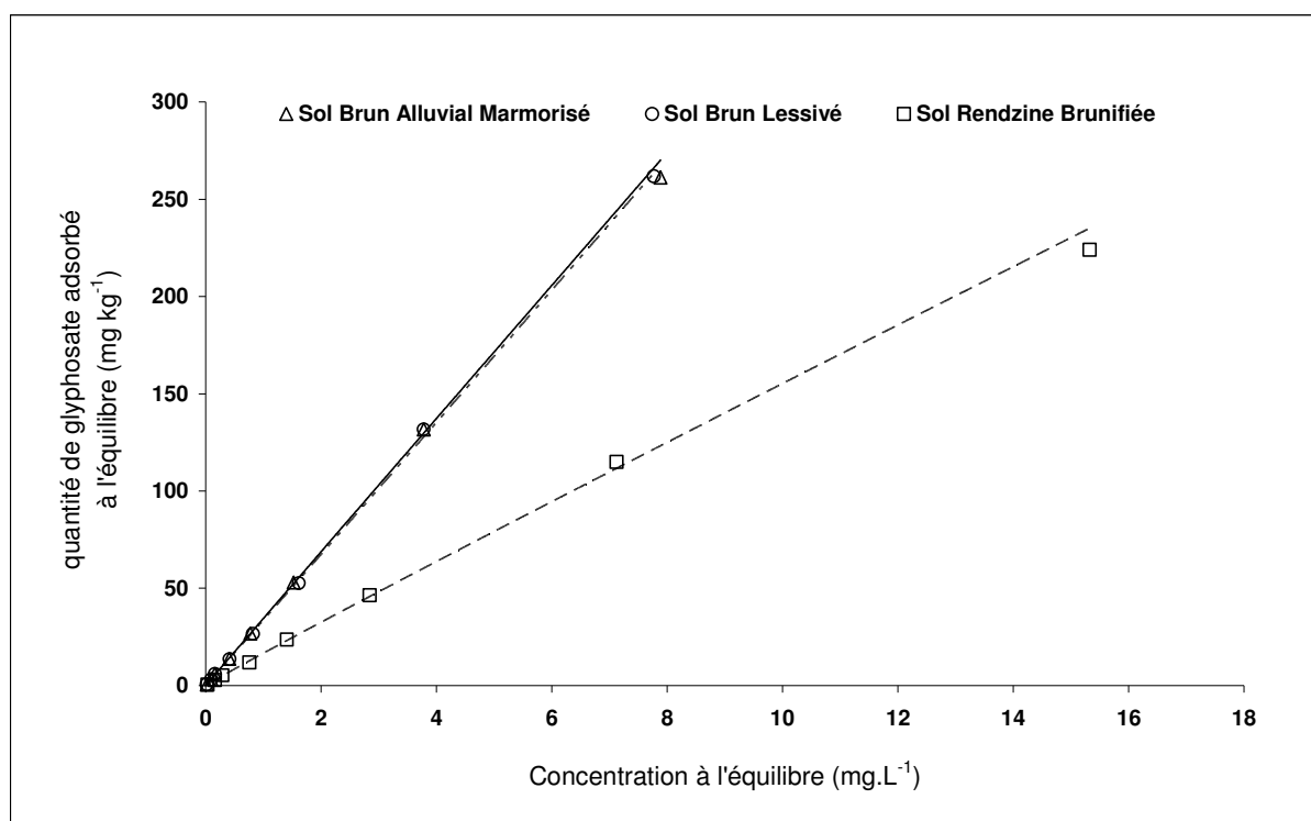
Figure 2. 1. Isothermes d'adsorption du glyphosate obtenues avec les 3 sols étudiés : sol brun lessivé, rendzine brunifiée et sol brun alluvial marmorisé (symboles : valeurs expérimentales ; Courbes : modèle de Freundlich). Ecart-type présents mais inférieurs à la taille des symboles.
