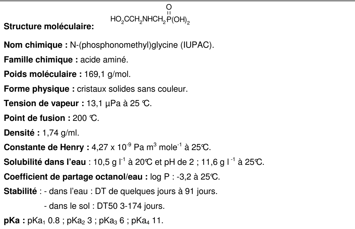
Figure 1.1. Principales caractéristiques physico-chimiques du glyphosate (Worthing et Hance. 2000 ; Agritox, 2007 ; Couture et al. , 1995).
