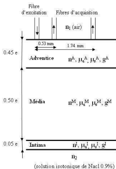
FIG. 4.7 – Représentation schématique du modèle tri-couche utilisé pour simuler le transport de la lumière dans le tissu artériel. e représente l'épaisseur totale de l'artère, n^i, \mu_a^i, \mu_s^i, g^i correspondent respectivement à l'indice de réfraction, aux coefficients d'absorption et de diffusion et au facteur d'anisotropie pour l'adventice ( i = A ), la média ( i = M ) et l'intima ( i = I ). n_1 et n_2 sont les indices de réfraction des milieux environnants, c'est-à-dire l'air ( n_1 = 1 ) la solution isotonique de NaCl ( n_2 = 1,33 ). Les mesures des épaisseurs e des trois couches artérielles sont déterminées à partir des coupes histologiques et des images réalisées.
